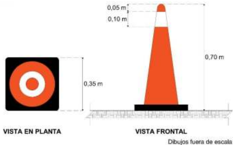
Figura V.6-5 Cono
