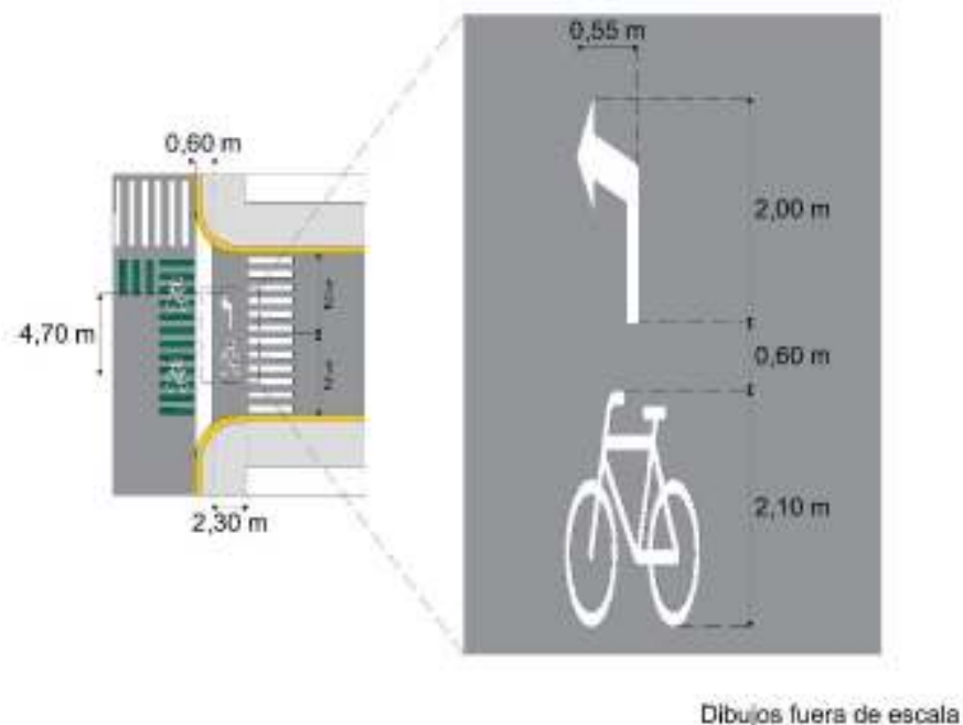
Figura VII.2- 14 Pictogramas y flecha para señalar el área de espera ciclista avanzada
