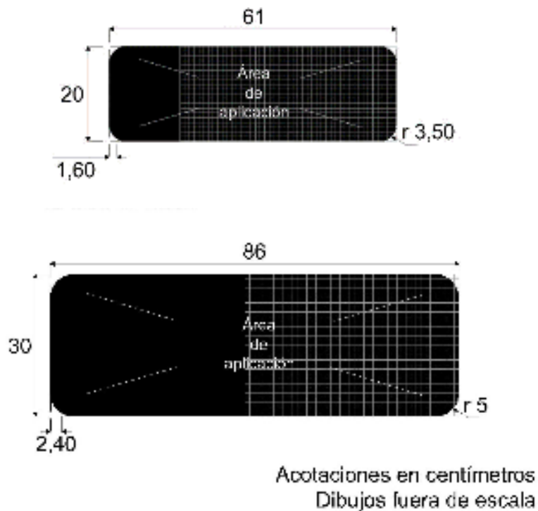
Figura III.3-7 Área de aplicación para la señal SR-37 Sentido de circulación
