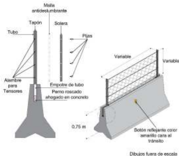
Figura IV.11- 1 Detalle de malla antideslumbrante
