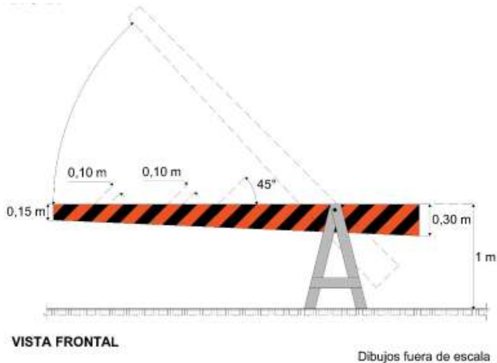
Figura V.6-1 Barrera levadiza
