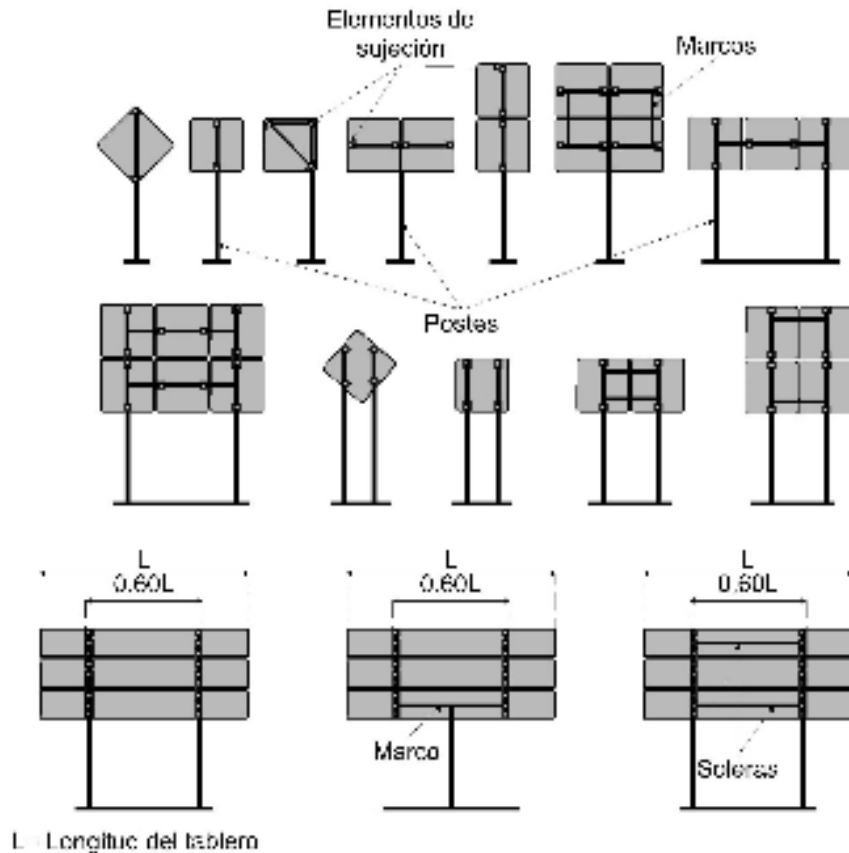
L = Longitud del tablero Fuente: "Capítulo N-CMT-5-02 002 Láminas y Estructuras para Señalamiento Vertical, de la Normativa para la Infraestructura del Transporte, de la Secretaría de Infraestructura, Comunicaciones y Transportes".
