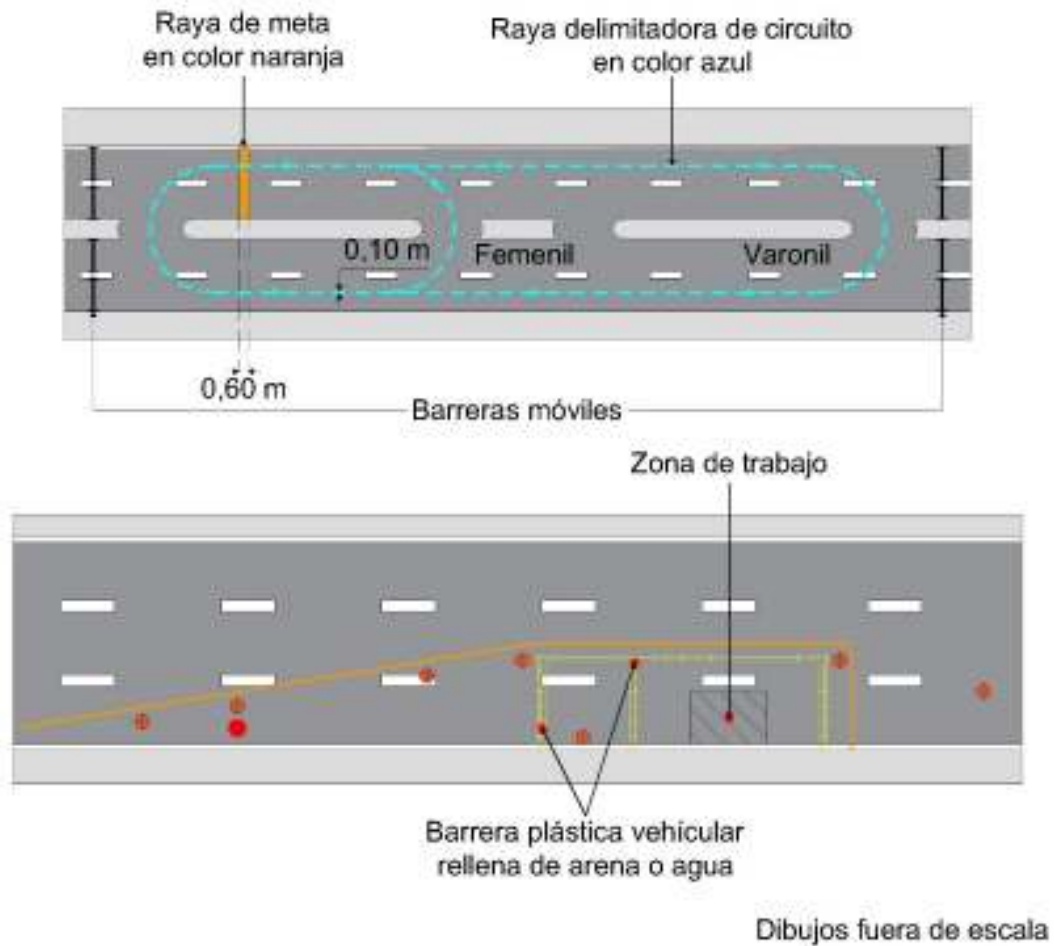
Figura II.2- 52 Marcas temporales
