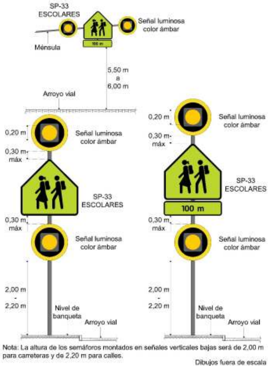
Figura VI.5- 19 Semáforo en zonas escolares
