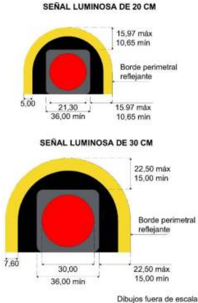
Figura VI.5-34 Pantalla antirreflejante del semáforo
