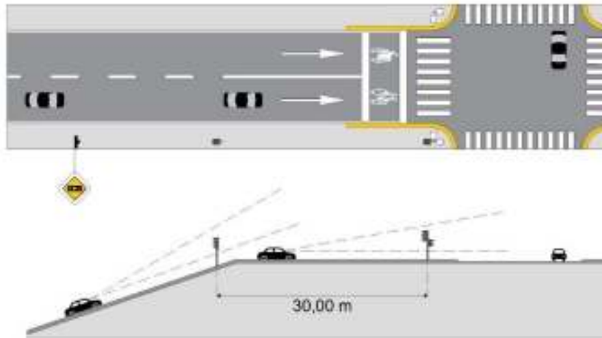
Figura VI.5-11 Ubicación de semáforos en pendientes
