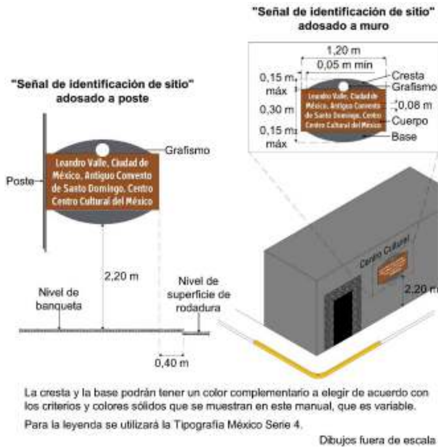
Figura VII.1- 17 Señal para identificar sitio de interés
