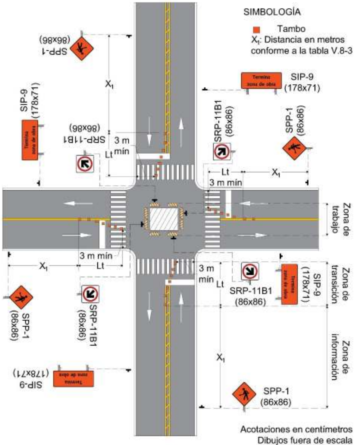
Figura V.10-16 Cierres de carriles en el centro de una intersección (Vía con ancho de arroyo vial menor a 9 m)
