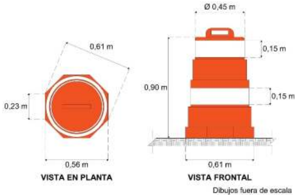
Figura V.6-6 Tambo
