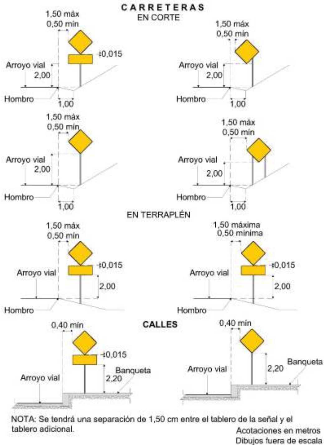
Figura III.2-3 Distancia lateral y altura de las señales preventivas
