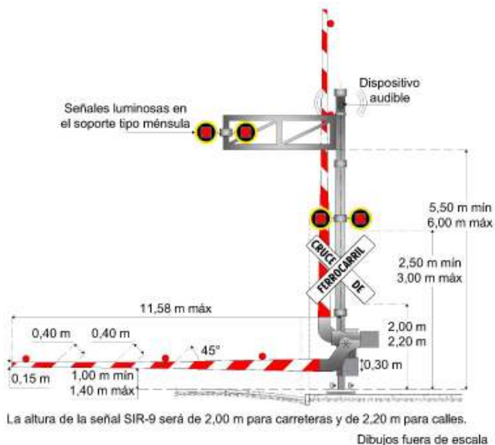
Figura VI.6- 2 Señal audible para cruce de vía férrea
