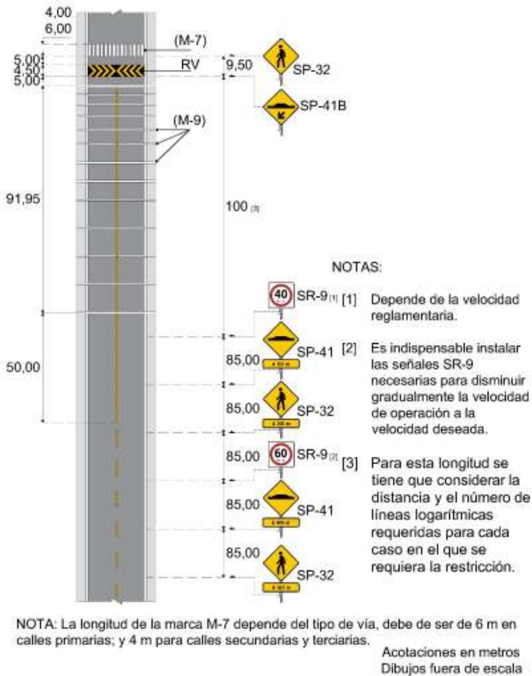
Figura VIII.1-25 Sistema de control de velocidad 5C para cruce de peatones en zona rural
