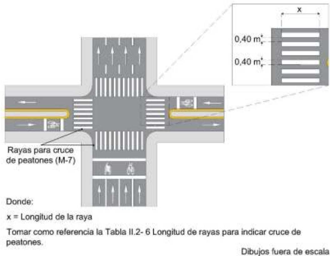
Figura II.2- 18 Rayas para cruce de peatones (M-7)
