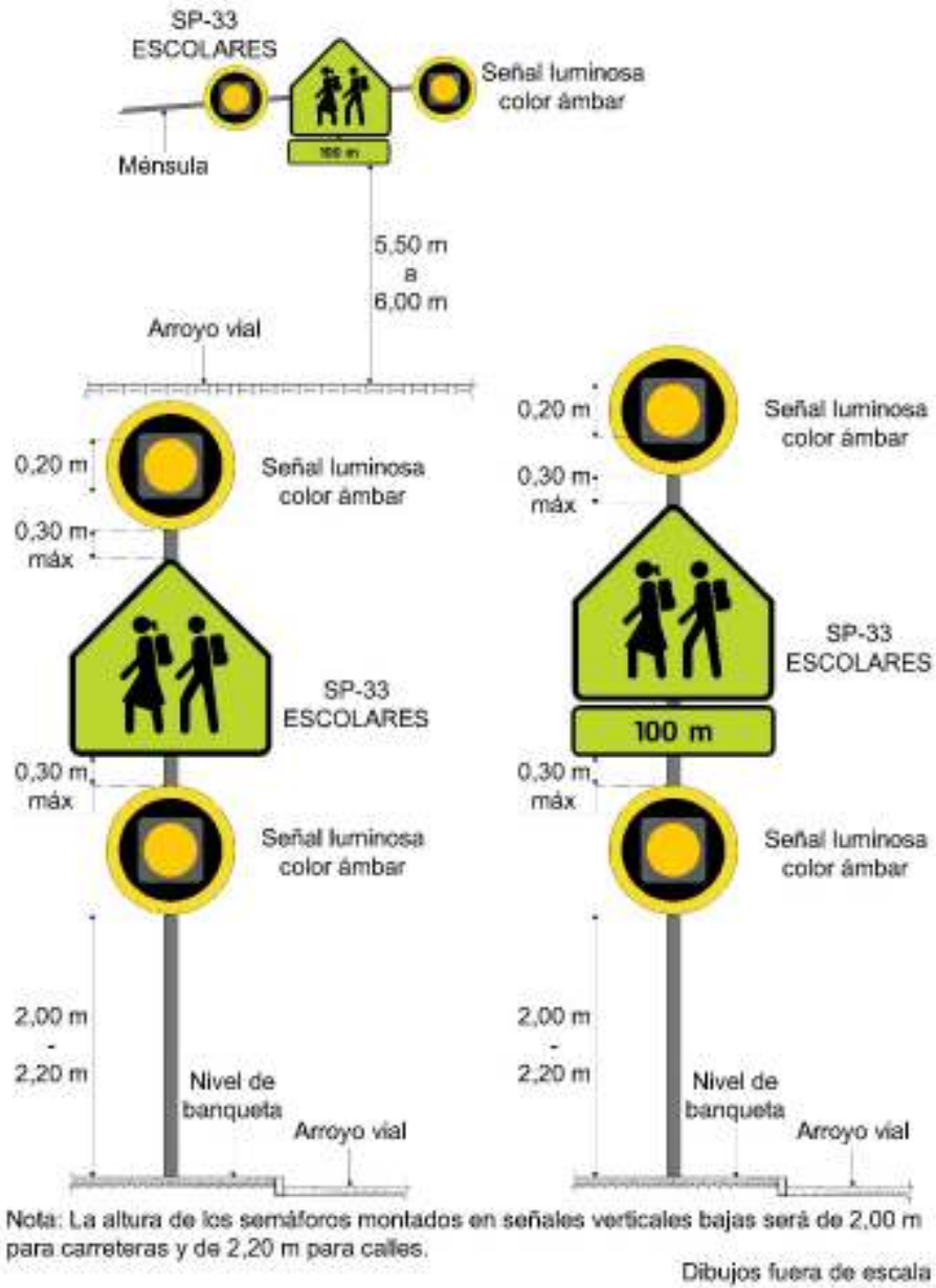
Figura VIII.2-21 Semáforo de destello de zona escolar
