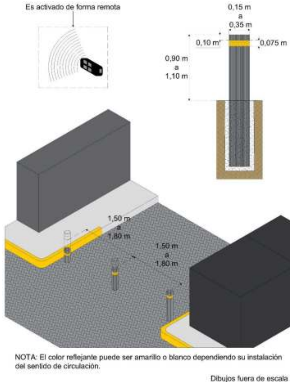
Figura IV.13- 3 Bolardo retráctil
