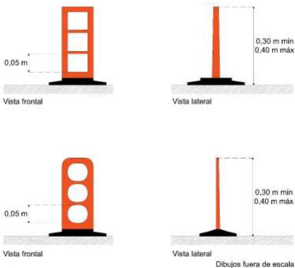
Figura V.6-19 Baliza temporal
