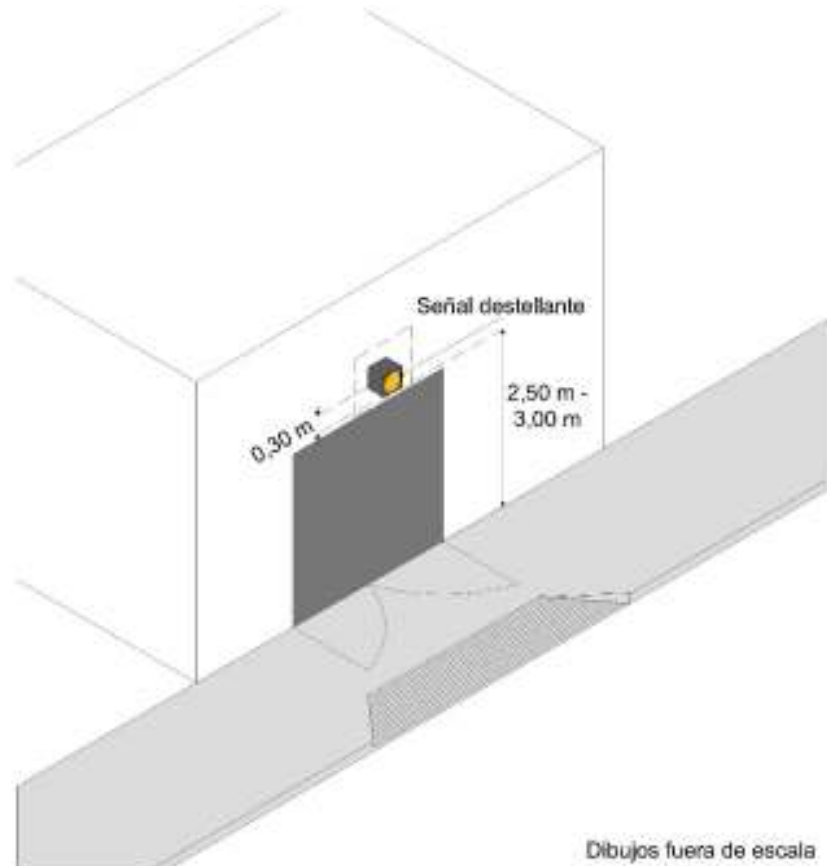
Figura VI.5-16 Semáforo para acceso vehicular a predios
