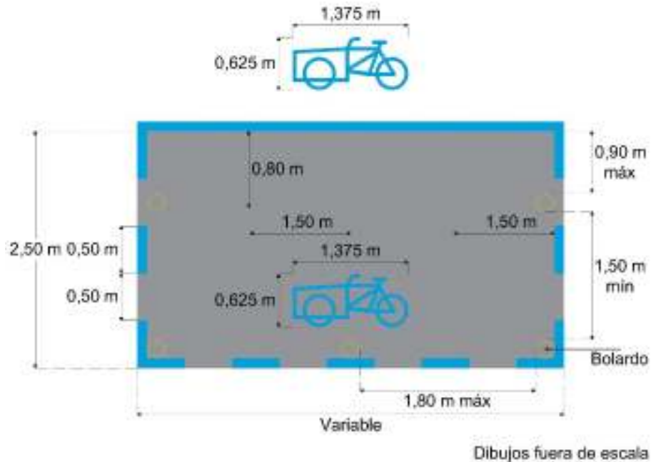
Figura VII.2- 12 Marcas para estacionamiento de bicicletas de carga
