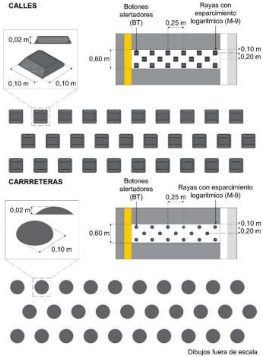
Figura IV.4- 6 Botones alertadores (BT) en rayas con espaciamiento logarítmico
