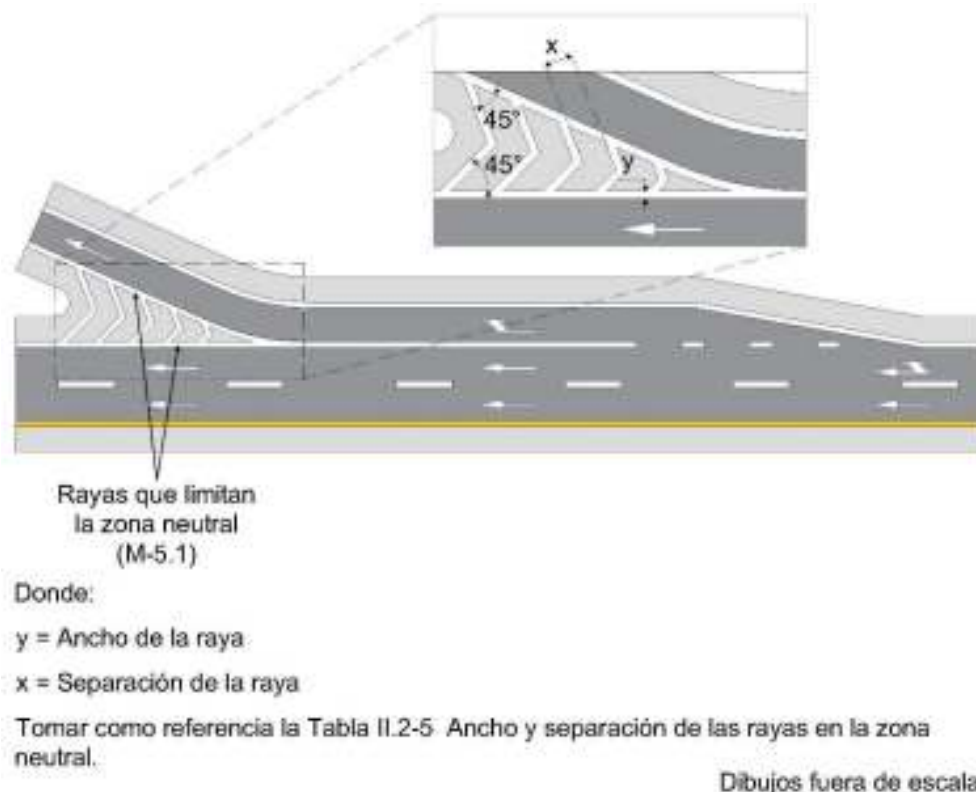
Figura II.2- 15 Rayas que limitan la zona neutral (M-5.1)
