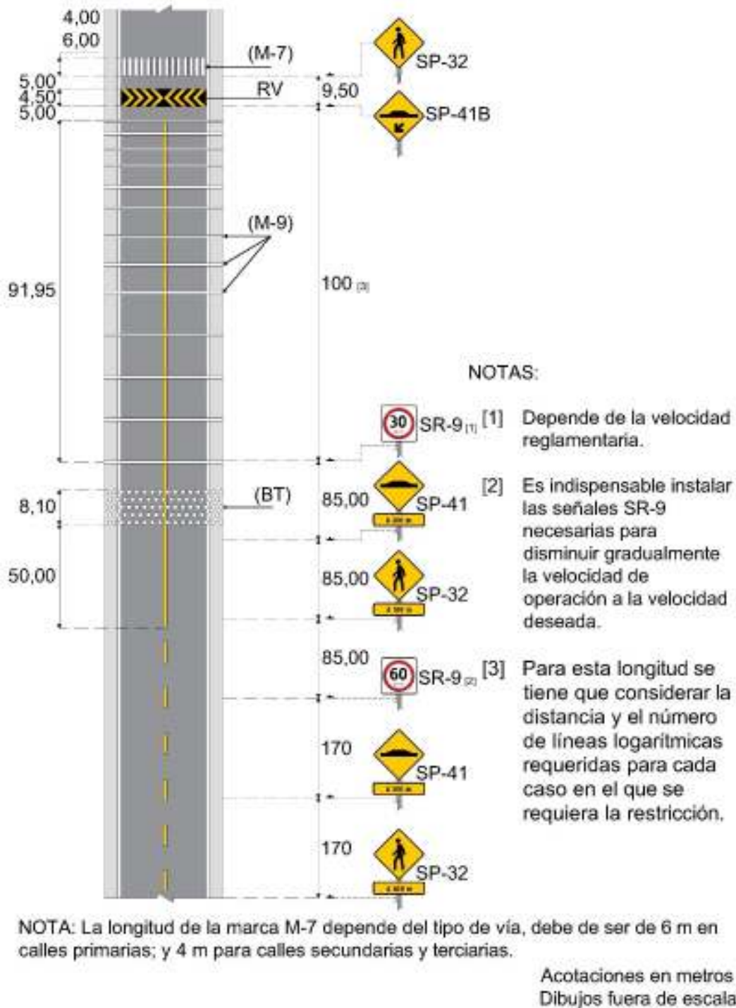
Figura VIII.1-16 Sistema de control de velocidad 1D para cruce de peatones en zona urbana
