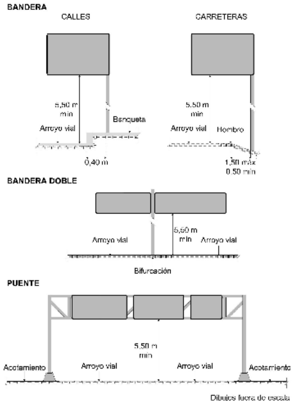
Figura III.8- 7 Ubicación de las señales elevadas
