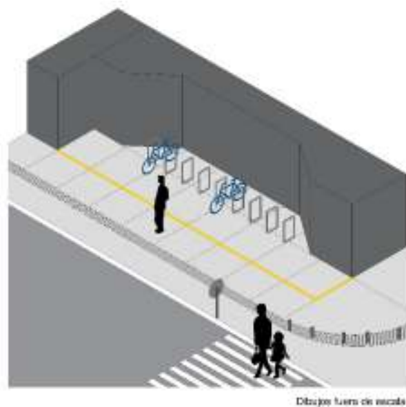
Figura VII.1- 26 Aplicación de pavimento táctil lineal de límite
