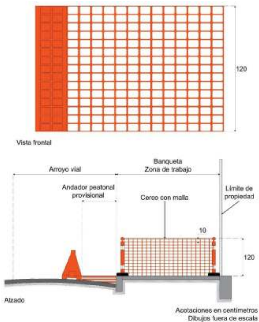
Figura V.6-16 Malla
