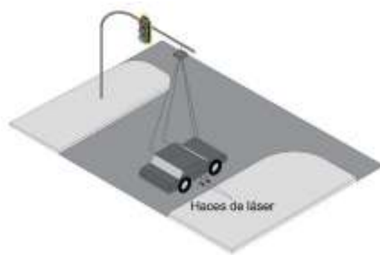
Figura VI.8-8 Configuración de radar con haz láser (infrarrojo activo)
