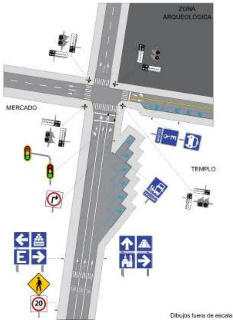
Figura VIII.2- 48 Señalización para estacionamiento en zona turística
