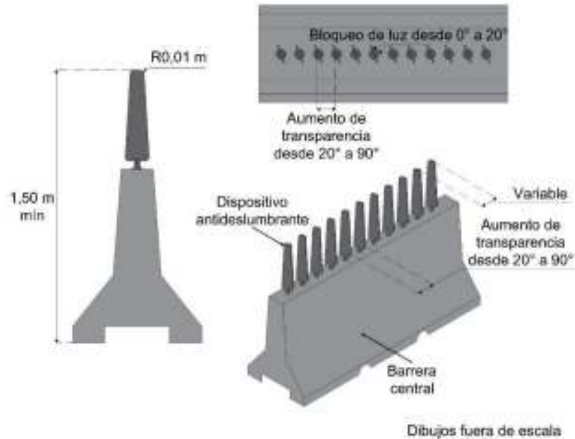
Figura IV.11- 2 Valla antideslumbrante
