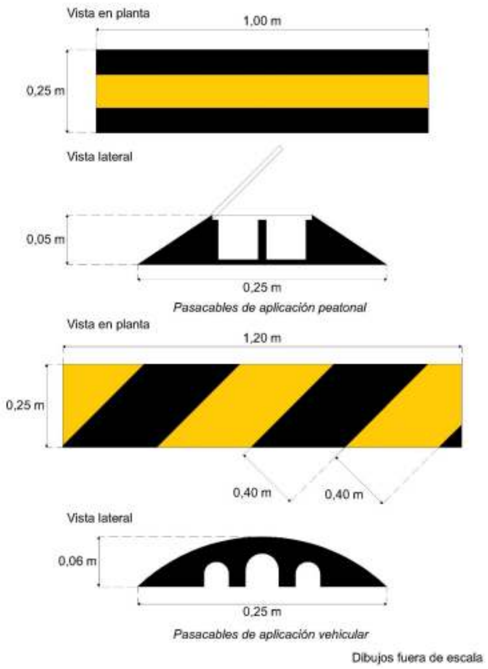
Figura V.6-24 Pasacables
