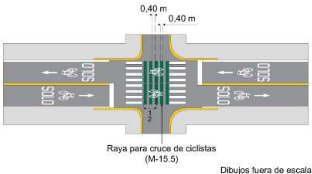
Figura II.2- 51 Rayas para cruce de vía ciclista bidireccional
