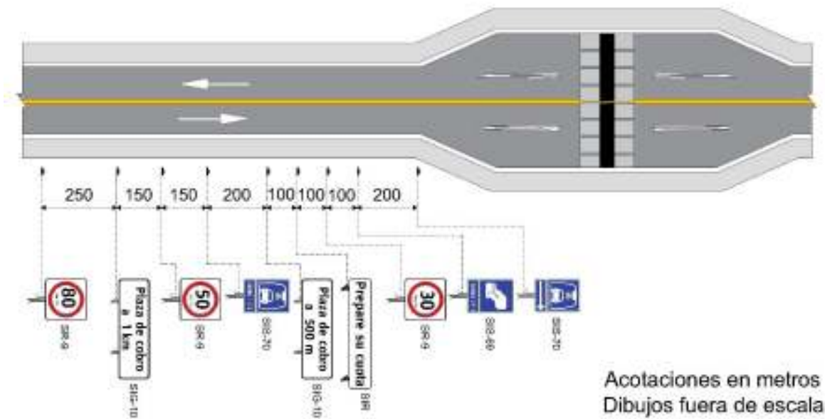
Figura VIII.2-13 Ejemplo de aplicación de la señalización previa a la plaza de cobro
