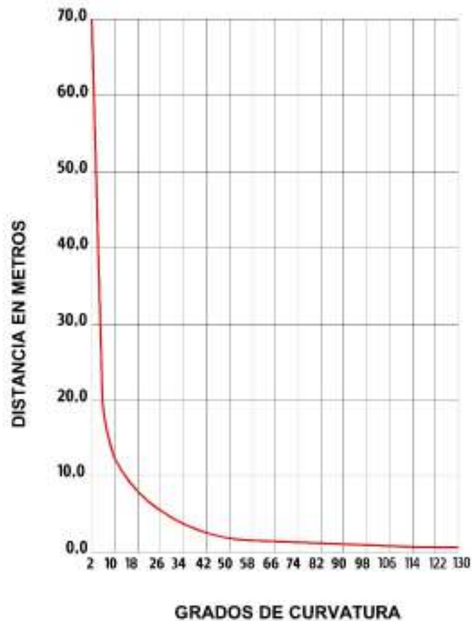
Figura III.6- 6 Distancia máxima de espaciamiento entre indicadores de curva cerrada OD-12
