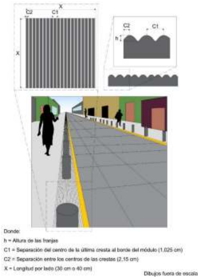
Figura VII.1- 25 Franja lineal de límite lateral con bolardos
