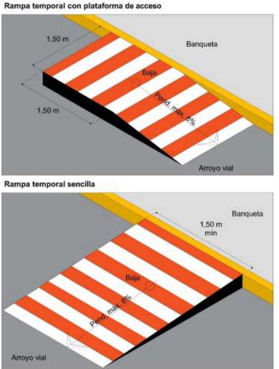
Figura V.6-22 Rampas temporales
