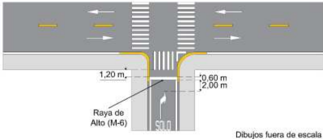
Figura II.2- 17 Rayas de alto (M-6)
