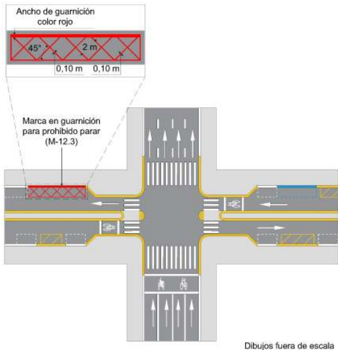
Figura II.2- 40 Marca para prohibición de parar (M-12.3)
