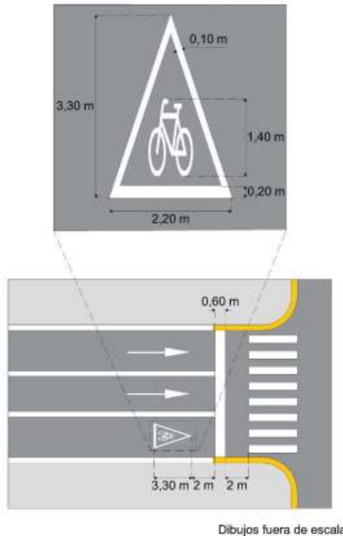
Figura II.2- 47 Marca para identificar vía ciclista con prioridad de uso (M-15.2)
