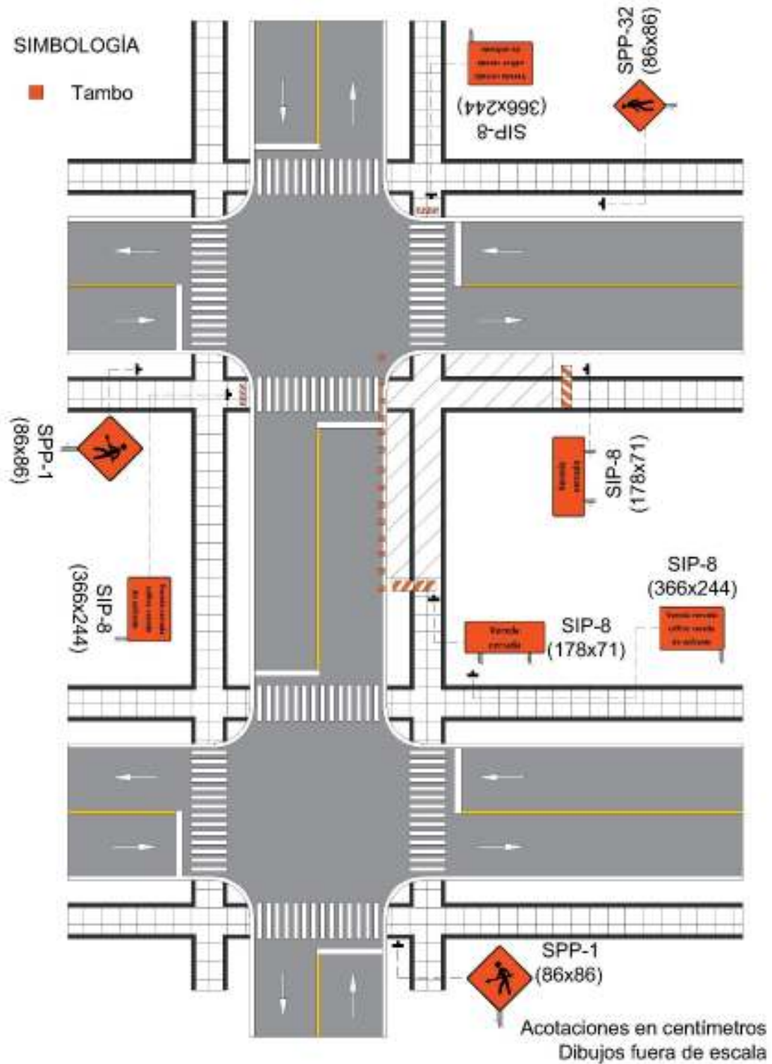
Figura V.10-19 Cierre de cruce peatonal y desvío de peatones (Vía con ancho de arroyo vial menor a 9 m)
