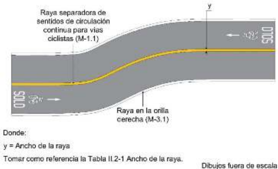
Figura VII.2- 5 Raya continua sencilla para vías ciclistas (M-1.1)
