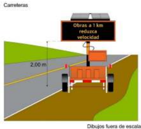
Figura VI.4-7 SMV Portátil
