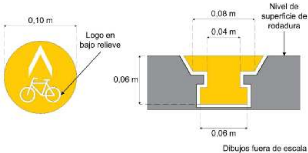
Figura IV.4- 5 Botones ciclistas para áreas peatonales
