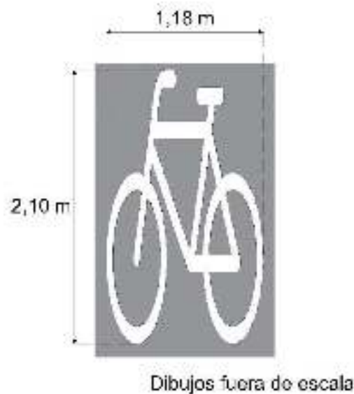
Figura VII.2- 17 Pictograma de bicicleta para vías ciclistas
