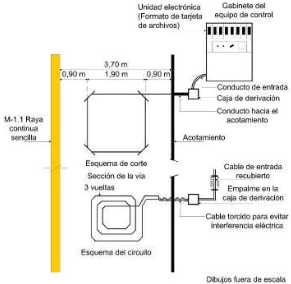
Figura VI.8-1 Lazos inductivos
