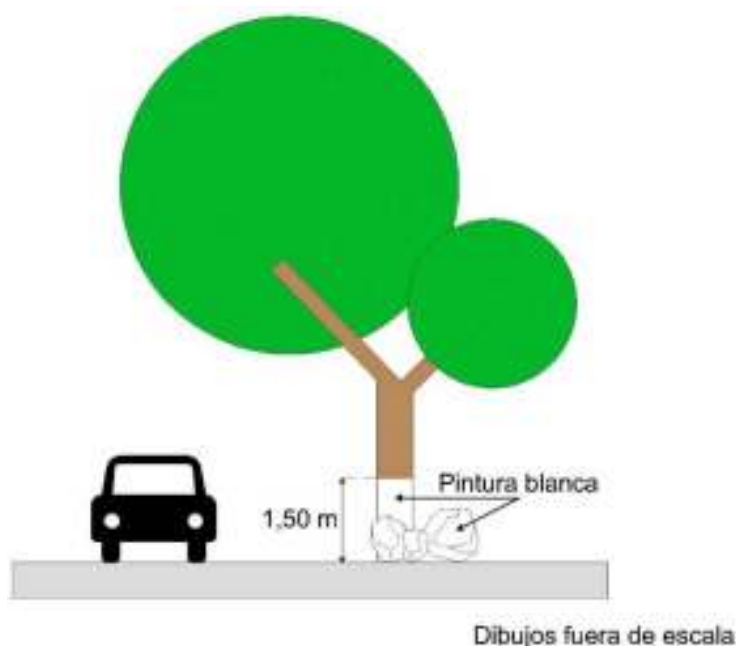
Figura II.2- 43 Marcas en otros objetos (M-13.2)
