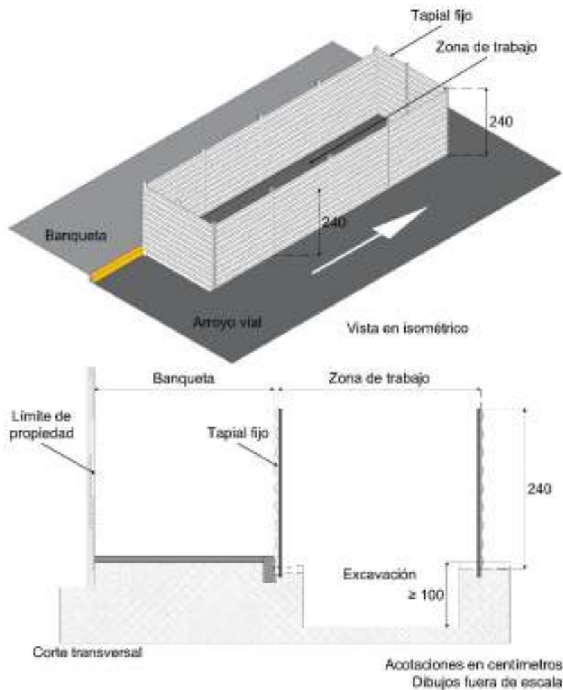
Figura V.6-18 Tapial fijo
