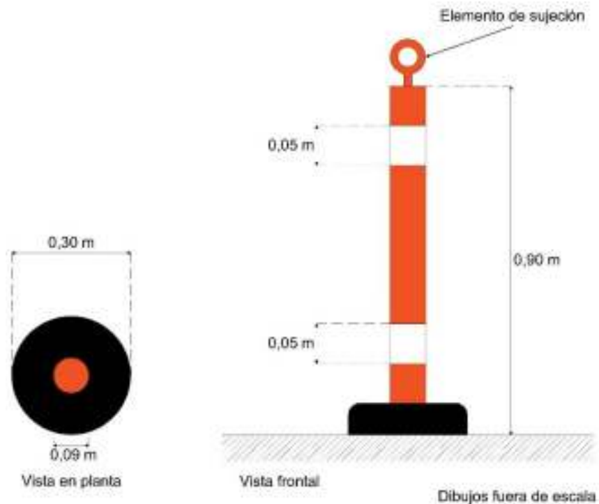
Figura V.6-20 Baliza delineadora
