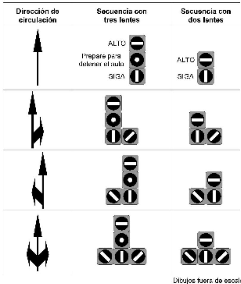
Figura VIII.2-36 Semáforos para la circulación de transporte público
