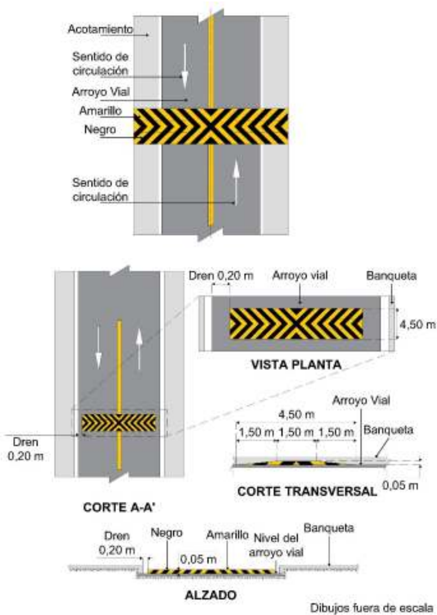
Figura IV.9- 2 Reductor de velocidad en carreteras
