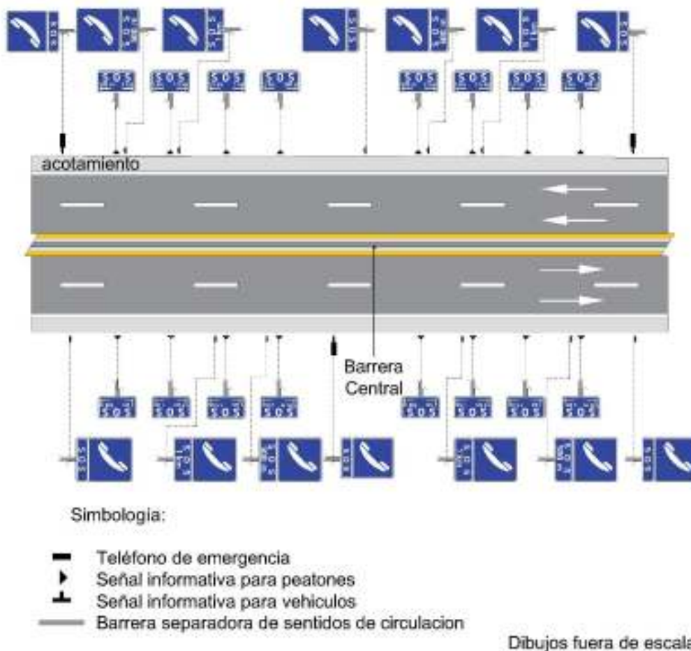
Figura VIII.1-2 Ubicación de la señalización informativa de cabinas telefónicas de emergencia (SOS)
