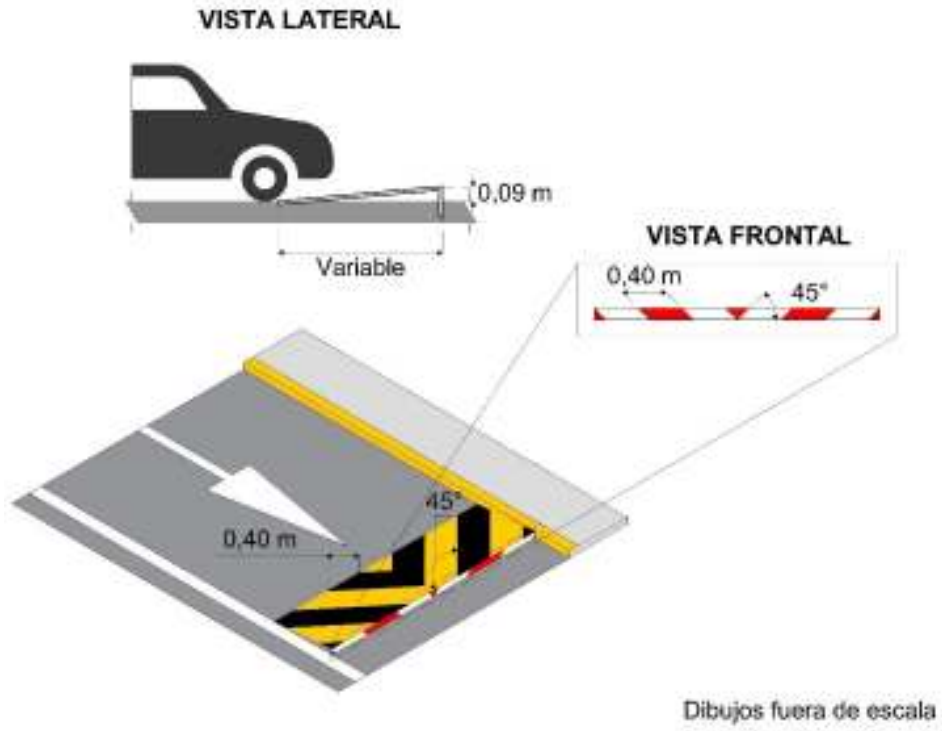
Figura IV.10- 1 Limitadores de sentido
