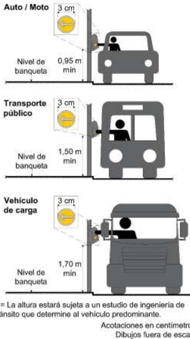
Figura VI.6-4 Botón de solicitud de paso vehicular
