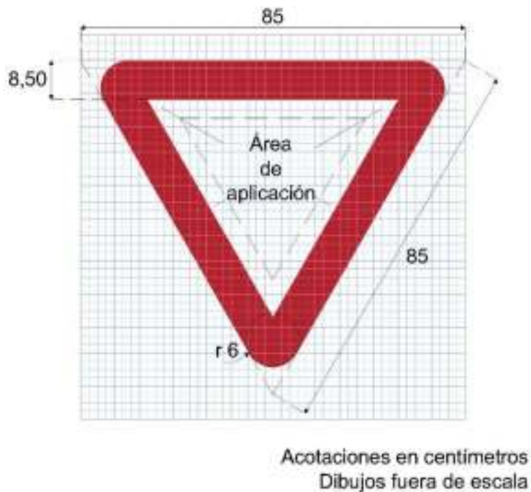
Figura III.3-4 Área de aplicación para la señal SR-7 Ceda el paso
