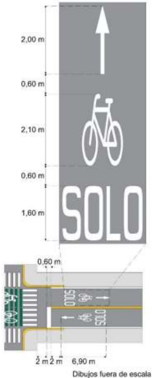
Figura II.2- 46 Marca para vías ciclistas
