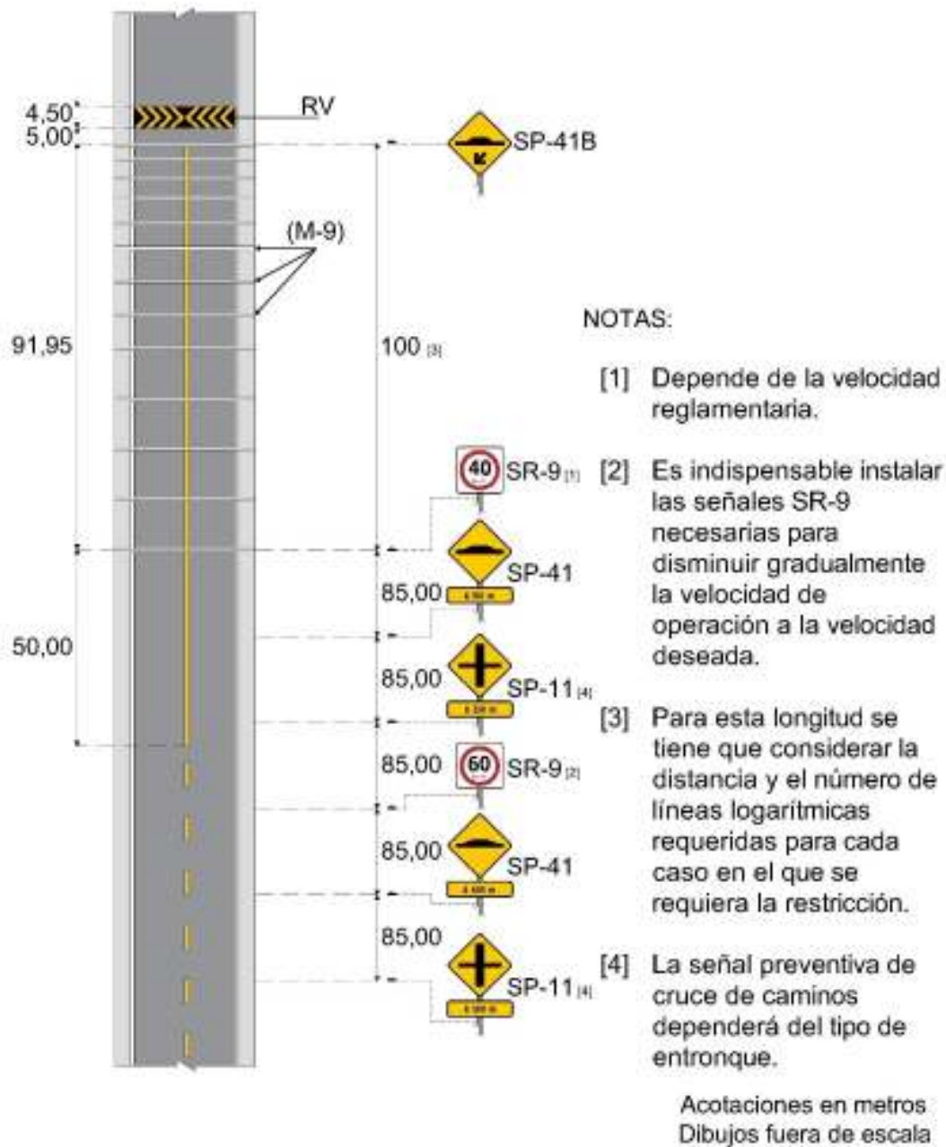
Figura VIII.1-20 Sistema de control de velocidad 3C para intersección próxima
