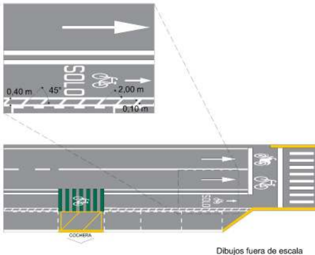
Figura II.2- 49 Rayas de protección al ciclista (M-15.4)
