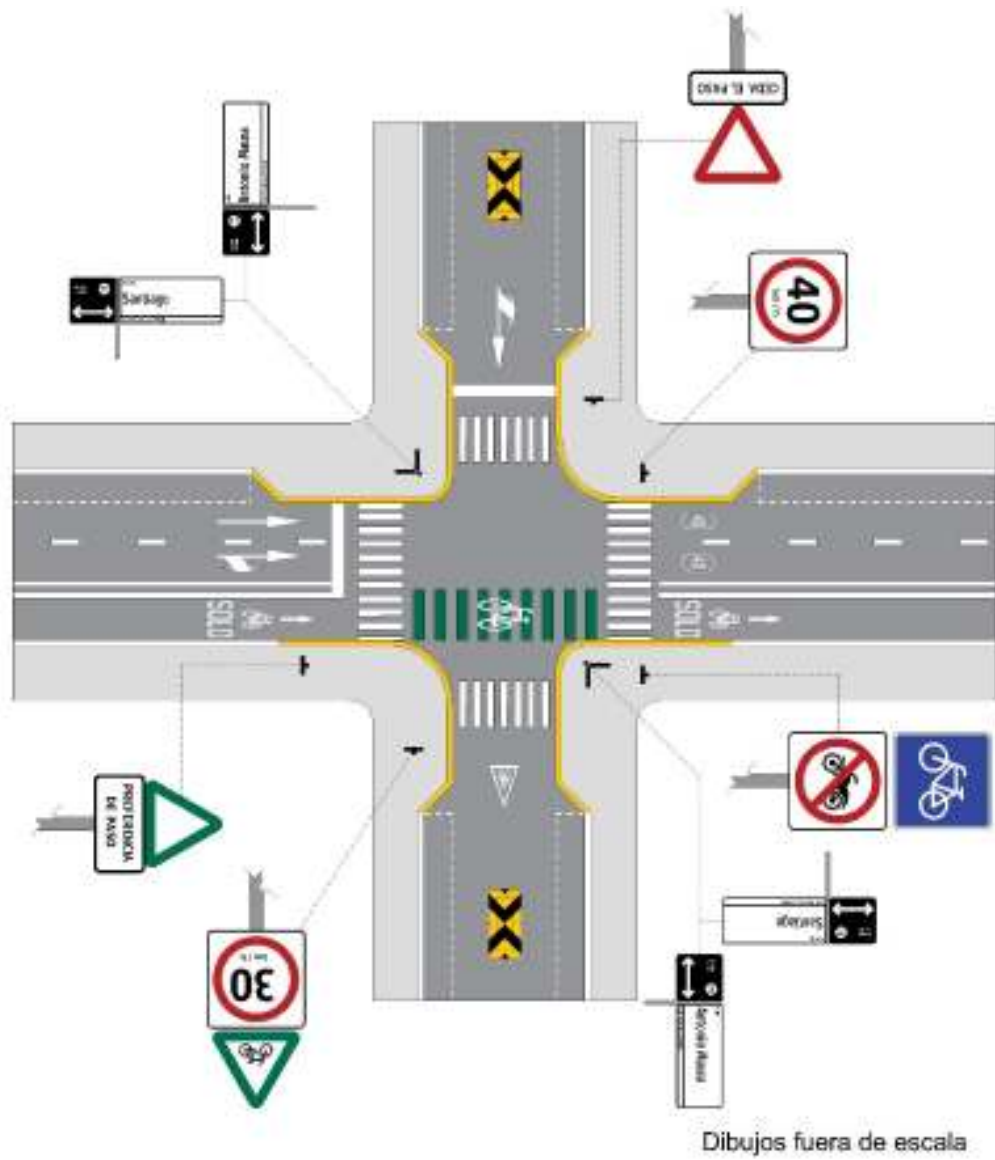
Figura VIII.2- 46 Intersección simple
