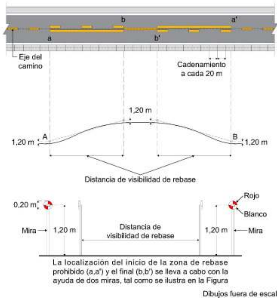
Figura A2- 3 Procedimiento para ubicar los límites de los tramos de rebase prohibido en curvas verticales
