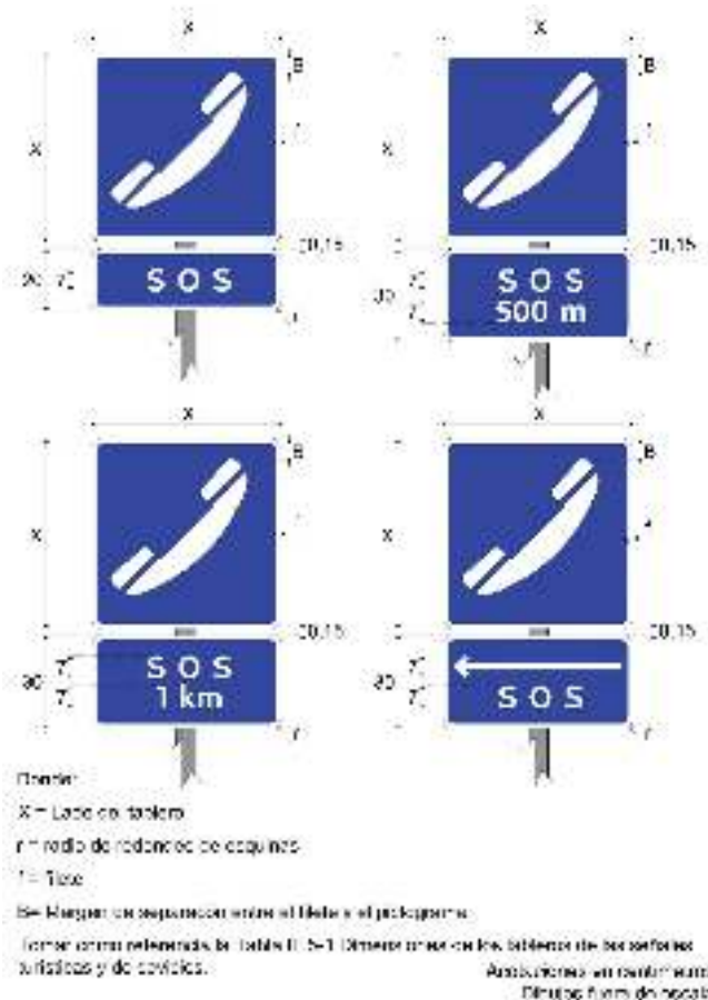
Figura VIII.1-3 Señales informativas para vehículos (SOS)
