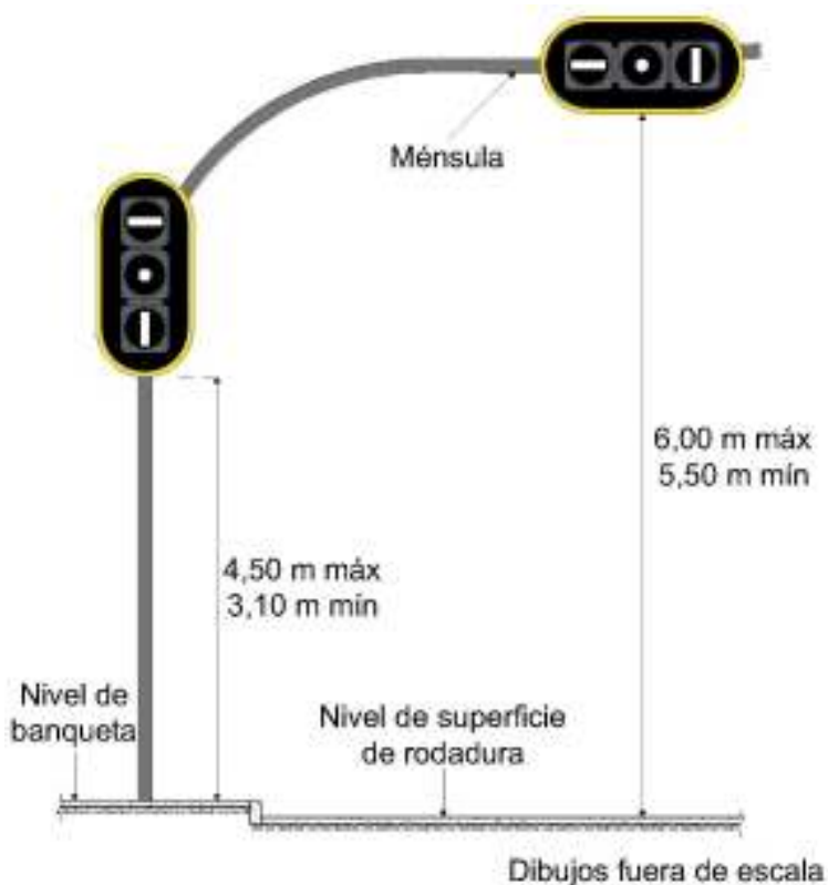
Figura VI.5-6 Soporte vertical y disposición horizontal
