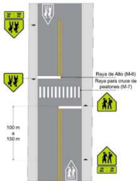
Figura VIII.2-17 Cruce escolar
