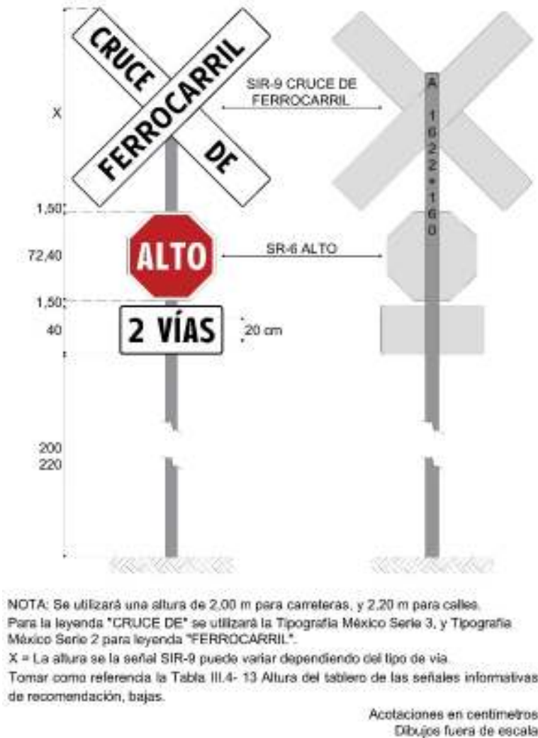
Figura VIII.1-5 Señalización para CRUCE DE FERROCARRIL
