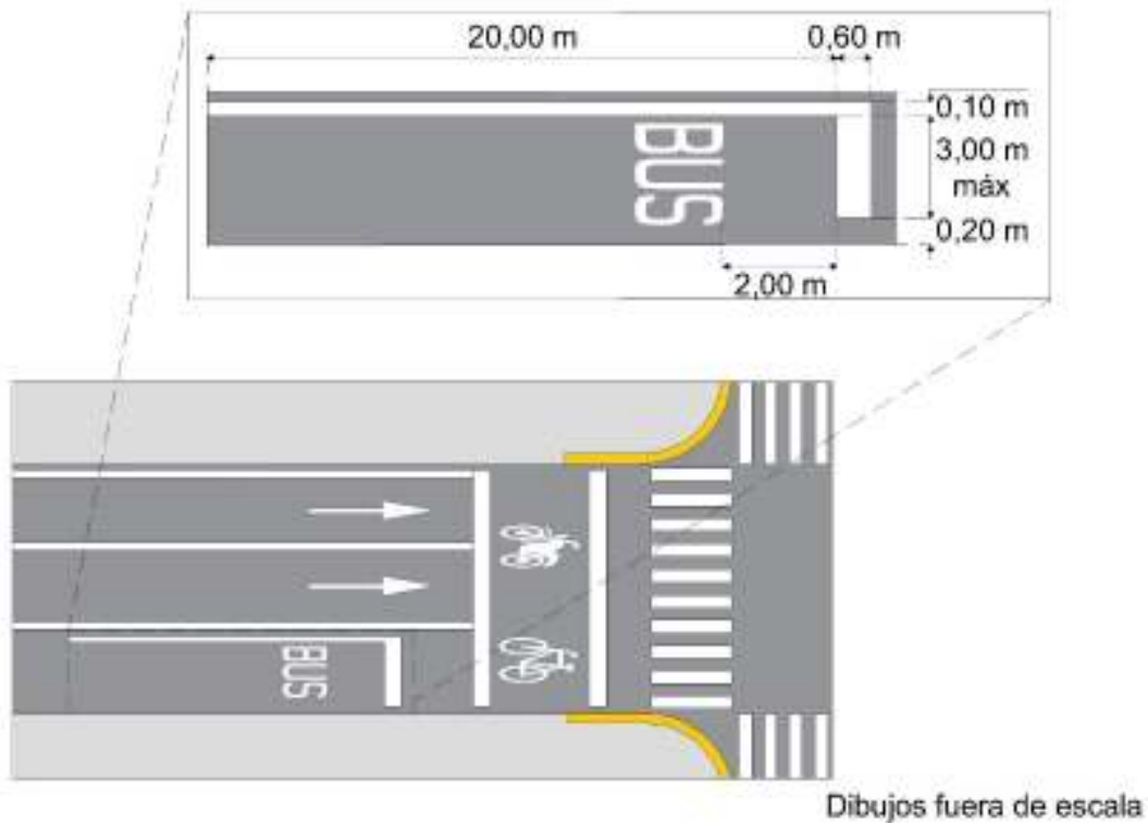
Figura II.2- 34 Marcas para establecer lugares de parada (M-11.3)
