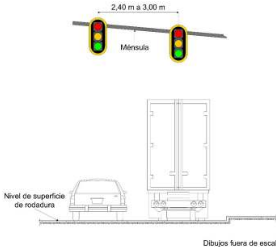
Figura VI.5-30 Colocación de dos caras de semáforo (Ubicación)
