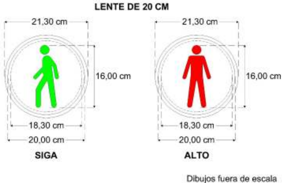
Figura VI.5-2 Inscripciones en la señal luminosa en semáforo para peatones
