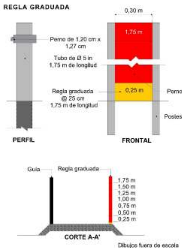
Figura III.6- 4 Regla graduada
