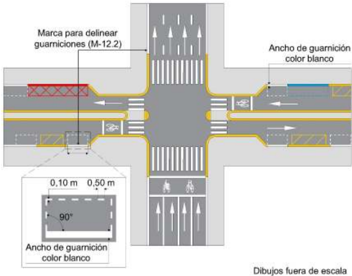
Figura II.2- 39 Marca para delinear guarniciones (M-12.2)
