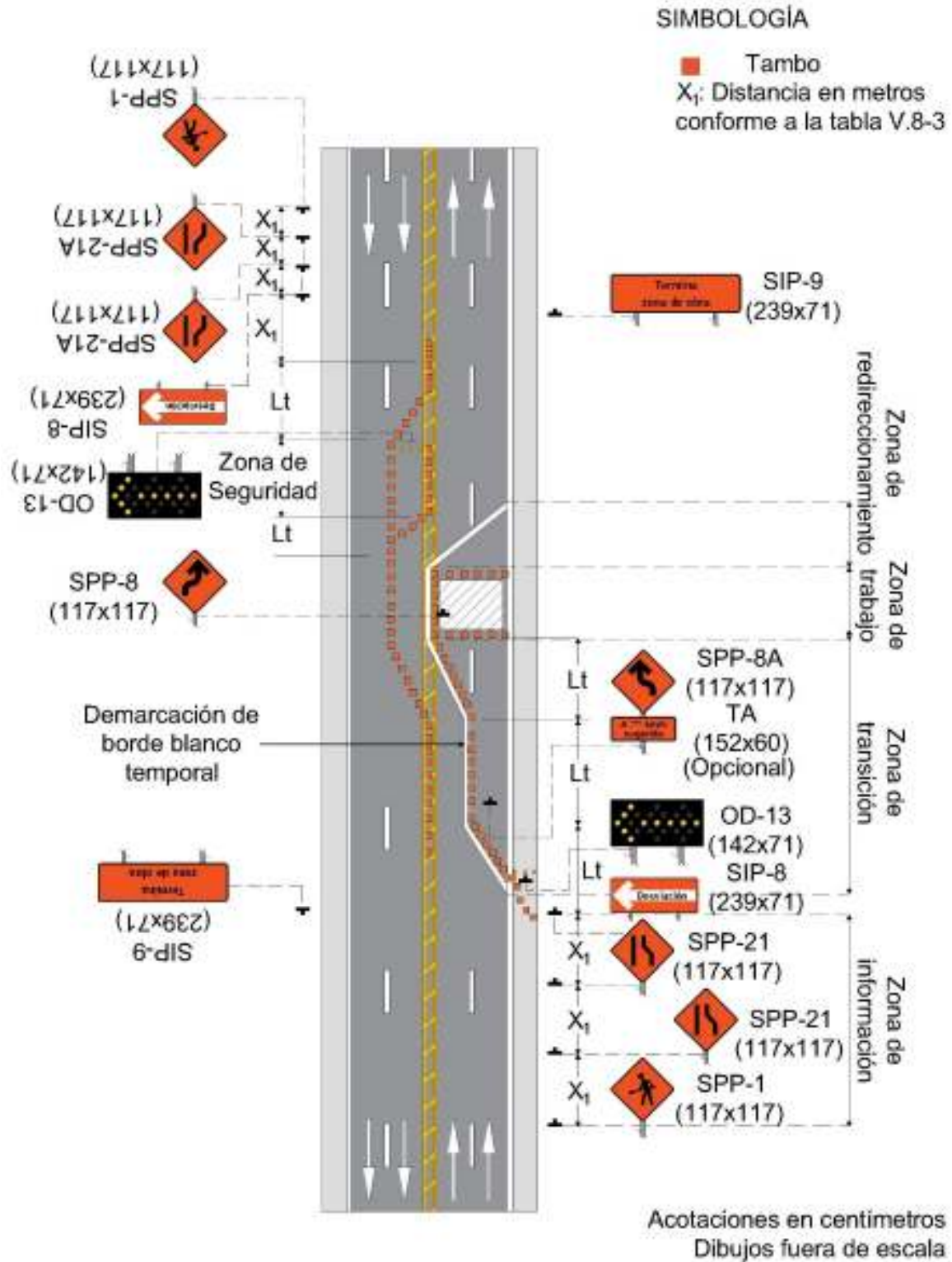
Figura V.10-22 Cierre de mitad de vía de alta velocidad en una vía de múltiples carriles (Vía de 4 o más carriles)
