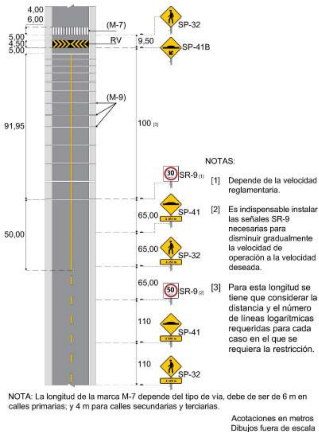
Figura VIII.1-15 Sistema de control de velocidad 1C para cruce de peatones en zona urbana
