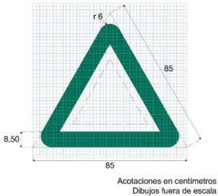
Figura III.3-5 Área de aplicación para la señal SR-7 Preferencia de paso
