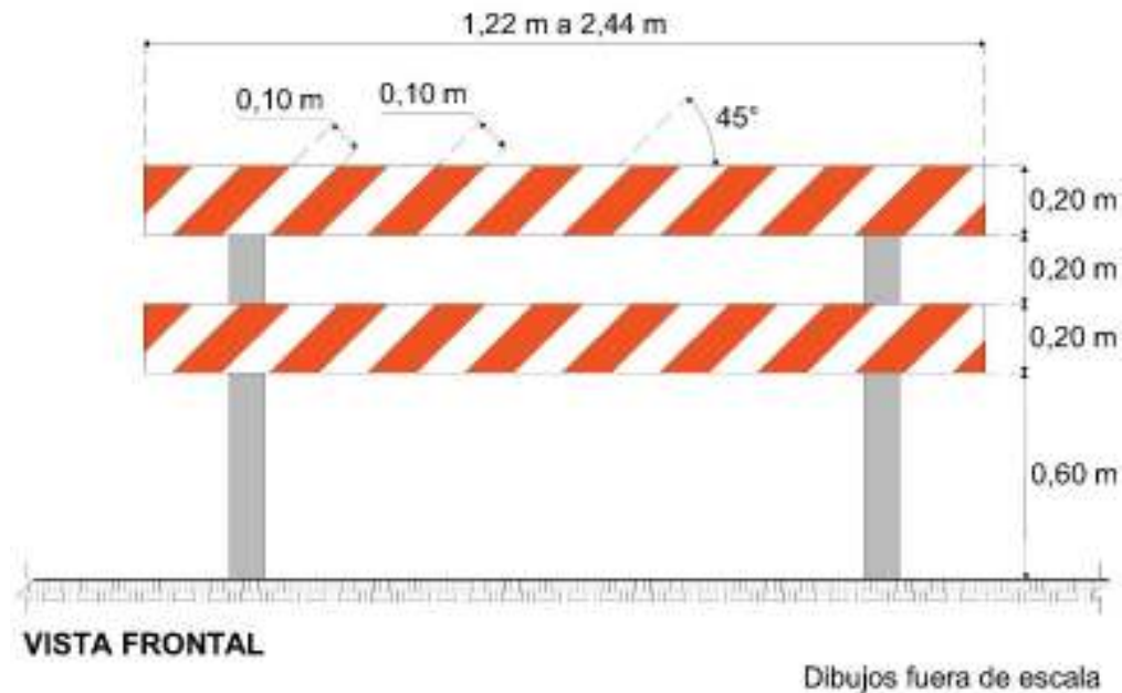
Figura V.6-2 Barrera fija
