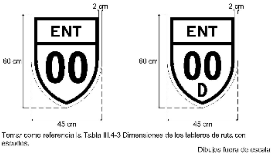
Figura III.4- 25 Trazo del escudo de carretera estatal SII-9
