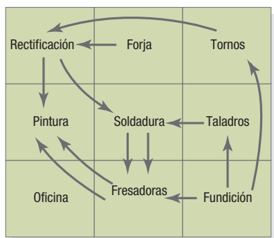
(a) Distribución de un taller de trabajo
