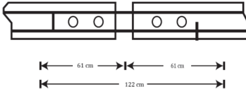
Figura 9 Junta de clase 3 a 5.
