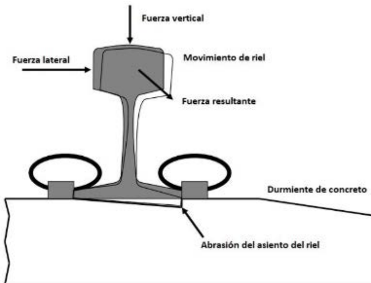
Figura 15 Desgaste de durmiente.
