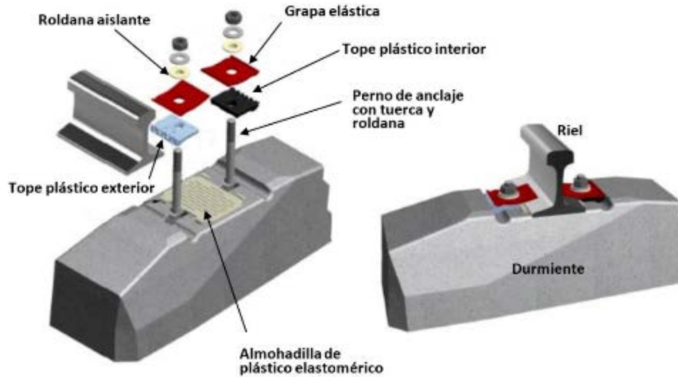
Figura 6 Sistema de fijación en vía elástica.
