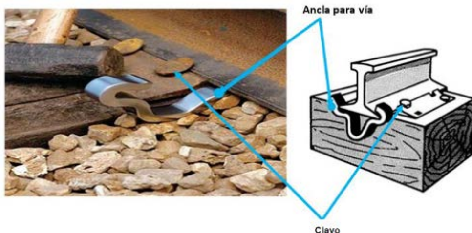
Figura 5 Sistema de fijación en vía clásica.
