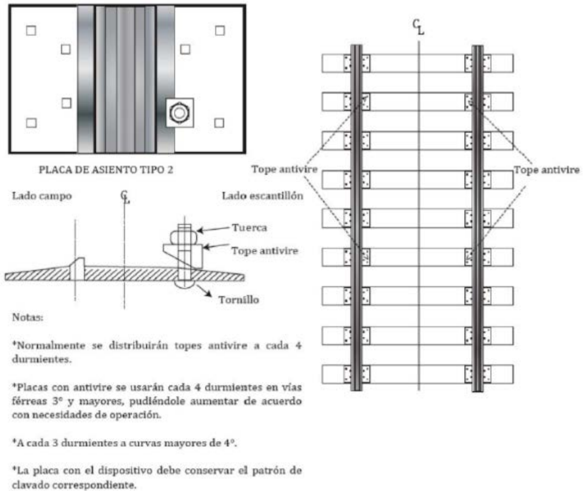
Figura 4 Dispositivos antivire.
