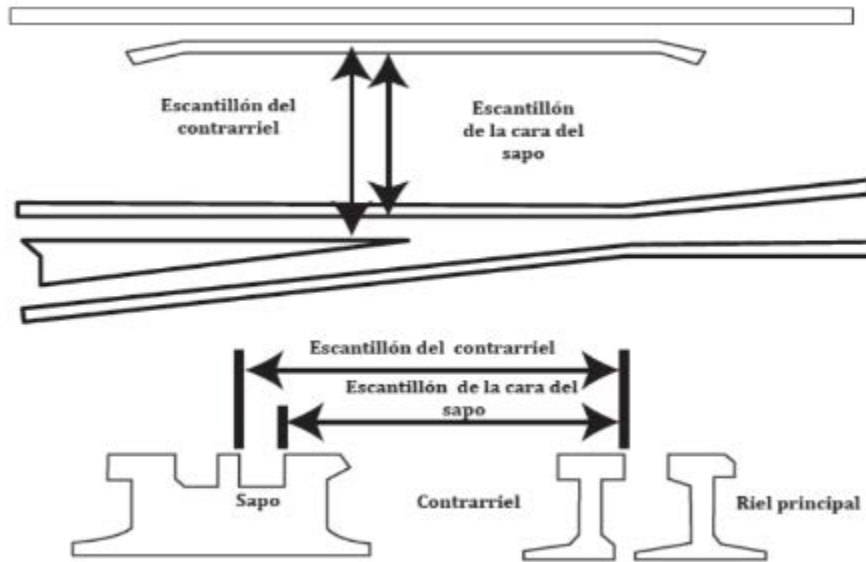
Figura 14 Escantillón de sapo y contrarriel.
