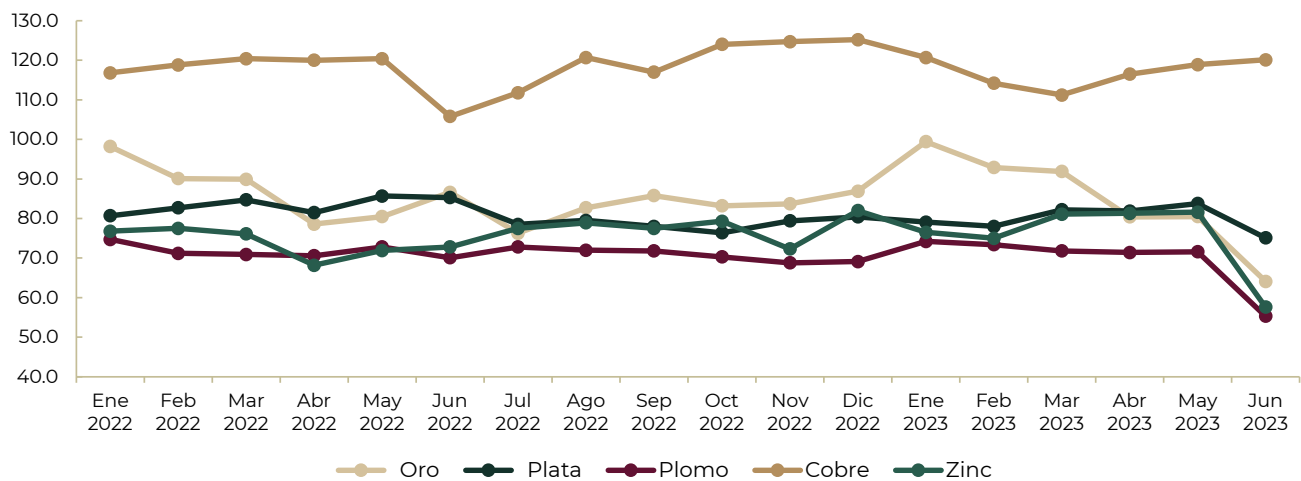
Índice de volumen físico de la producción minero-metalúrgica (Metales Preciosos e Industriales No Ferrosos)
