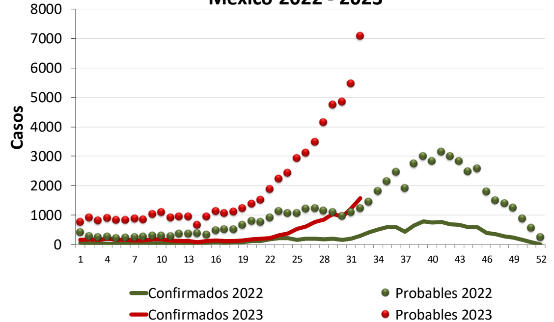
Casos de dengue Probables y Confirmados. México 2022 - 2023
