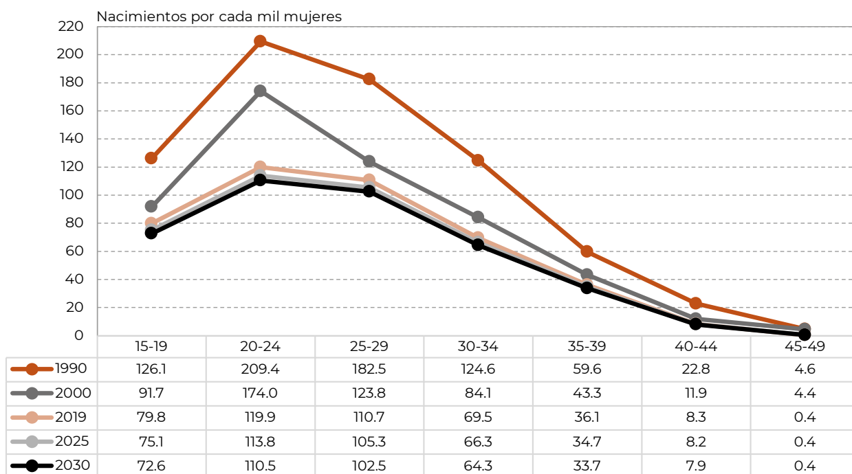
Gráfica 5.3. Campeche. Tasas específicas de fecundidad, 1990-2030
