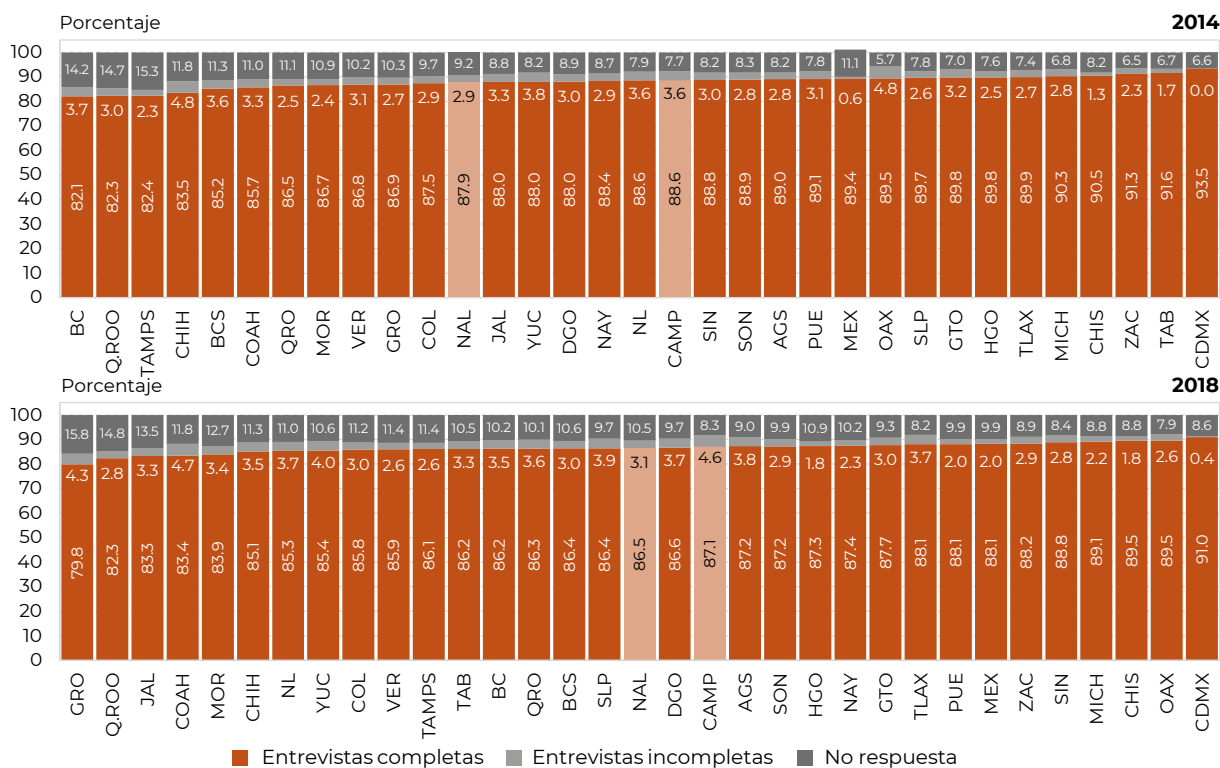
Gráfica 1.1. Porcentaje de entrevistas completas, incompletas y tasa de no respuesta en las viviendas al final del levantamiento de la ENADID 2014 y 2018 por coordinación estatal
