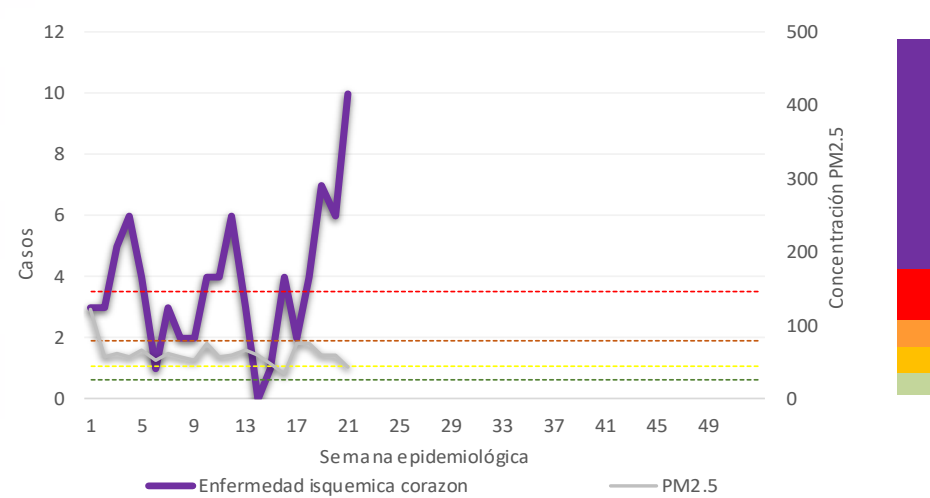
Casos de Enfermedad Isquémica del Corazón y niveles máximos de PM 2.5 por semana epidemiológica. Región Noroeste– ZMVM, 2023
