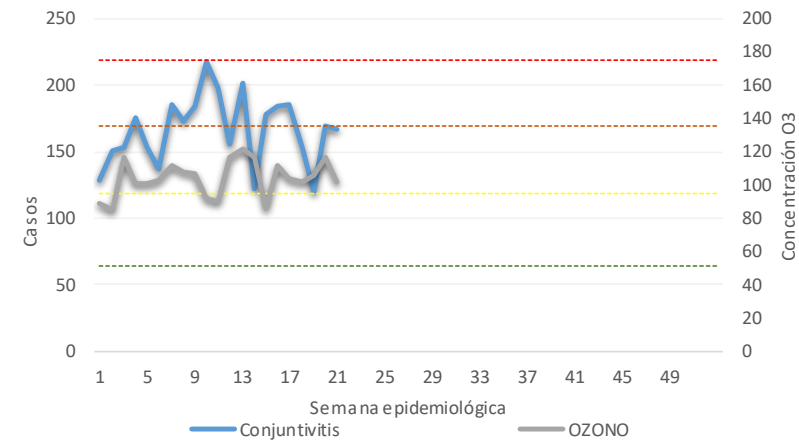
Casos de Conjuntivitis y niveles máximos de ozono por semana epidemiológica. Región Noreste – ZMVM, 2023
