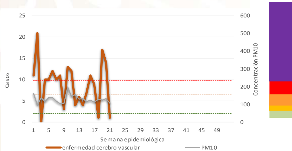
Casos de Enfermedad Cerebro Vascular y niveles máximos de PM10 por semana epidemiológica. Región Centro – ZMVM, 2023
