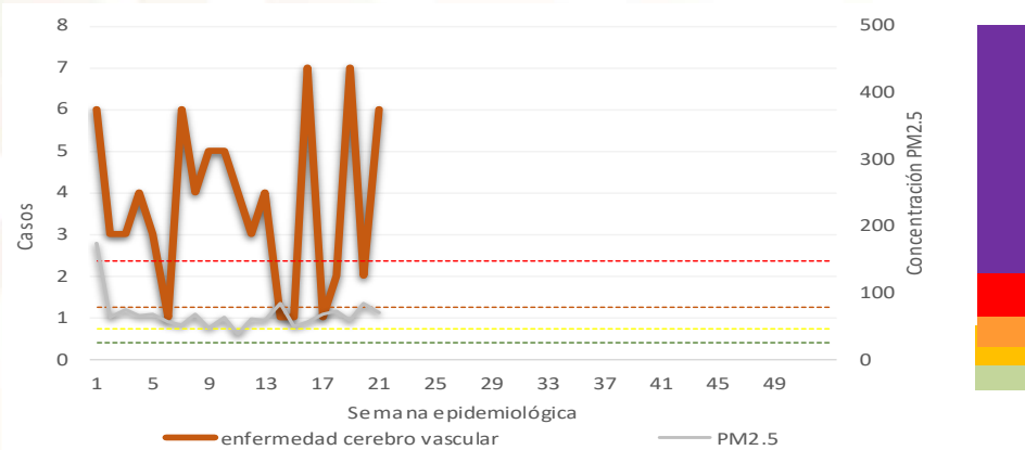
Casos de Enfermedad Cerebro Vascular y niveles máximos de PM 2.5 por semana epidemiológica. Región Sureste – ZMVM, 2023
