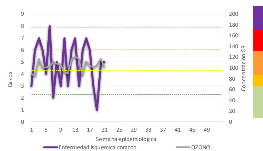
Casos de Enfermedad Isquémica del Corazón y niveles máximos de ozono por semana epidemiológica. Región Noreste – ZMVM, 2023
