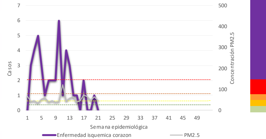
Casos de Enfermedad Isquémica del Corazón y niveles máximos de PM 2.5 por semana epidemiológica. Región Suroeste– ZMVM, 2023
