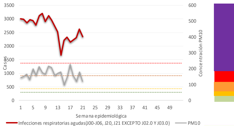
Casos de Infecciones Respiratorias Agudas (IRA) y niveles máximos de PM 10 por semana epidemiológica. Región Noroeste – ZMVM, 2023
