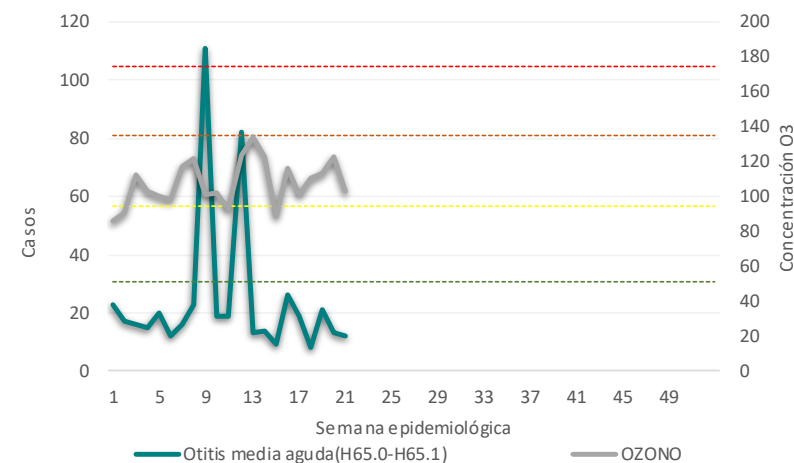
Casos de Otitis Media Aguda y niveles máximos de ozono por semana epidemiológica. Región Centro – ZMVM, 2023
