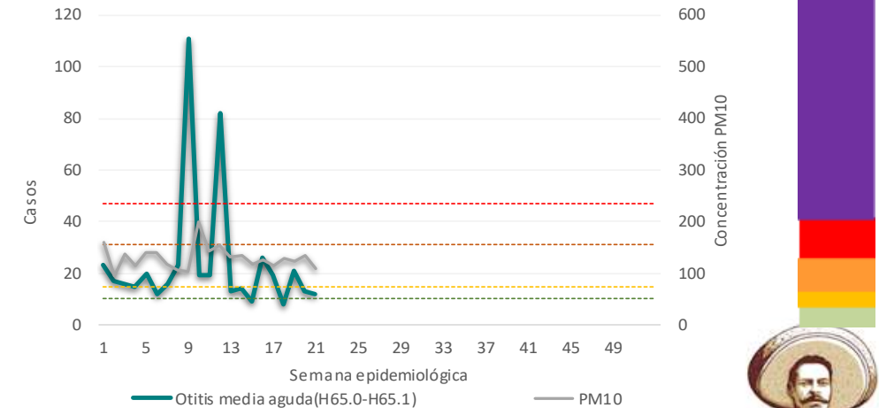
Casos de Otitis Media Aguda y niveles máximos de PM 10 por semana epidemiológica. Región Centro – ZMVM, 2023
