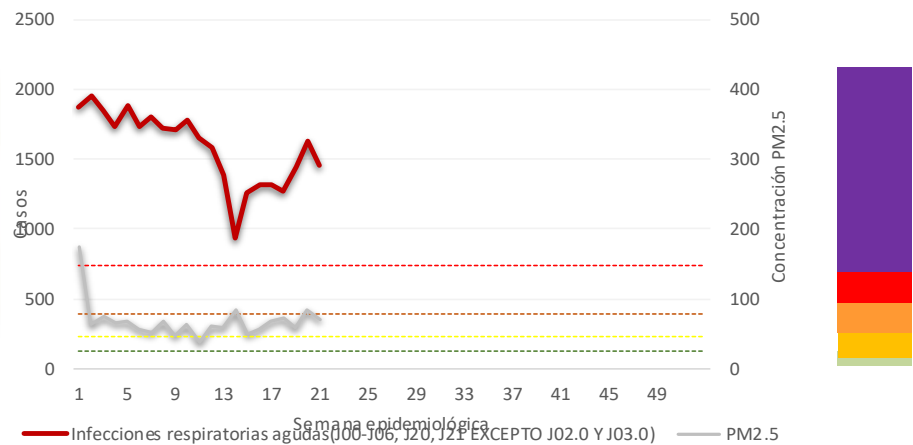
Casos de Infecciones Respiratorias Agudas (IRA) y niveles máximos de PM 2.5 por semana epidemiológica. Región Sureste – ZMVM, 2023
