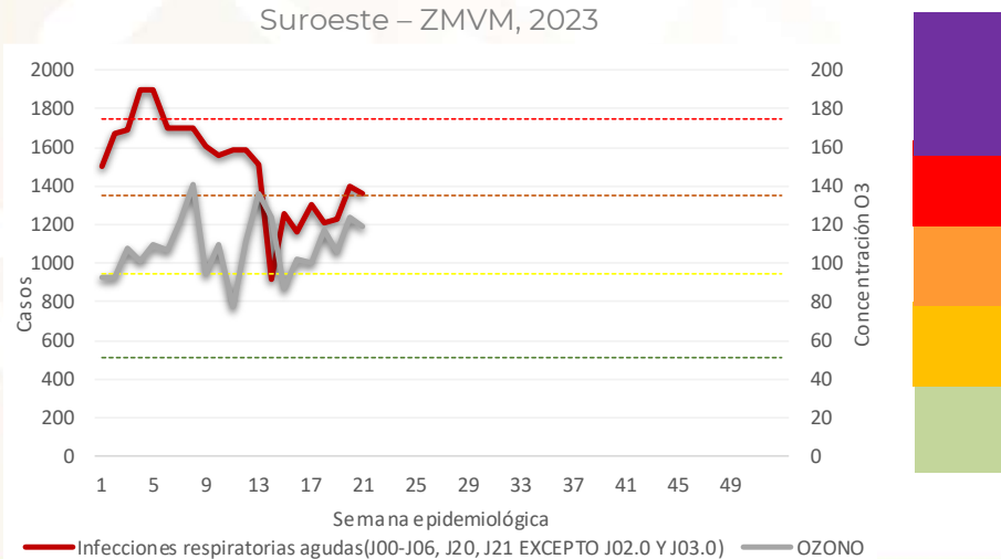
Casos de Infecciones Respiratorias Agudas (IRA) y niveles máximos de ozono por semana epidemiológica. Región Suroeste – ZMVM, 2023
