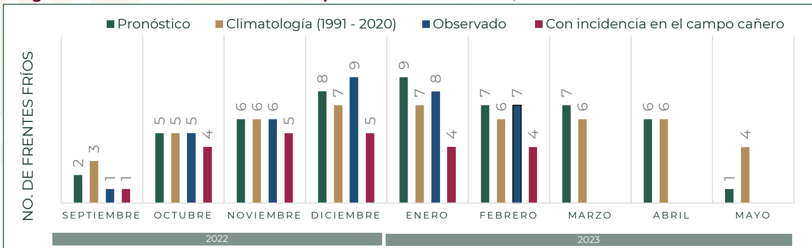
Gráfica: Perspectiva y seguimiento de Frentes Fríos con incidencia en el campo cañero. Temporada invernal 2022/2023. Elaboró: CONADESUCA. Fuente: SMN. Pronóstico de Frentes Fríos. http://smn.conagua.gob.mx/es/climatologia/pronostico-climatico/frentes-frios
