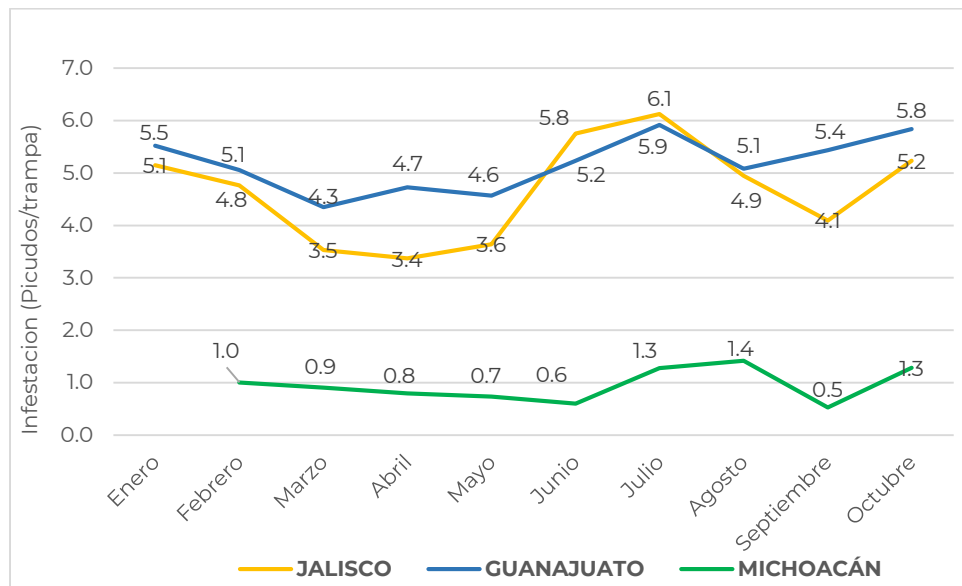
Gráfica 1. Promedio mensual de picudos capturados por trampa a nivel estatal en el marco de la campaña contra plagas reglamentadas del agave, durante el periodo de enero a octubre de 2022.
