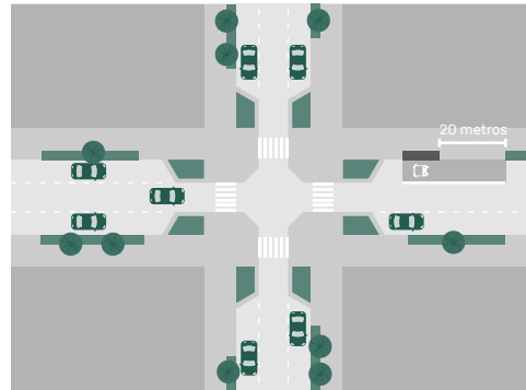
Cruce peatonal perpendicular con ampliación de acera y parada de transporte
