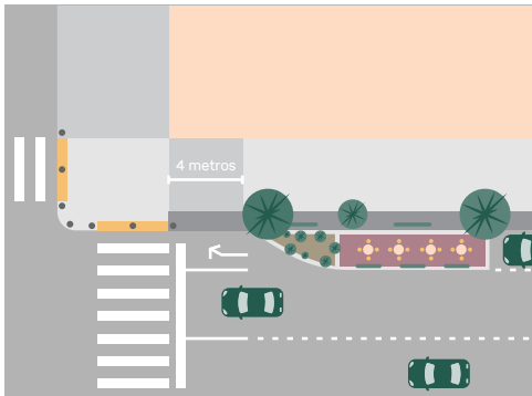
Cruce peatonal en esquina con ampliación de acera con jardín de lluvia y enseres
