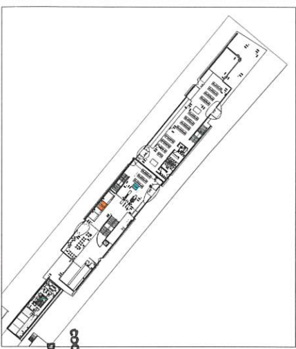
PLANTA ALTA DEL EDIFICIO TERMINAL
