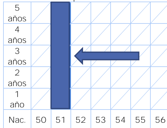
Figura 1.2 Análisis transversal para la construcción de tablas de mortalidad.
