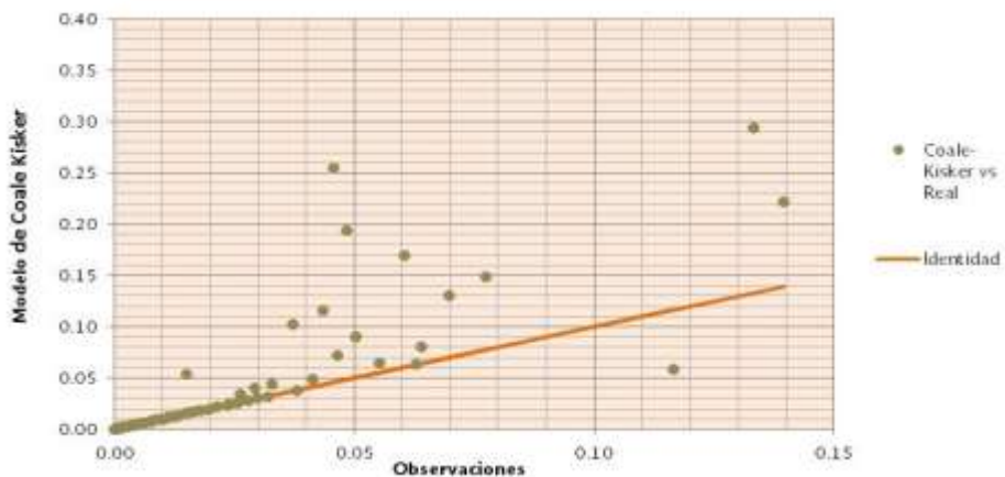
Figura 2.6.2 Cuantil-Cuantil modelo de Coale-Kisker vs observaciones aplicado a la mortalidad mexicana 2000-I.
