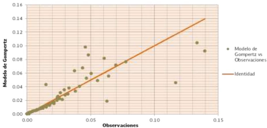
Figura 2.3.3 Cuantil-Cuantil modelo de Gompertz vs observaciones aplicado a la mortalidad mexicana 2000-I.
