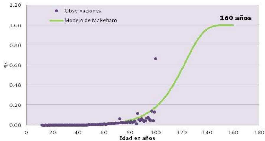
Figura 2.4.1 Modelo de Makeham aplicado a los datos base de mortalidad mexicana 2000-I 19 .
