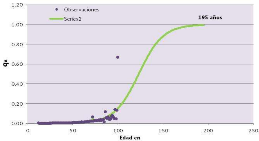
Figura 2.7.3 Modelo logit aplicado a los datos base de mortalidad mexicana 2000-I. Parámetros estimados por la CNSF-2000-I 33 .
