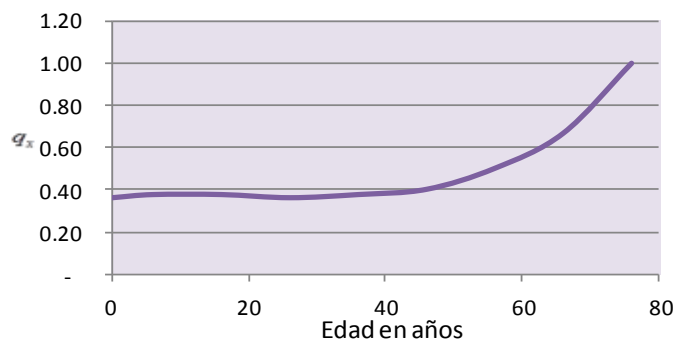
Figura 2.1 Mortalidad de Londres en 1662 según John Graunt.
