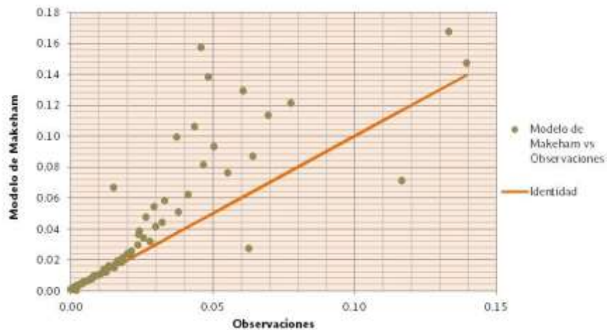
Figura 2.4.2 Cuantil-Cuantil modelo de Makeham vs observaciones aplicado a la mortalidad mexicana 2000-I.
