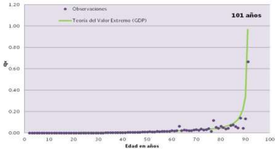
Figura 3.1.1 Teoría de extremos (GPD) aplicada a los datos base de mortalidad mexicana CNSF-2000-I 43 .
