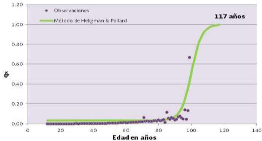
Figura 2.5.1 Modelo de Heligman & Pollard aplicado a los datos base de mortalidad mexicana 2000-I.
