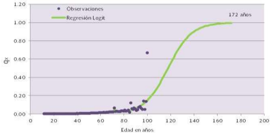
Figura 2.7.1 Modelo logit aplicado a los datos base de mortalidad mexicana 2000-I.
