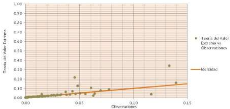
Figura 3.1.2 Teoría de extremos (GPD) vs observaciones aplicada a los datos base de mortalidad mexicana CNSF-2000-I
