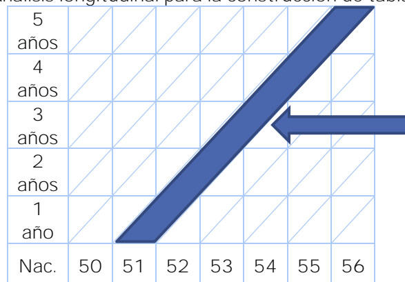
Figura 1.1 Análisis longitudinal para la construcción de tablas de mortalidad.
