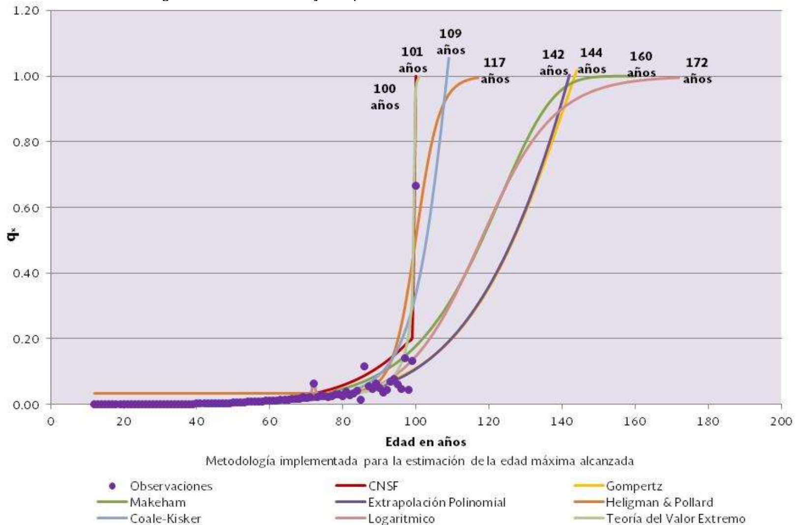
Figura 4.1 Modelos de ajuste para la mortalidad mexicana CNSF-2000-I.
