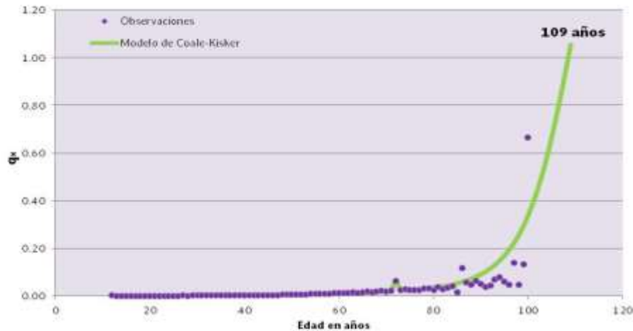
Figura 2.6.1 Modelo de Coale-Kisker aplicado a los datos base de mortalidad mexicana 2000-I.
