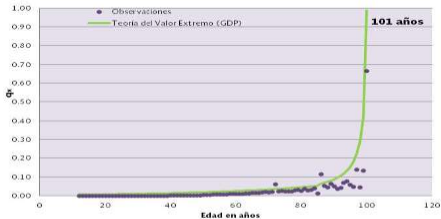
Figura 5.1 Teoría de extremos aplicada a los datos base de mortalidad mexicana CNSF-2000-I
