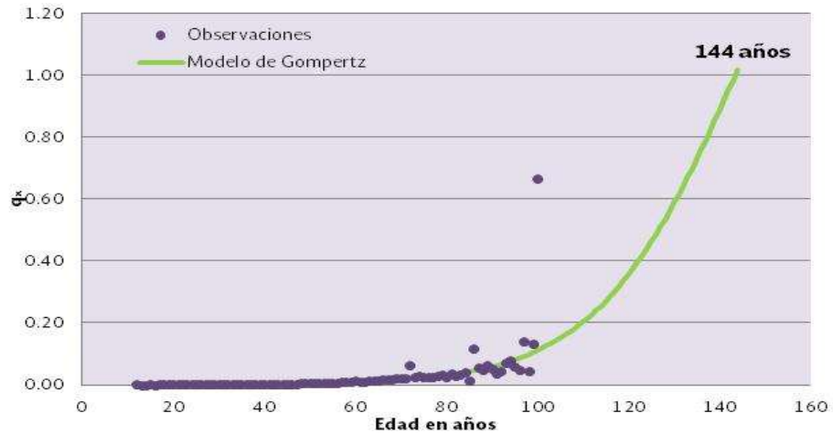
Figura 2.3.2 Modelo de Gompertz aplicado a los datos base de mortalidad mexicana 2000-I.
