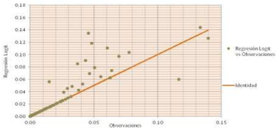
Figura 2.7.2 Cuantil-Cuantil regresión logit (CNSF) vs observaciones aplicado a la mortalidad mexicana 2000-I.
