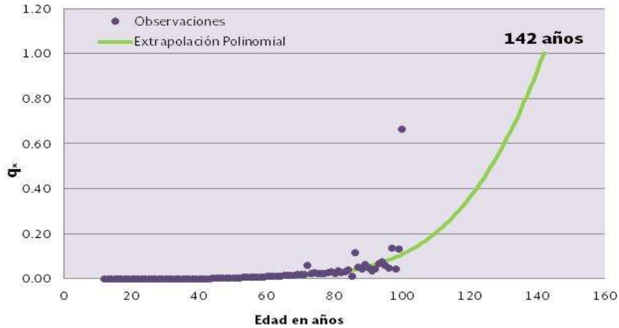
Figura 2.2.1 Método de extrapolación polinomial aplicado a los datos base de mortalidad mexicana 2000-I.
