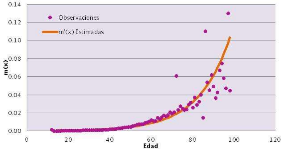
Figura 2.3.1 Ajuste de parámetros estimados para m_x para el modelo de Gompertz de los datos base de la población mexicana 2000-I.
