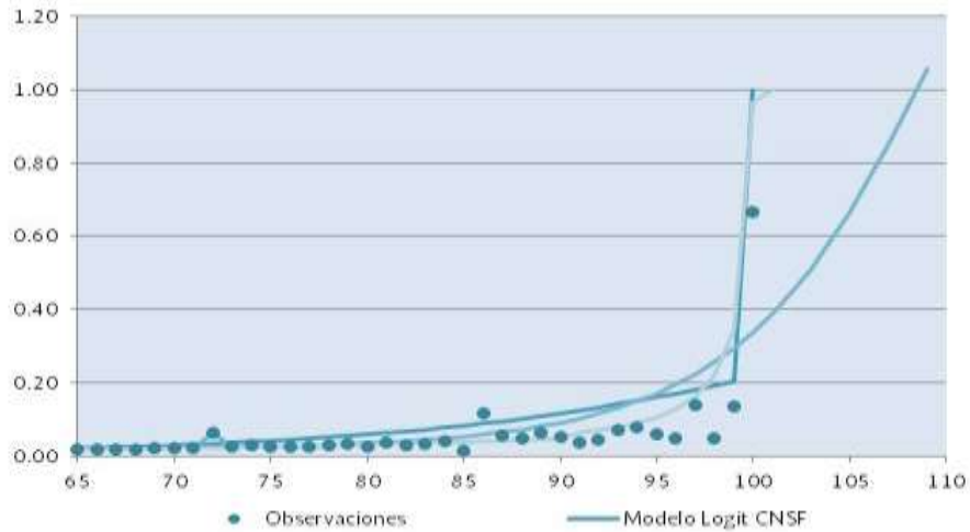
Figura 4.2 Análisis de probabilidades de fallecimiento observadas vs modelo de Coale-Kisker, logit CNSF y teoría de extremos (GPD).
