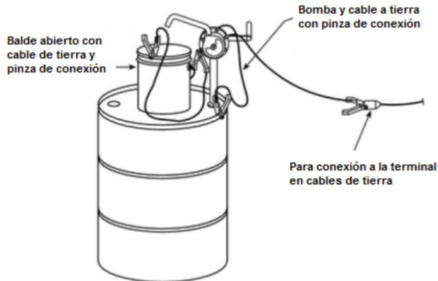
Figura I.2 â Ejemplo de algunas formas para proveer conexión equipotencial y conexión a tierra.
