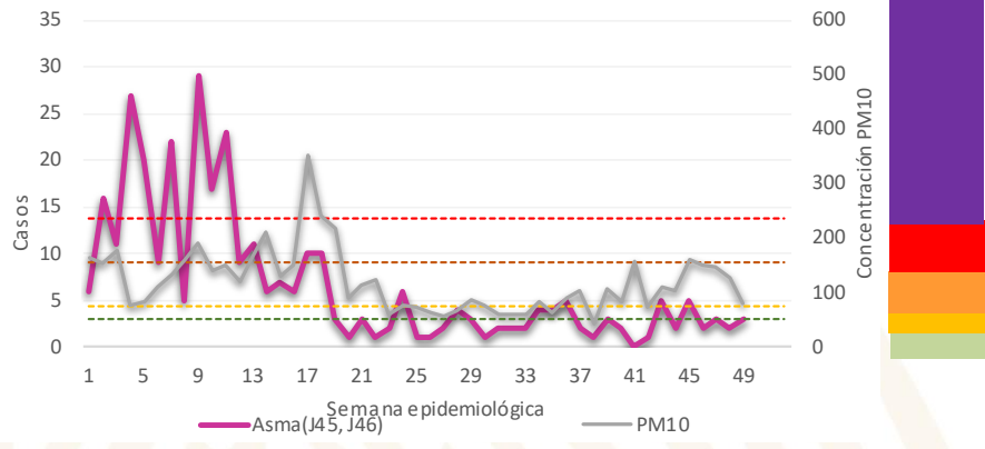
Casos de Asma y niveles máximos de PM10 por semana epidemiológica. Región Sureste – ZMVM, 2020
