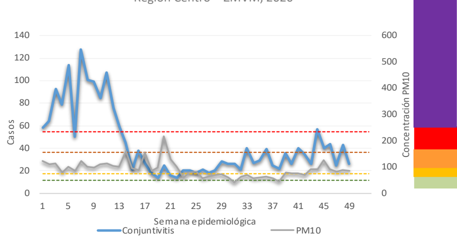
Casos de Conjuntivitis y niveles máximos de PM10 por semana epidemiológica. Región Centro – ZMVM, 2020
