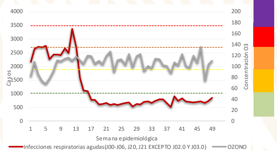
Casos de Infecciones Respiratorias Agudas (IRA) y niveles máximos de ozono por semana epidemiológica. Región Suroeste – ZMVM, 2020
