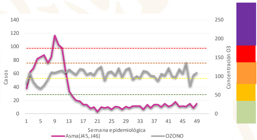
Casos de Asma y niveles máximos de ozono por semana epidemiológica. Región Suroeste – ZMVM, 2020
