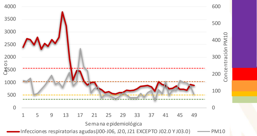
Casos de Infecciones Respiratorias Agudas (IRA) y niveles máximos de PM10 por semana epidemiológica. Región Sureste – ZMVM, 2020
