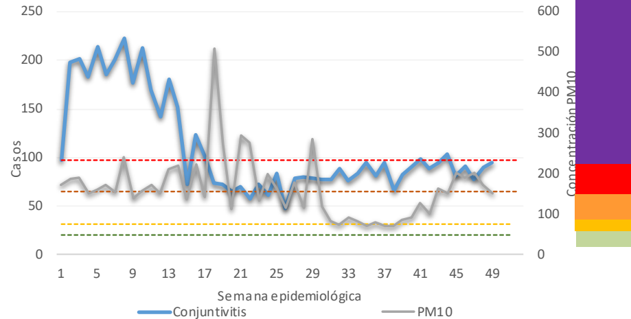
Casos de Conjuntivitis y niveles máximos de PM10 por semana epidemiológica. Región Noreste – ZMVM, 2020
