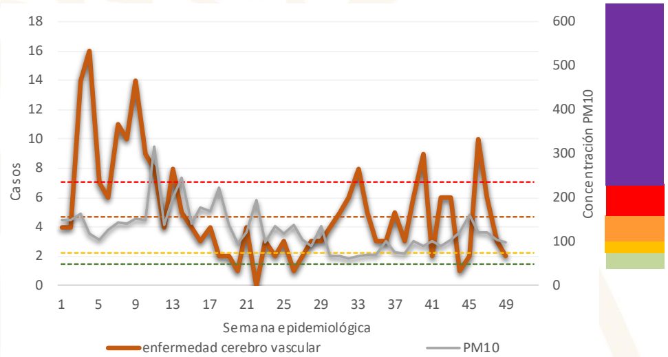
Casos de Enfermedad Cerebro Vascular y niveles máximos de PM10 por semana epidemiológica. Región Noroeste – ZMVM, 2020
