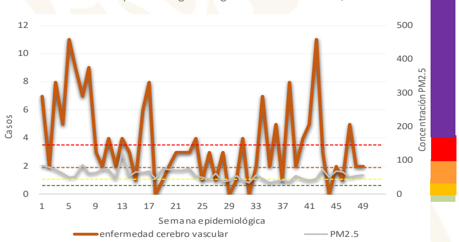
Casos de Enfermedad Cerebro Vascular y niveles máximos de PM2.5 por semana epidemiológica. Región Noreste – ZMVM, 2020
