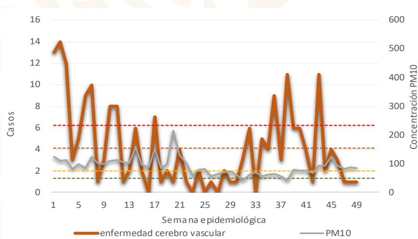
Casos de Enfermedad Cerebro Vascular y niveles máximos de PM10 por semana epidemiológica. Región Centro – ZMVM, 2020
