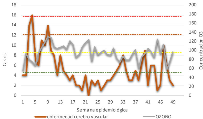
Casos de Enfermedad Cerebro Vascular y niveles máximos de ozono por semana epidemiológica. Región Noroeste – ZMVM, 2020
