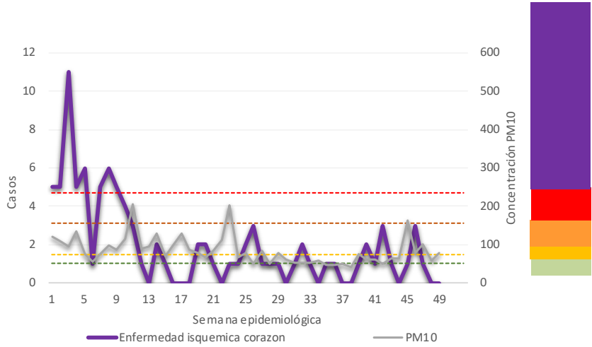
Casos de Enfermedad Isquémica del Corazón y niveles máximos de PM10 por semana epidemiológica. Región Suroeste– ZMVM, 2020
