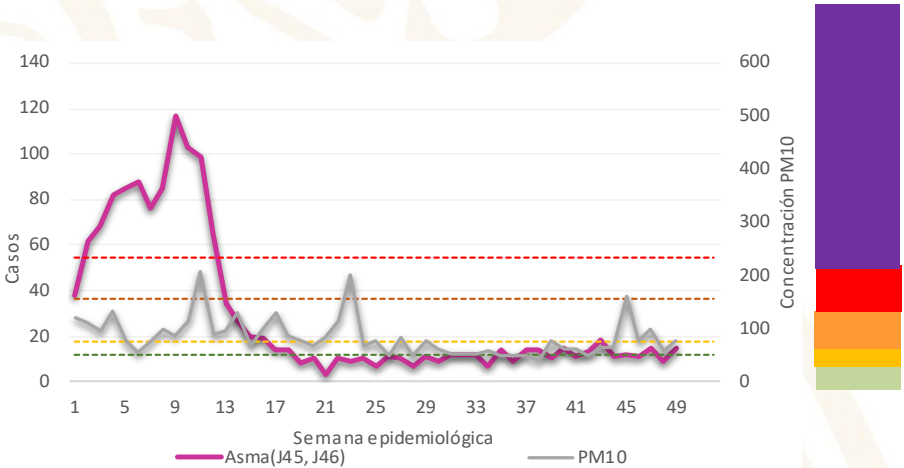
Casos de Asma y niveles máximos de PM10 por semana epidemiológica. Región Suroeste – ZMVM, 2020
