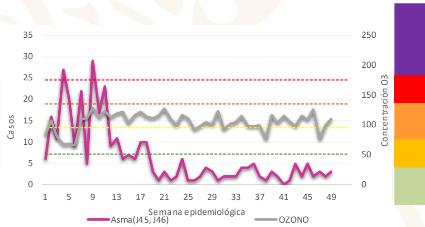
Casos de Asma y niveles máximos de ozono por semana epidemiológica. Región Sureste – ZMVM, 2020
