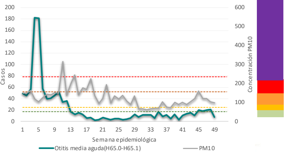
Casos de Otitis Media Aguda y niveles máximos de PM10 por semana epidemiológica. Región Noroeste – ZMVM, 2020
