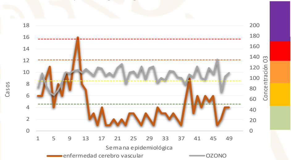
Casos de Enfermedad Cerebro Vascular y niveles máximos de ozono por semana epidemiológica. Región Suroeste – ZMVM, 2020
