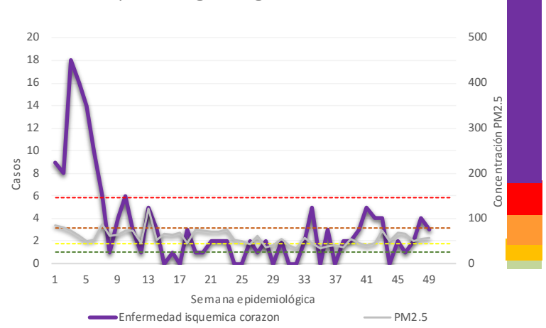
Casos de Enfermedad Isquémica del Corazón y niveles máximos de PM2.5 por semana epidemiológica. Región Noreste– ZMVM, 2020
