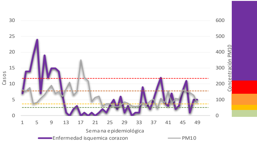
Casos de Enfermedad Isquémica del Corazón y niveles máximos de PM10 por semana epidemiológica. Región Sureste– ZMVM, 2020
