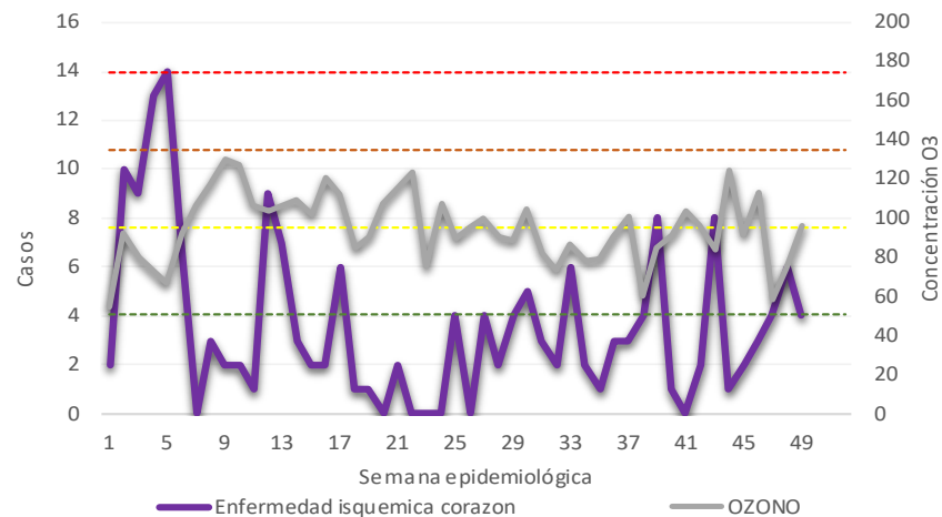
Casos de Enfermedad Isquémica del Corazón y niveles máximos de ozono por semana epidemiológica. Región Noroeste – ZMVM, 2020
