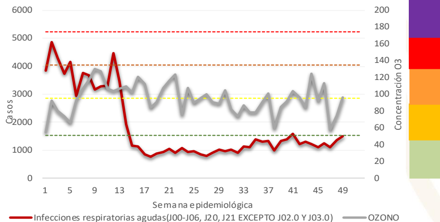
Casos de Infecciones Respiratorias Agudas (IRA) y niveles máximos de ozono por semana epidemiológica. Región Noroeste – ZMVM, 2020
