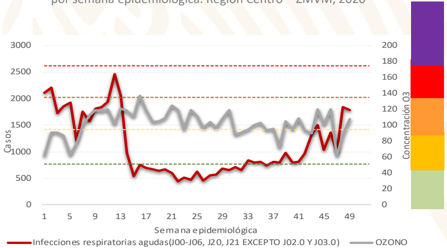
Casos de Infecciones Respiratorias Agudas (IRA) y niveles máximos de ozono por semana epidemiológica. Región Centro – ZMVM, 2020
