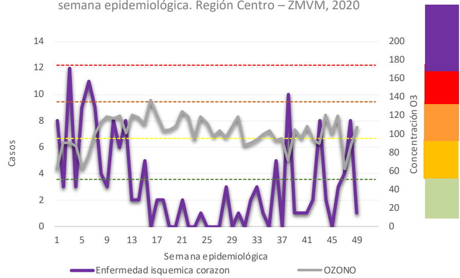
Casos de Enfermedad Isquémica del Corazón y niveles máximos de ozono por semana epidemiológica. Región Centro – ZMVM, 2020
