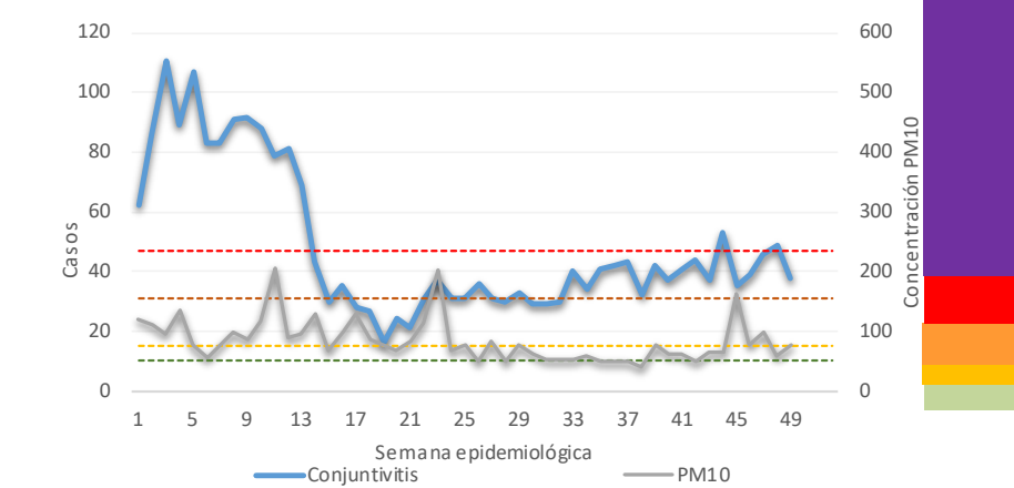
Casos de Conjuntivitis y niveles máximos de PM10 por semana epidemiológica. Región Suroeste – ZMVM, 2020
