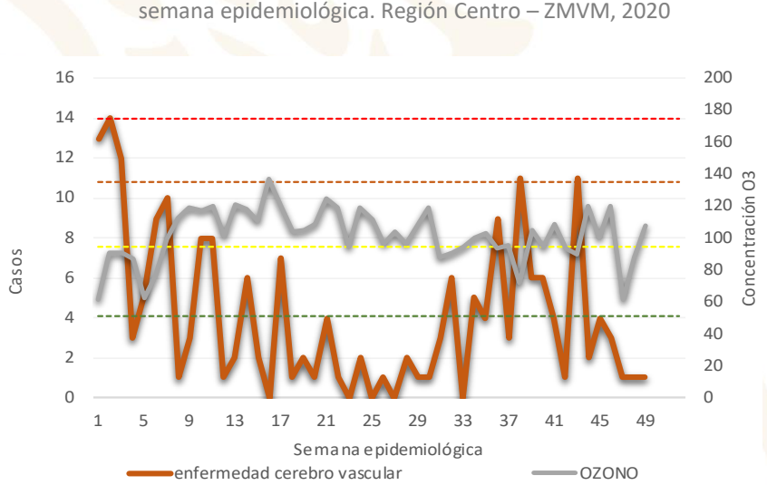
Casos de Enfermedad Cerebro Vascular y niveles máximos de ozono por semana epidemiológica. Región Centro – ZMVM, 2020
