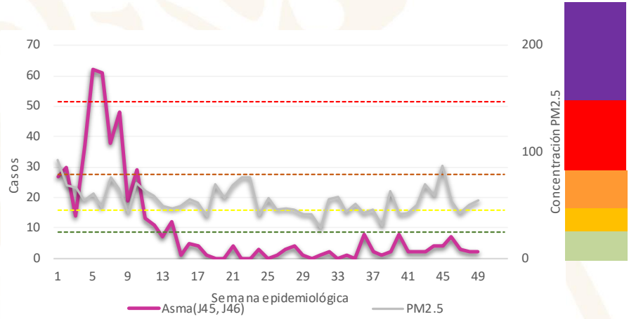
Casos de Asma y niveles máximos de PM2.5 por semana epidemiológica. Región Centro – ZMVM, 2020
