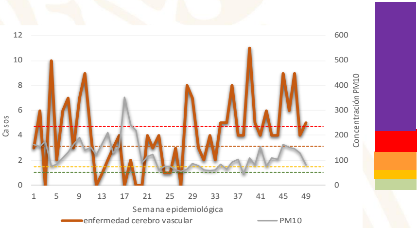
Casos de Enfermedad Cerebro Vascular y niveles máximos de PM10 por semana epidemiológica. Región Sureste – ZMVM, 2020
