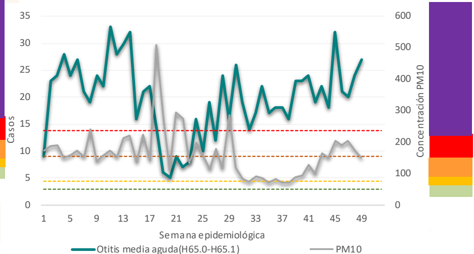
Casos de Otitis Media Aguda y niveles máximos de PM10 por semana epidemiológica. Región Noreste – ZMVM, 2020
