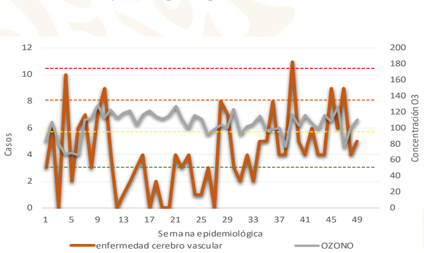
Casos de Enfermedad Cerebro Vascular y niveles máximos de ozono por semana epidemiológica. Región Sureste – ZMVM, 2020
