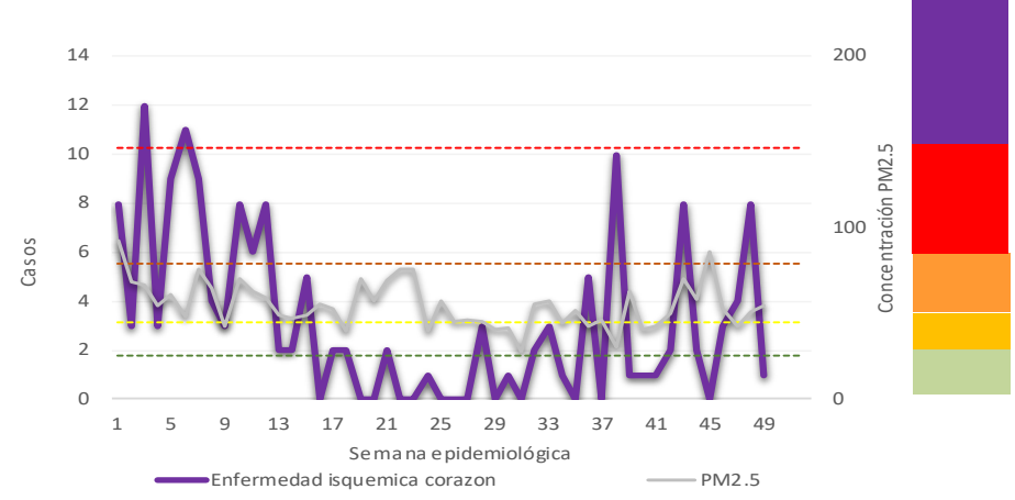
Casos de Enfermedad Isquémica del Corazón y niveles máximos de PM2.5 por semana epidemiológica. Región Centro – ZMVM, 2020
