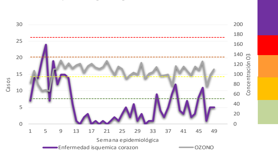
Casos de Enfermedad Isquémica del Corazón y niveles máximos de ozono por semana epidemiológica. Región Sureste – ZMVM, 2020
