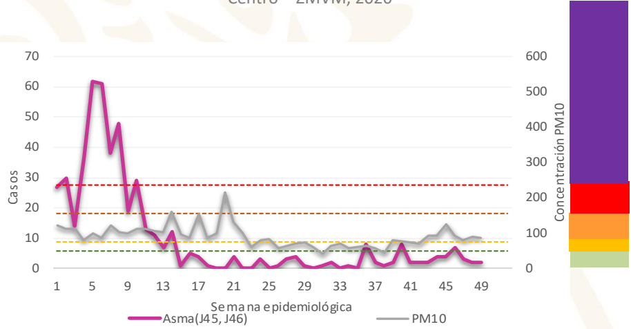
Casos de Asma y niveles máximos de PM10 por semana epidemiológica. Región Centro – ZMVM, 2020
