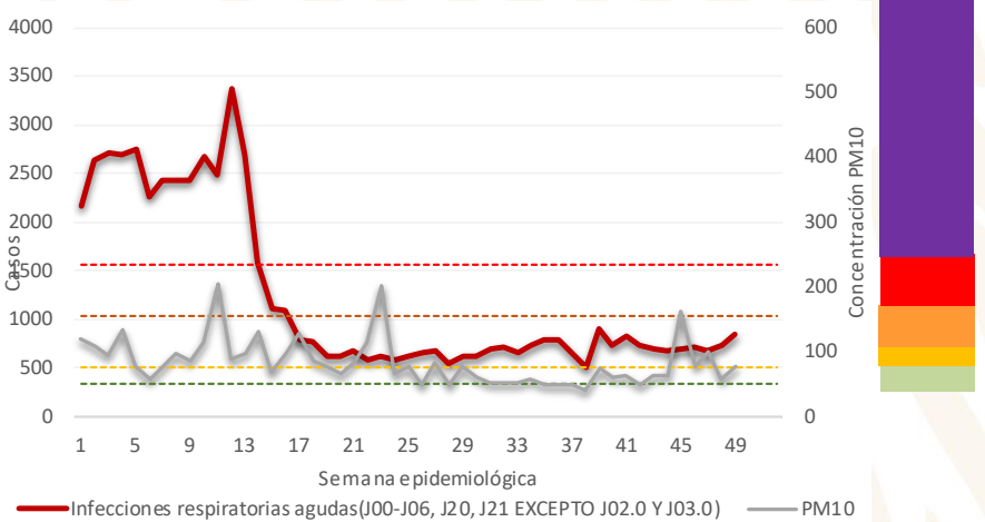
Casos de Infecciones Respiratorias Agudas (IRA) y niveles máximos de PM10 por semana epidemiológica. Región Suroeste – ZMVM, 2020
