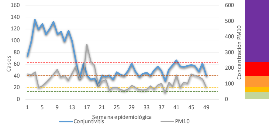
Casos de Conjuntivitis y niveles máximos de PM10 por semana epidemiológica. Región Sureste – ZMVM, 2020
