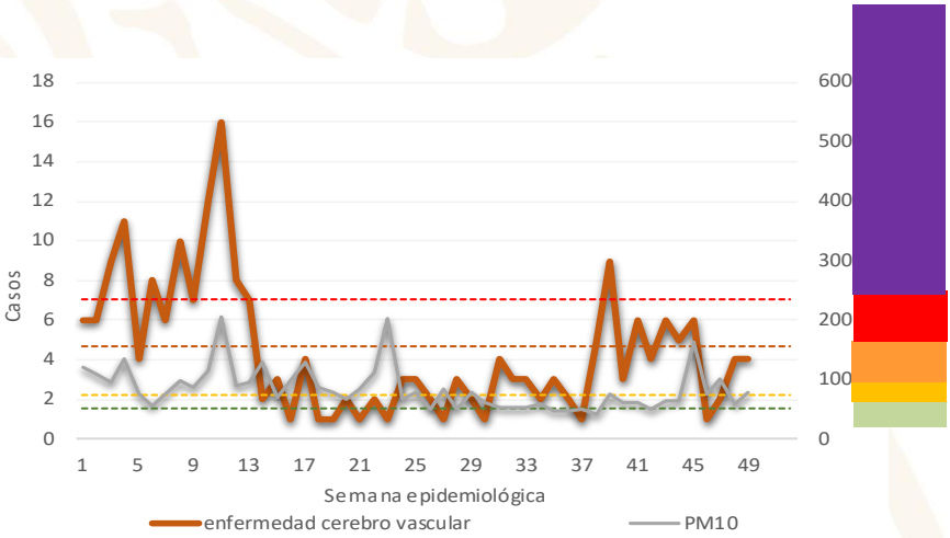
Casos de Enfermedad Cerebro Vascular y niveles máximos de PM10 por semana epidemiológica. Región Suroeste– ZMVM, 2020
