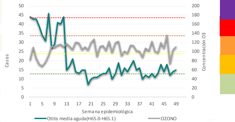
Casos de Otitis Media Aguda y niveles máximos de ozono por semana epidemiológica. Región Suroeste – ZMVM, 2020
