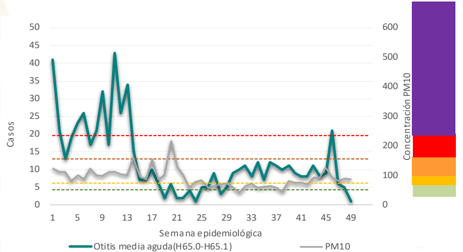
Casos de Otitis Media Aguda y niveles máximos de PM10 por semana epidemiológica. Región Centro – ZMVM, 2020
