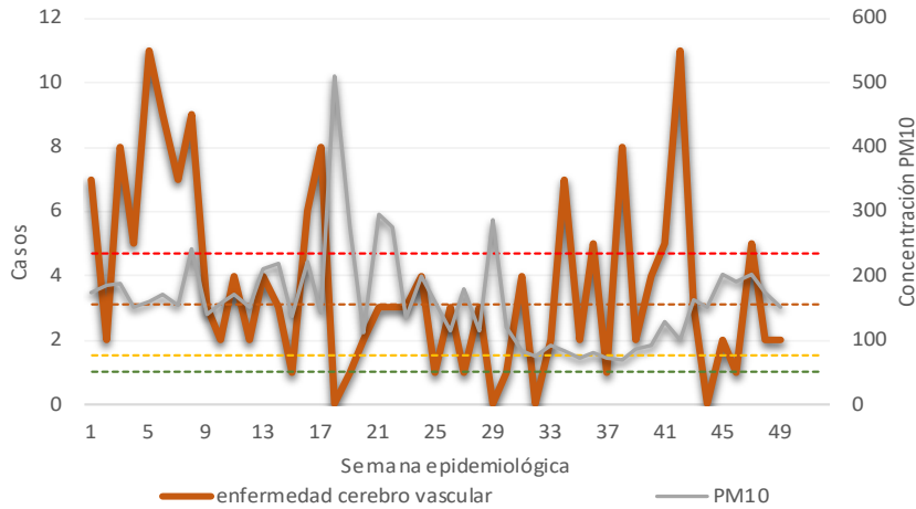
Casos de Enfermedad Cerebro Vascular y niveles máximos de PM10 por semana epidemiológica. Región Noreste – ZMVM, 2020
