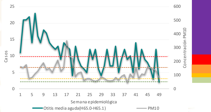
Casos de Otitis Media Aguda y niveles máximos de PM10 por semana epidemiológica. Región Sureste – ZMVM, 2020
