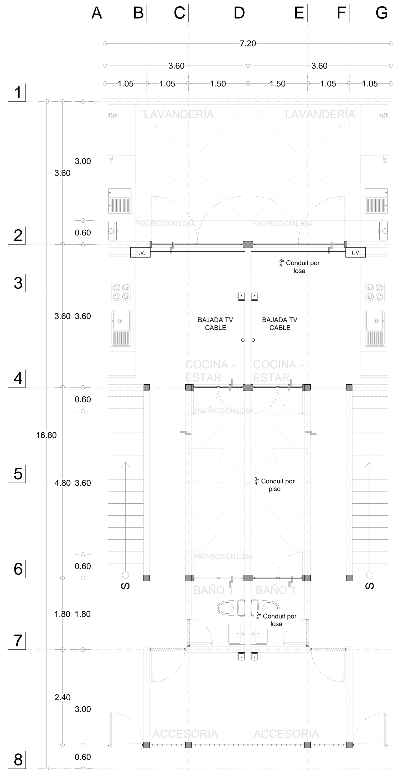
INS. VOZ Y DATOS PLANTA BAJA 1:50
