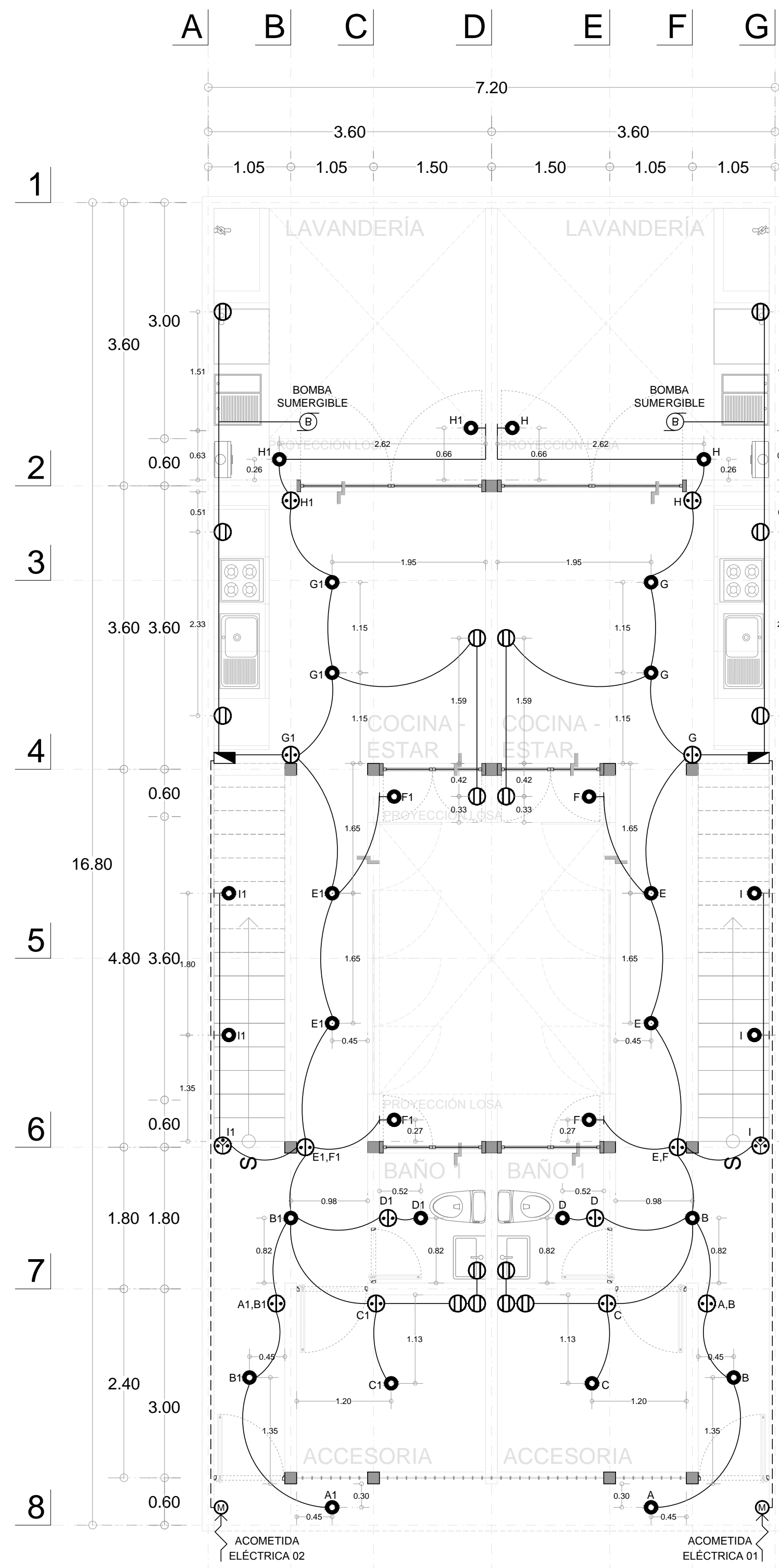
INS. ELÉCTRICA PLANTA BAJA 1:50
