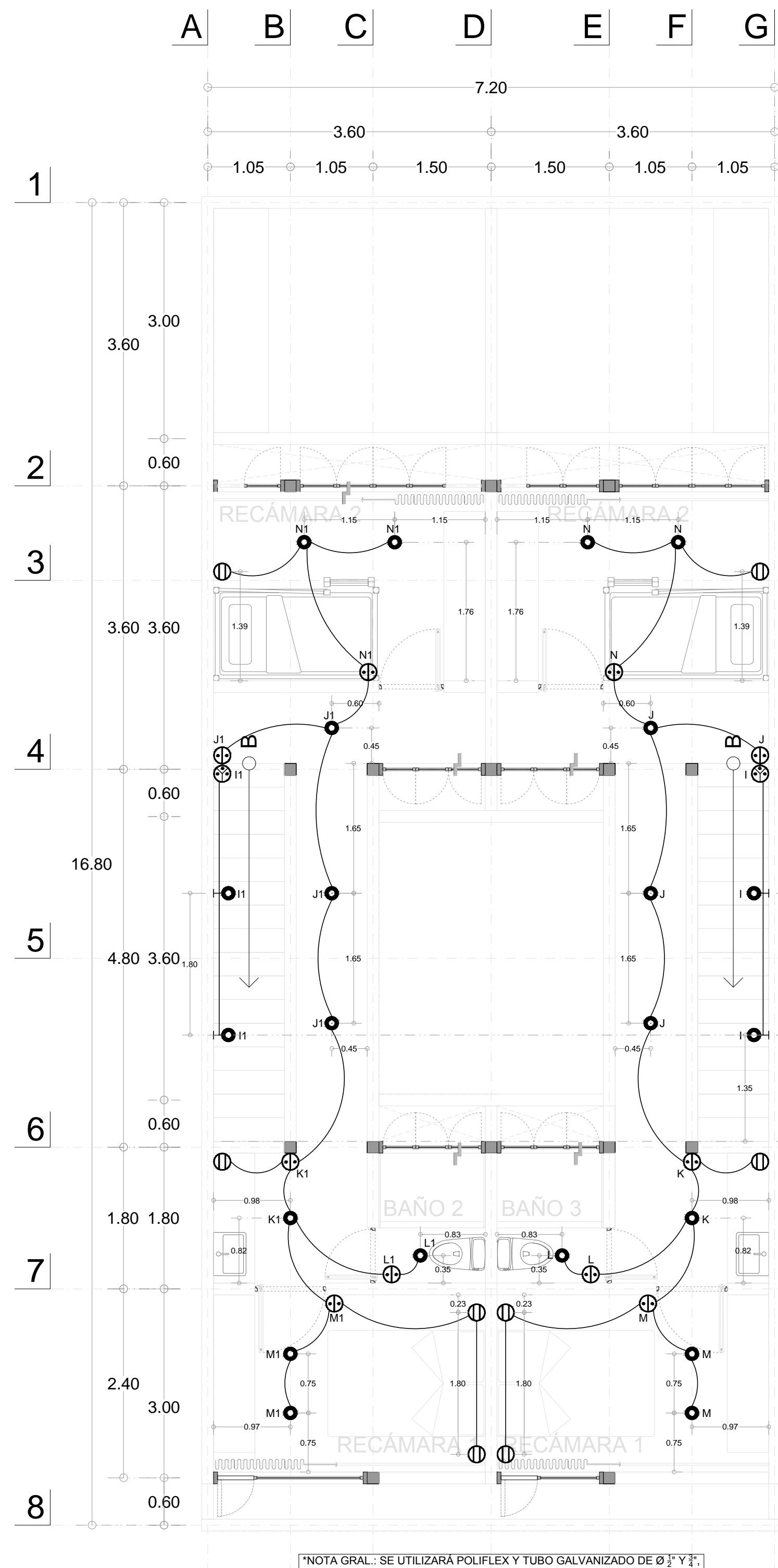
INS. ELÉCTRICA PLANTA ALTA 1:50
