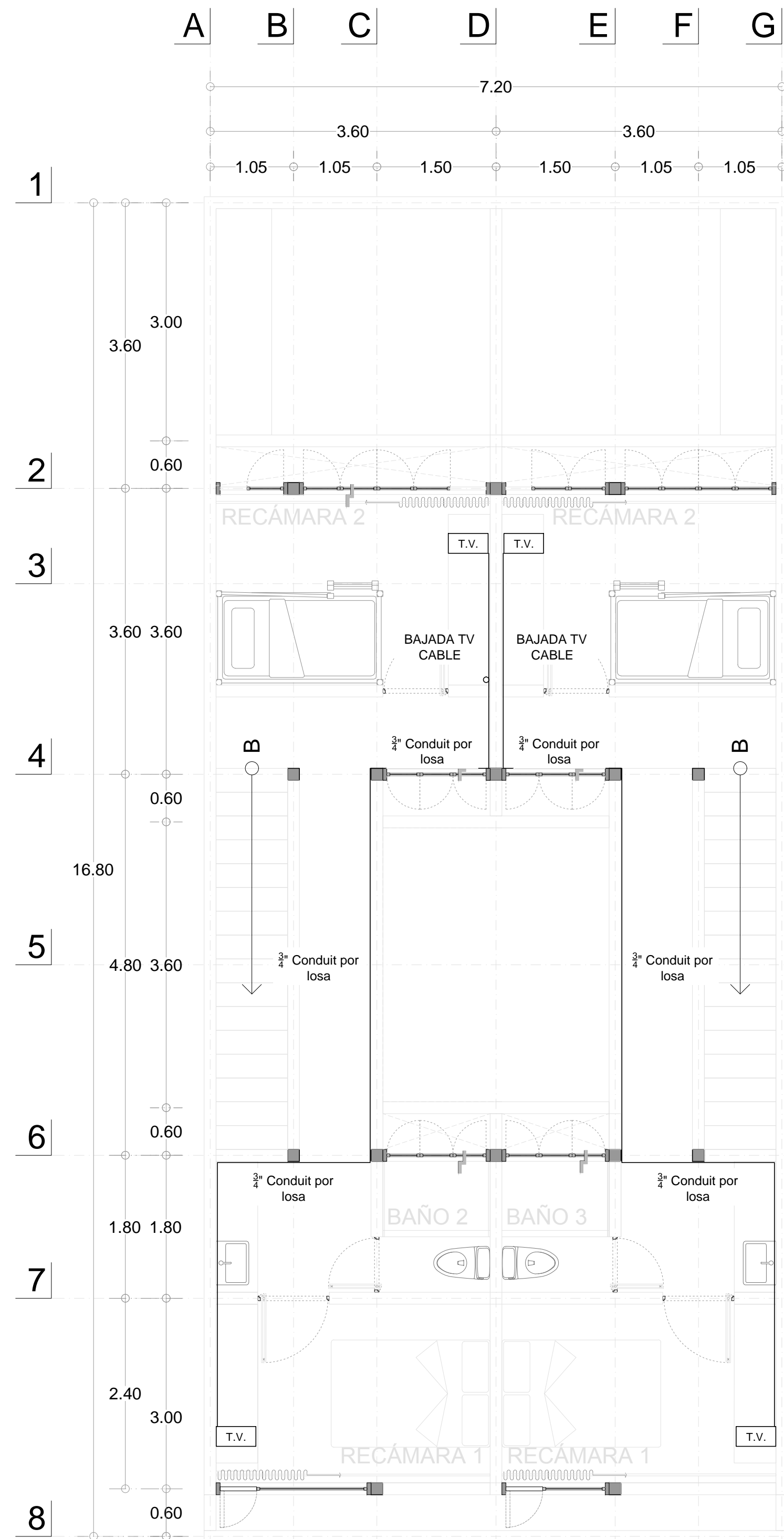
INS. VOZ Y DATOS PLANTA ALTA 1:50
