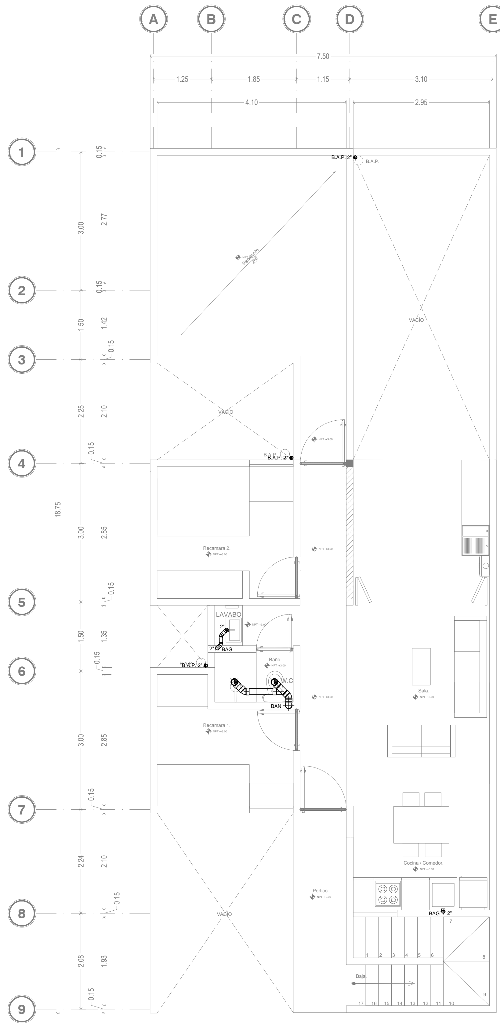
INS. SANITARIA PLANTA ALTA ESC. 1:50
