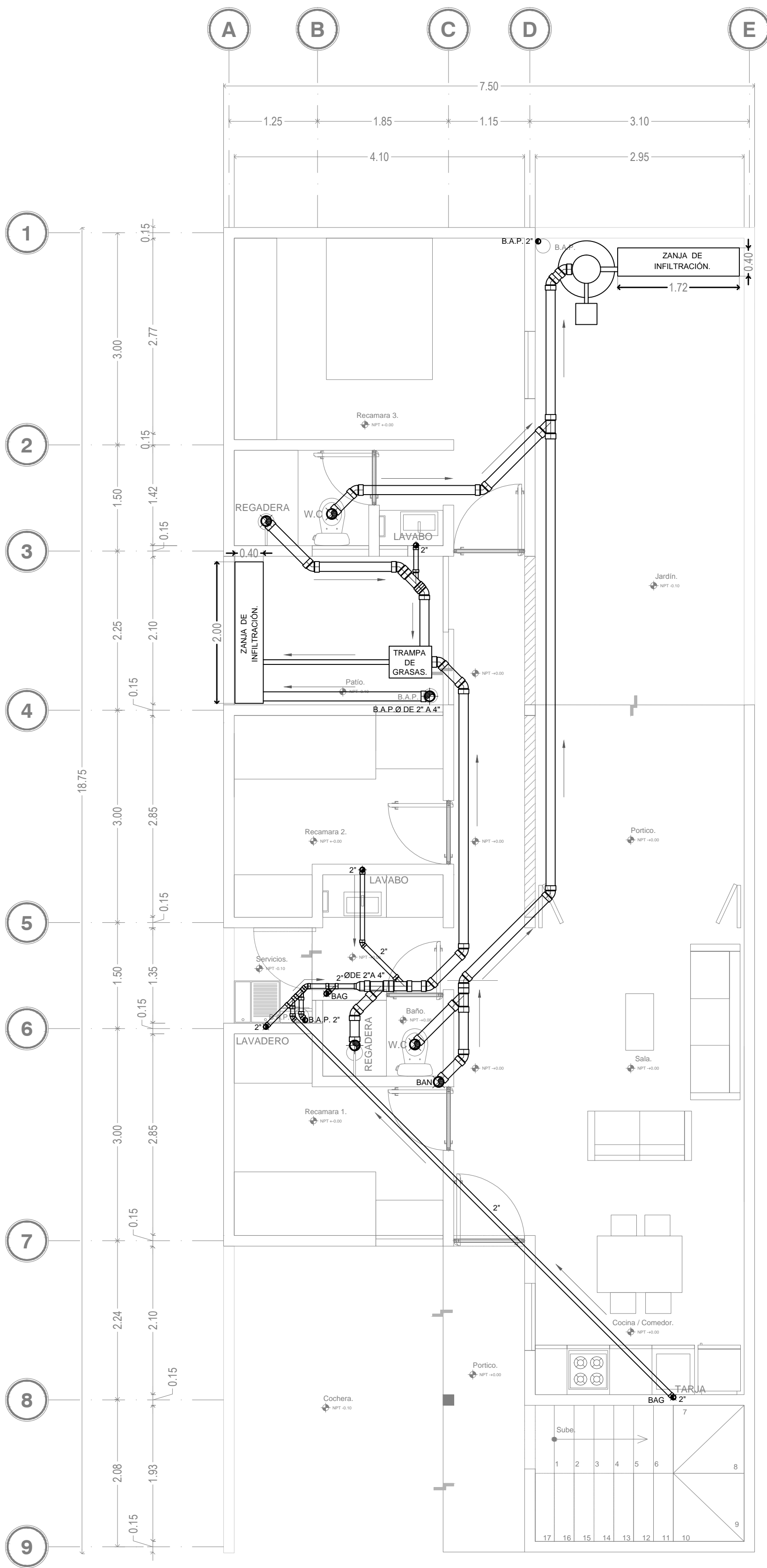
INS. SANITARIA PLANTA BAJA ESC. 1:50
