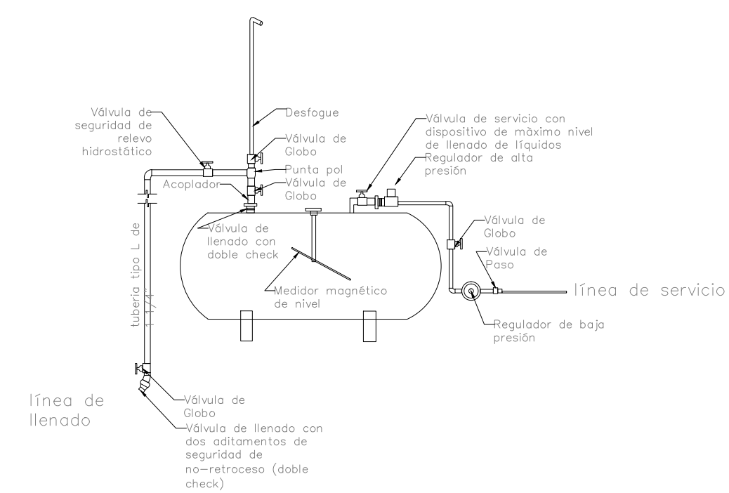
INS. GAS PLANTA ALTA ESC. 1:50
