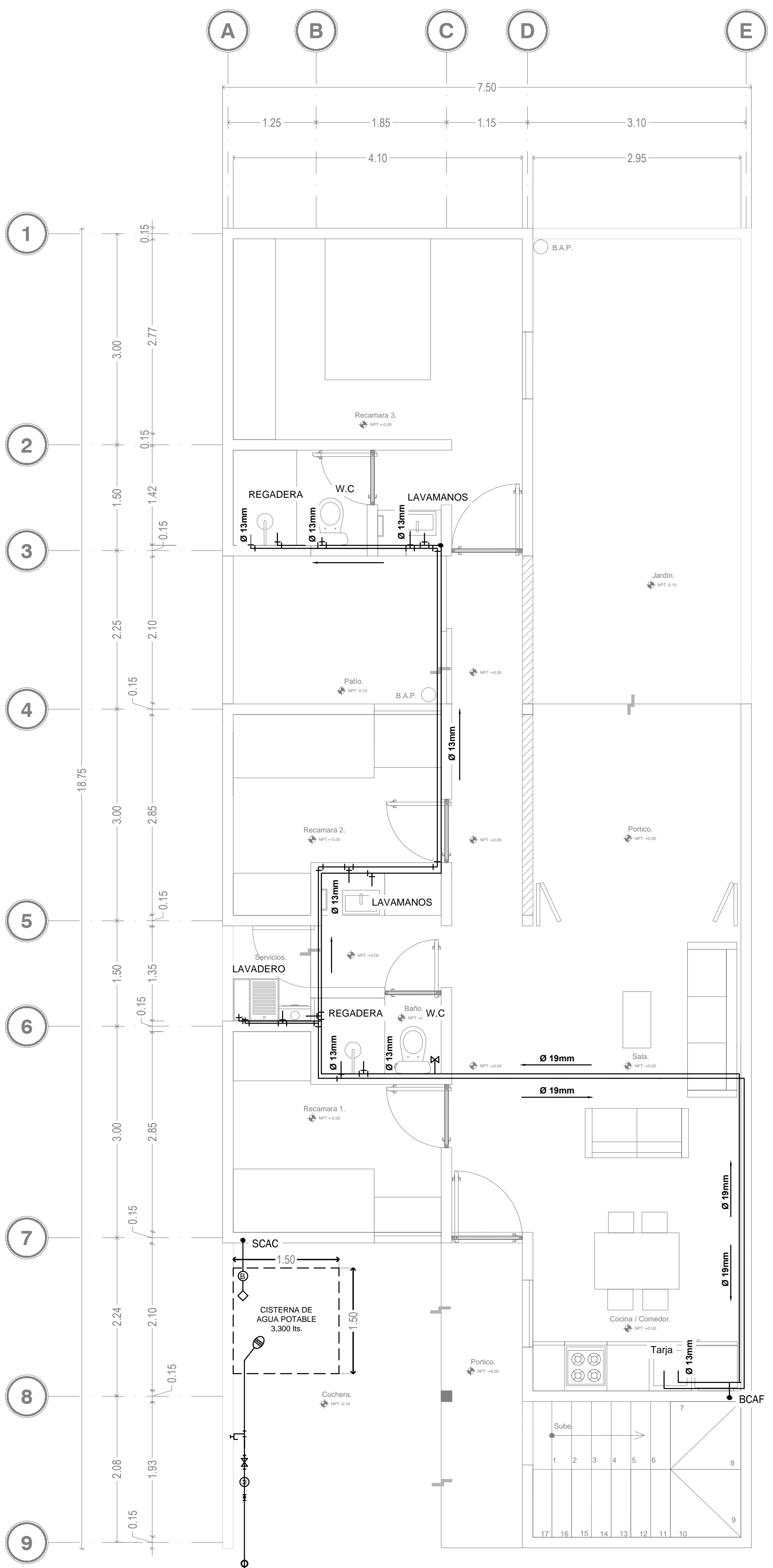
INS. HIDRÁULICA PLANTA BAJA ESC. 1:50
