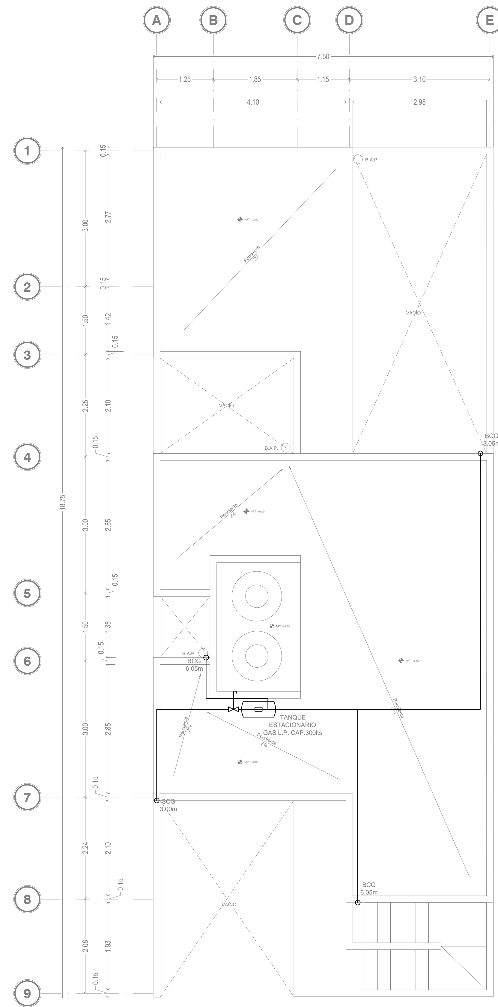
INS. GAS PLANTA DE AZOTEA ESC. 1:50
