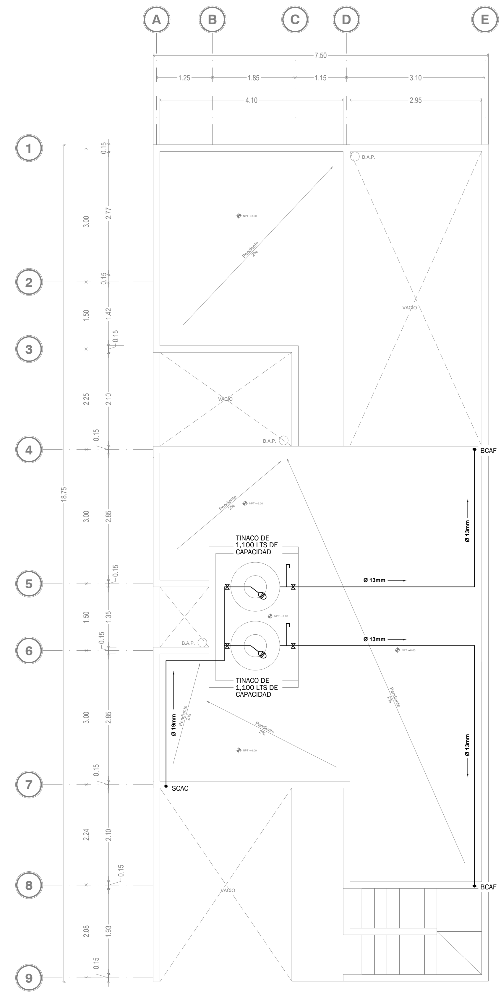
INS. HIDRÁULICA PLANTA DE AZOTEA ESC. 1:50
