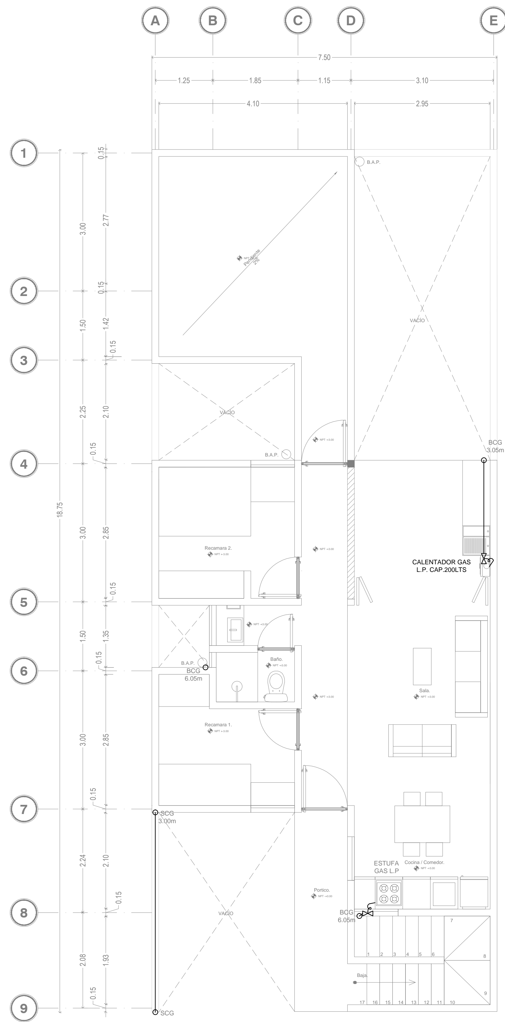
INS. GAS PLANTA ALTA ESC. 1:50
