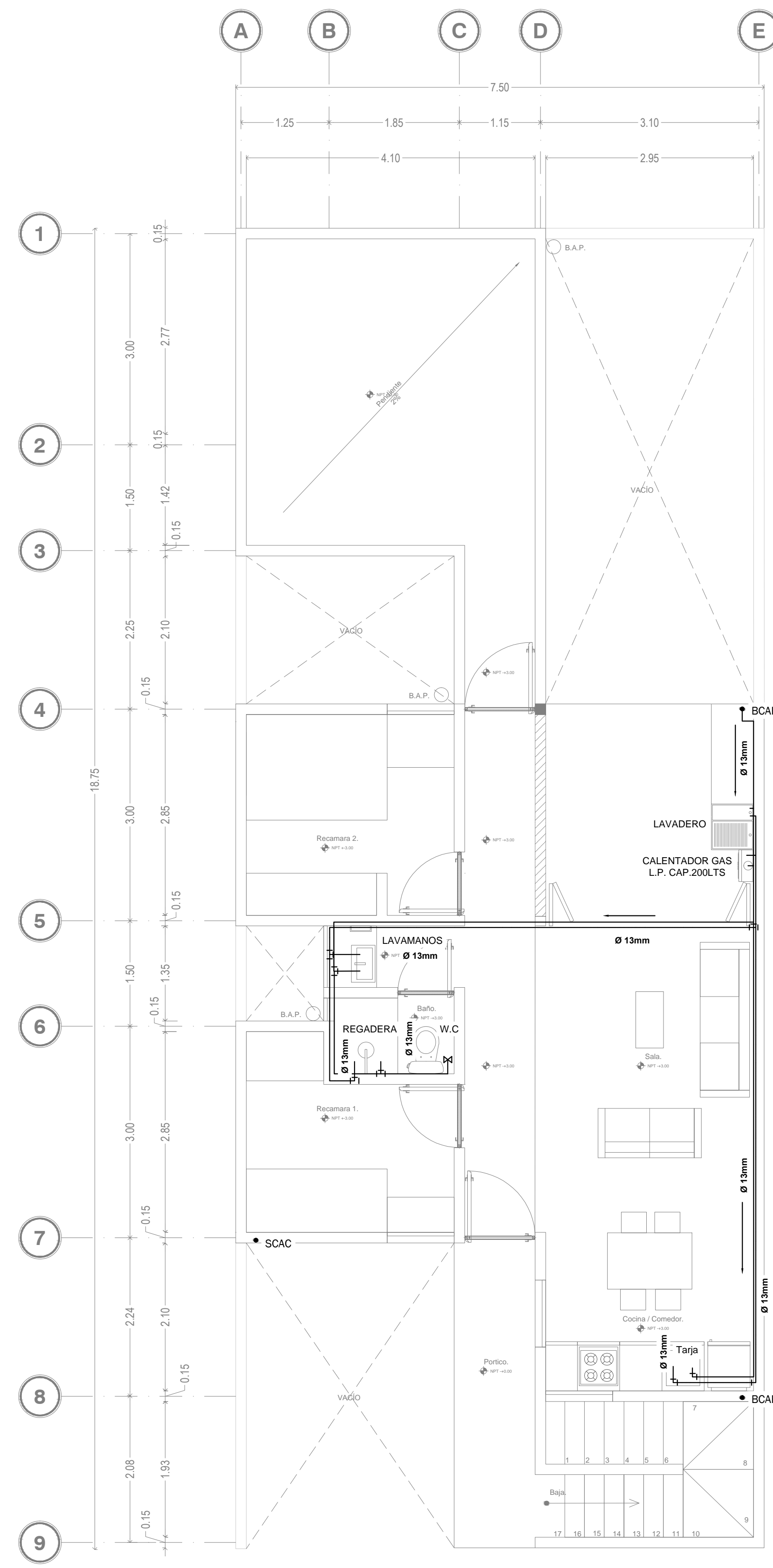
INS. HIDRÁULICA PLANTA ALTA ESC. 1:50
