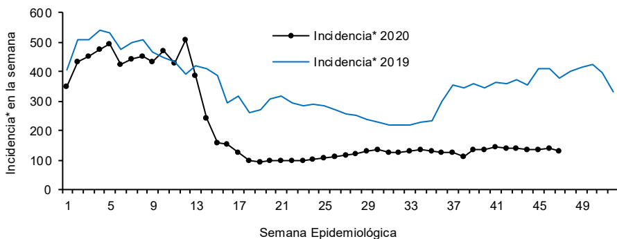
Gráfica 3. Incidencia de IRA durante la semana epidemiológica 47, México 2020.
