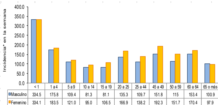
Gráfica 3. Incidencia de IRA durante la semana epidemiológica 47, México 2020.
