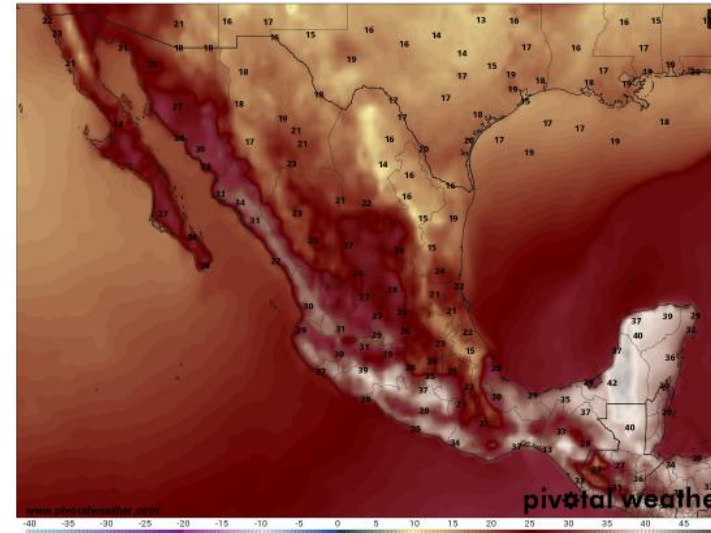
Imagen de referencia 1: Pronóstico de temperatura para el miércoles 15 a las 13:00 h (hora del centro).
