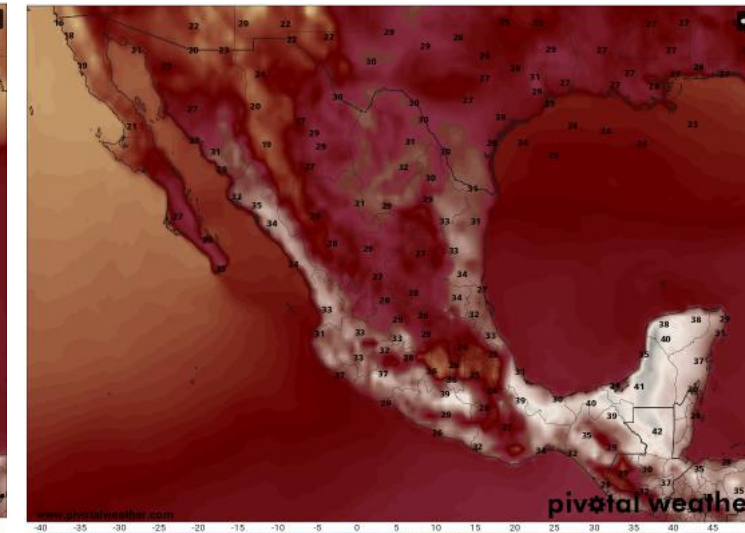
Imagen de referencia 2: Pronóstico de temperatura para el martes 21 a las 13:00 h (hora del centro).
