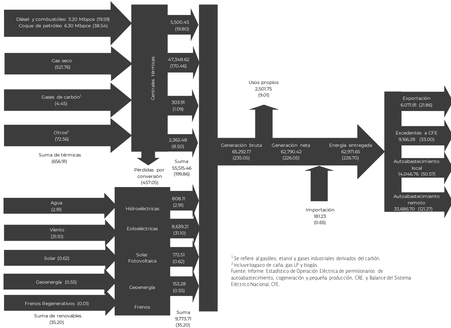
Diagrama 16. Balance de electricidad autoabastecedores 2017, GWh (Petajoules)
