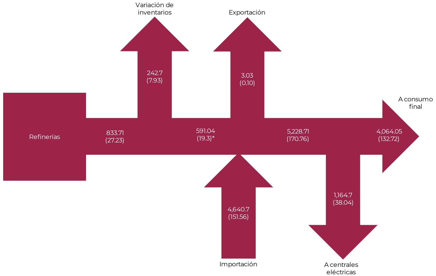
Diagrama 7. Balance de coque de petróleo 2018, miles de toneladas (Petajoules)
