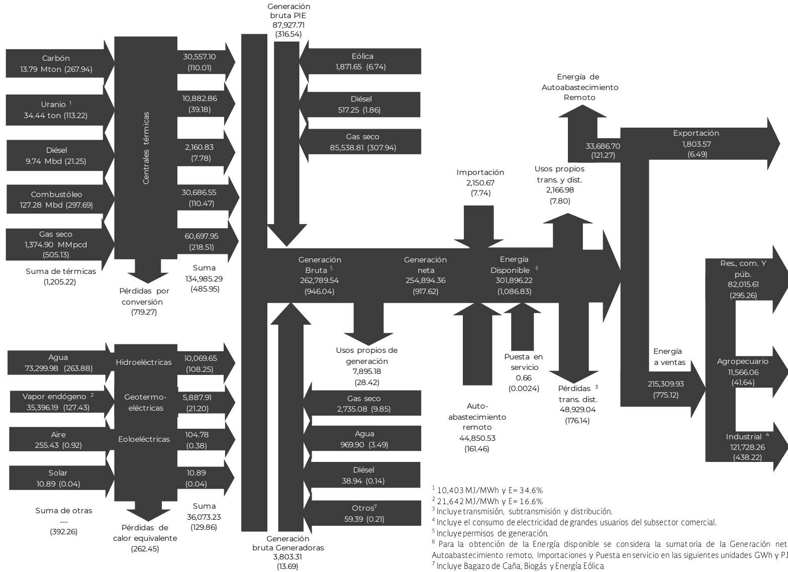
Diagrama 14. Balance de electricidad servicio público 2017, GWh (Petajoules)
