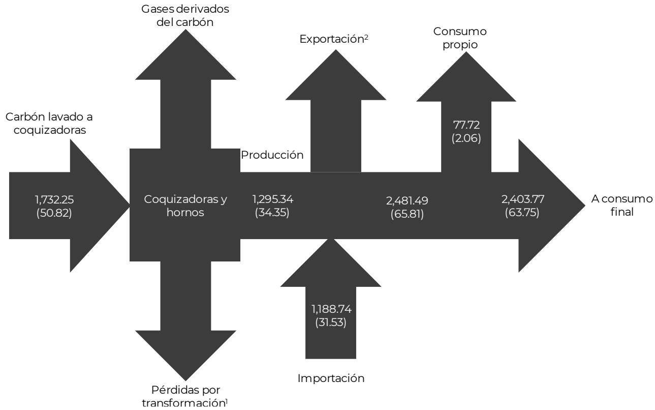
Diagrama 6. Balance de coque de carbón 2017, miles de toneladas (Petajoules)
