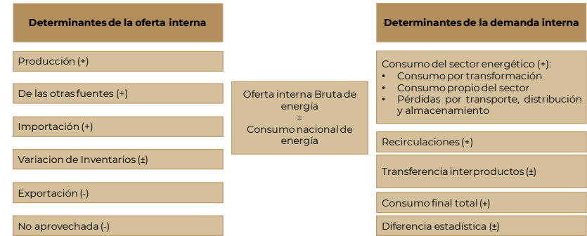
Esquema 1. Flujo de la oferta interna bruta o consumo nacional de energía
