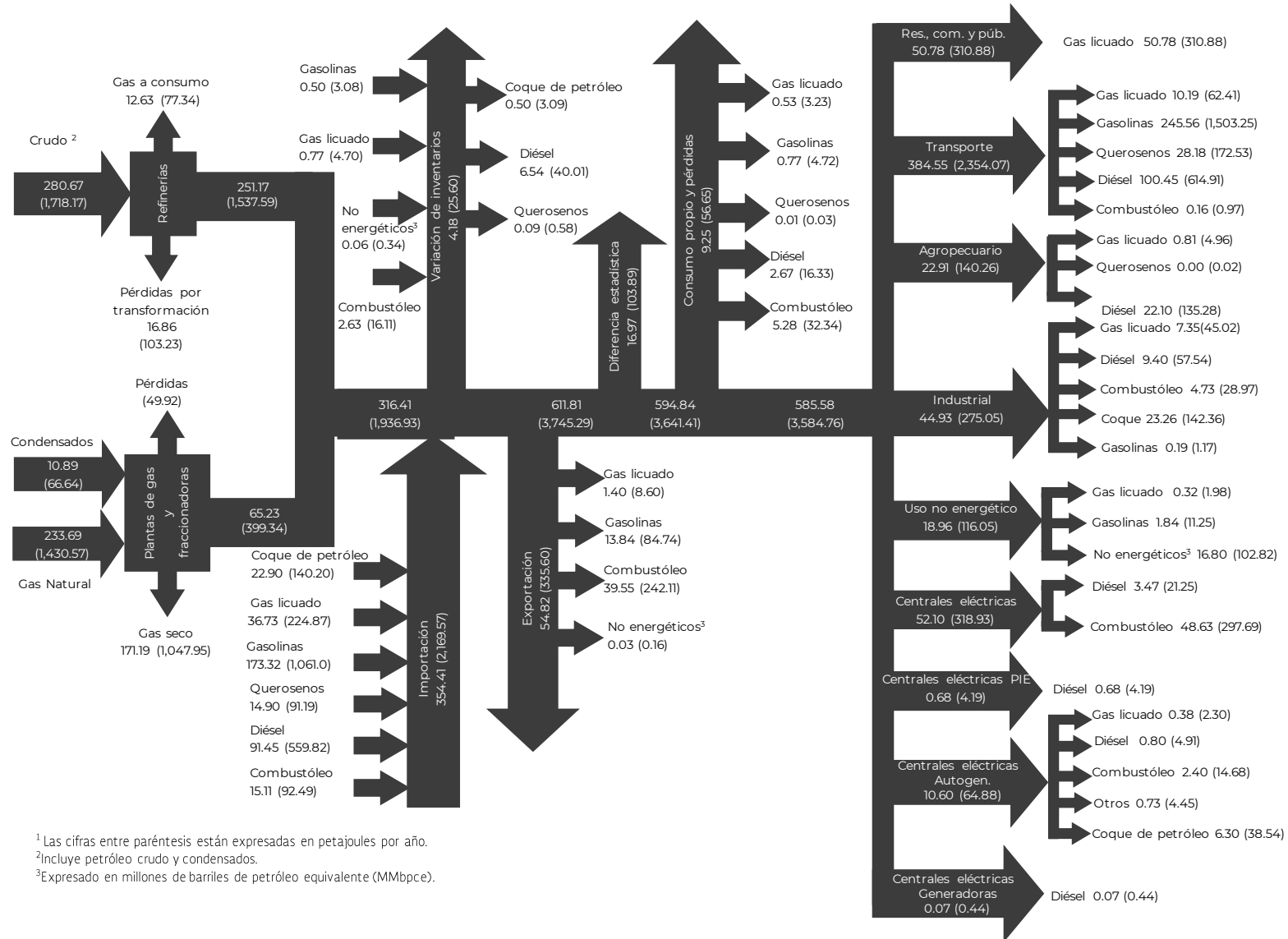
Diagrama 12. Balance de petrolíferos 2017, miles de barriles de petróleo equivalente diarios (Petajoules).
