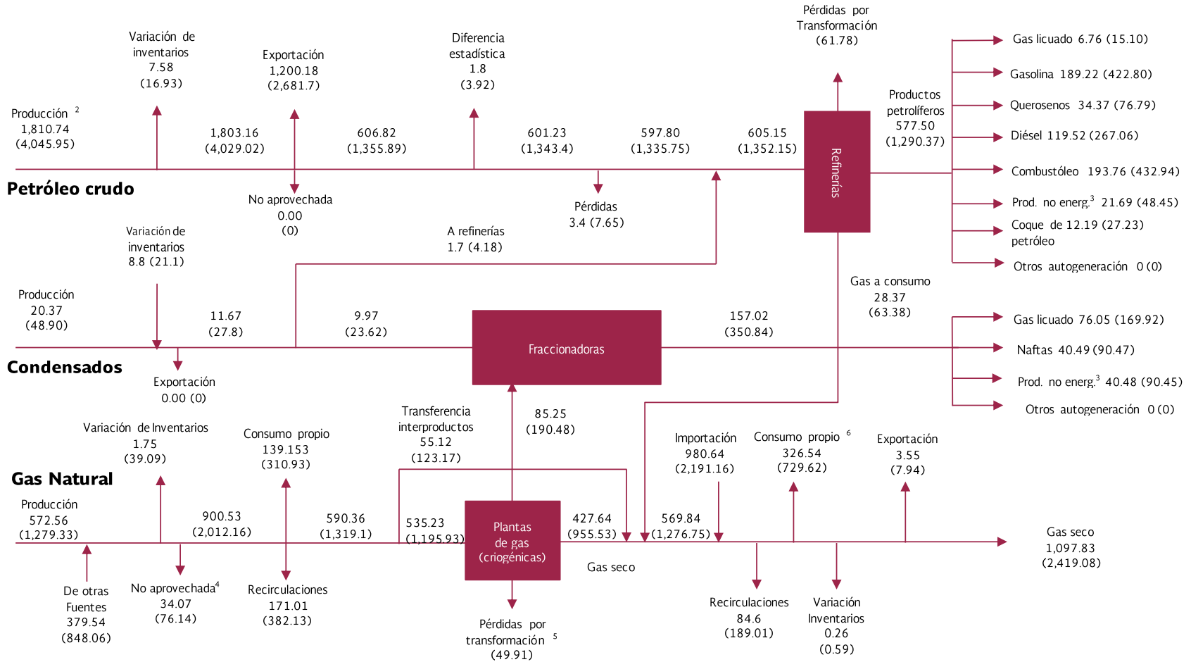
Diagrama 9. Balance de energía de hidrocarburos 2018, miles de barriles diarios (Petajoules)
