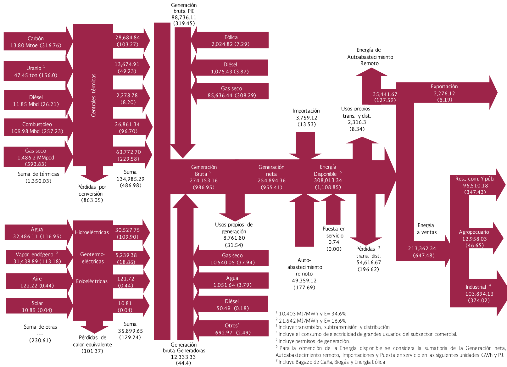
Diagrama 13. Balance de electricidad servicio público 2018, GWh (Petajoules).
