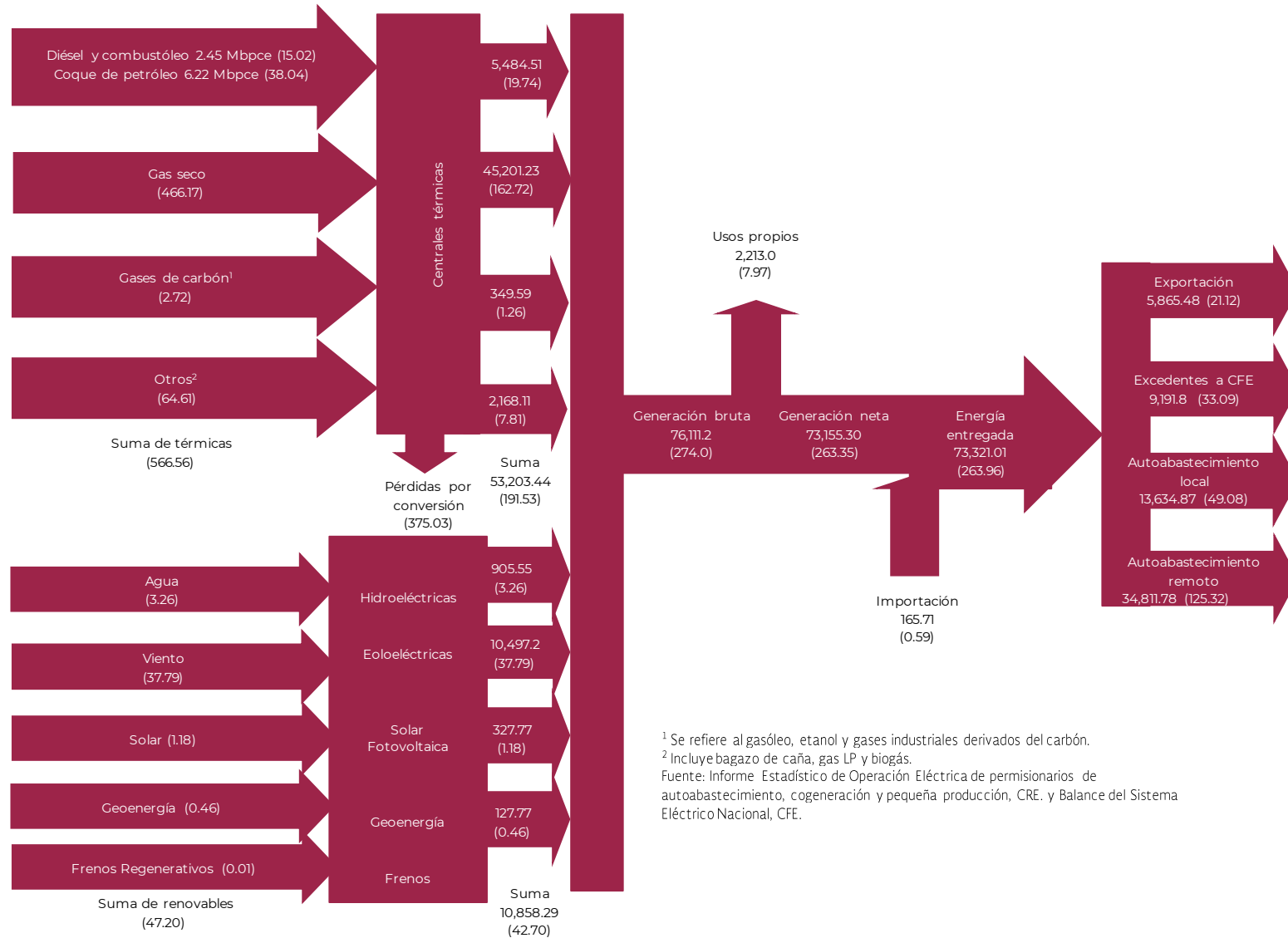
Diagrama 15. Balance de electricidad autoabastecedores 2018, GWh (Petajoules)
