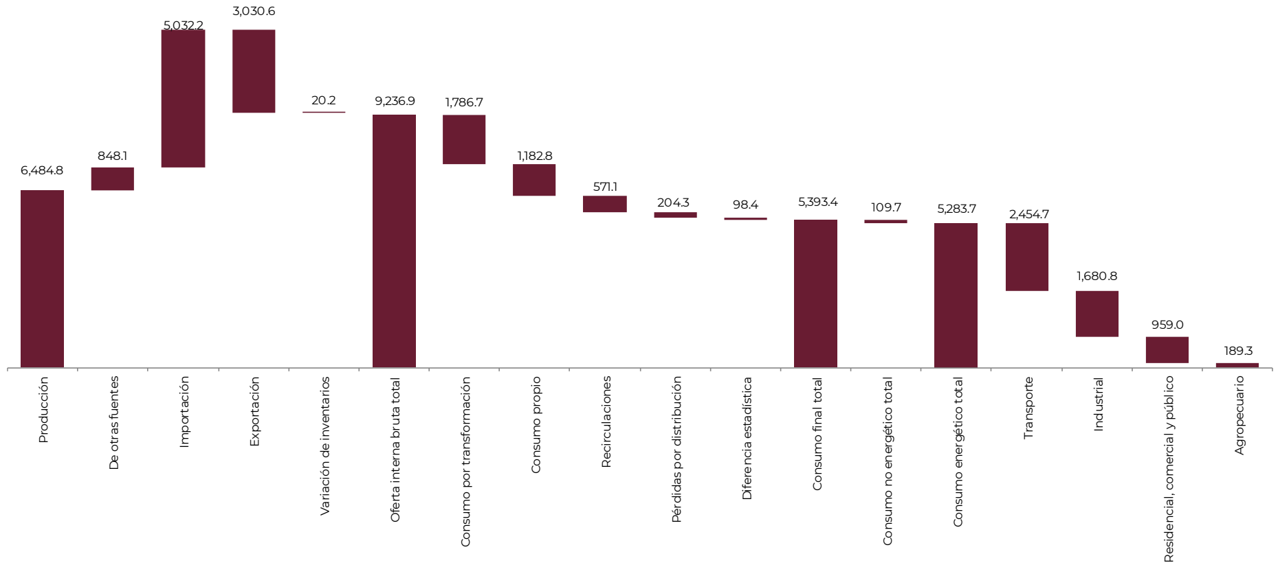
Figura 25. Balance Nacional de Energía, 2018 (Petajoules)
