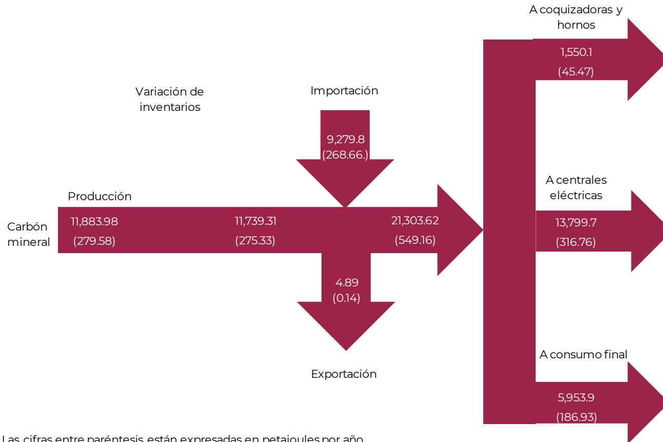
Diagrama 3. Balance de carbón 2018, miles de toneladas (Petajoules)
