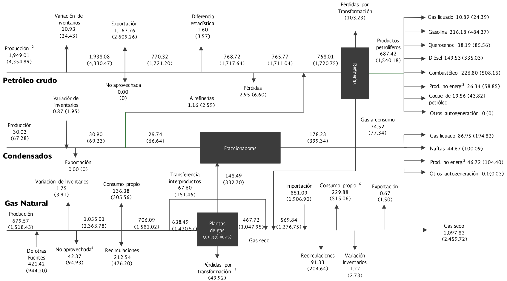
Diagrama 10. Balance de energía de hidrocarburos 2017, miles de barriles diarios (Petajoules)
