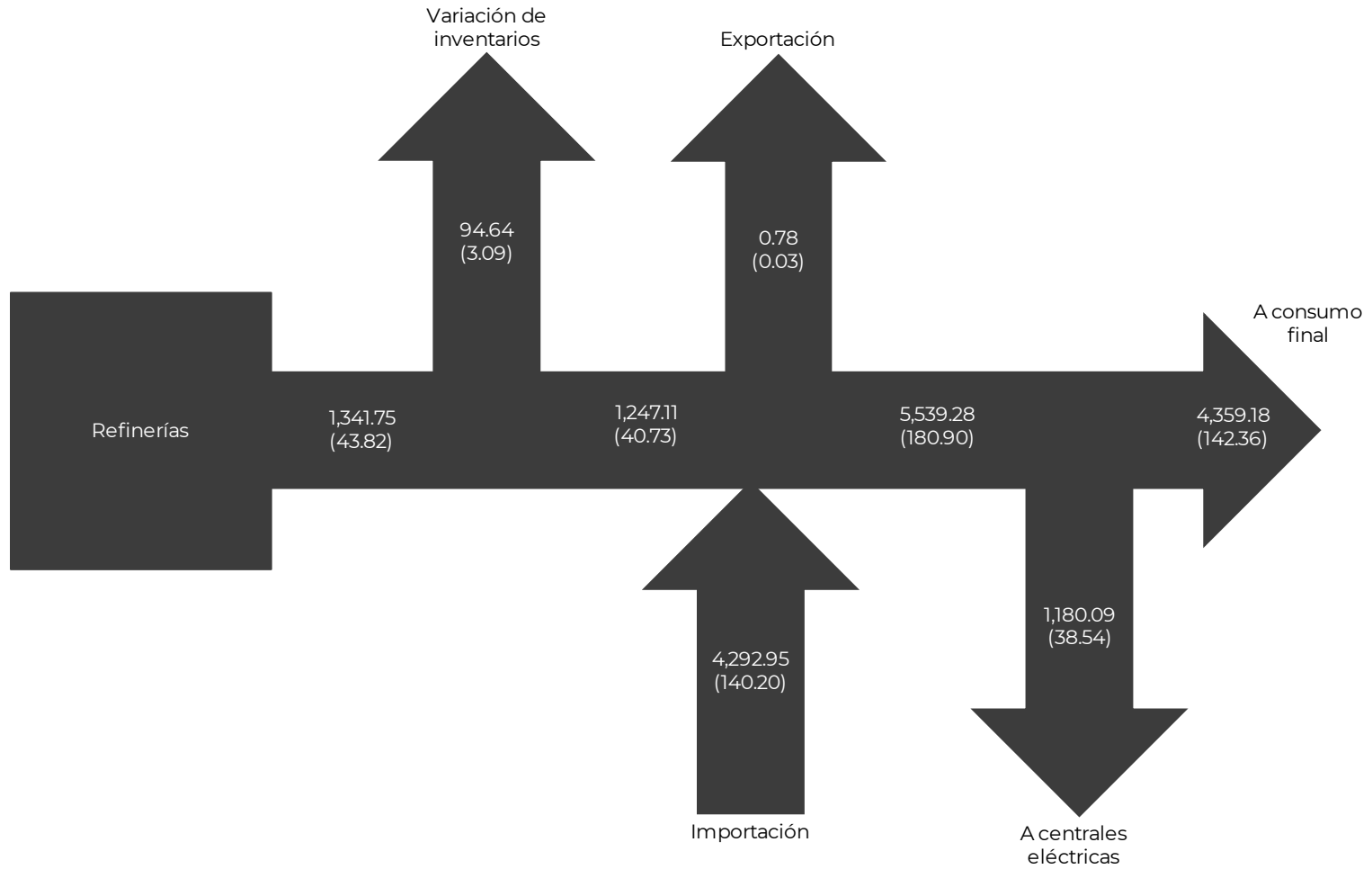
Diagrama 8. Balance de coque de petróleo 2017, miles de toneladas (Petajoules)
