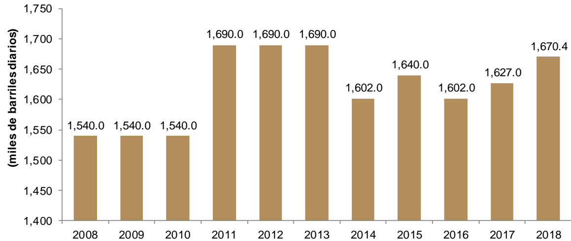
Evolución de la capacidad nominal de destilación atmosférica 2008-2018
