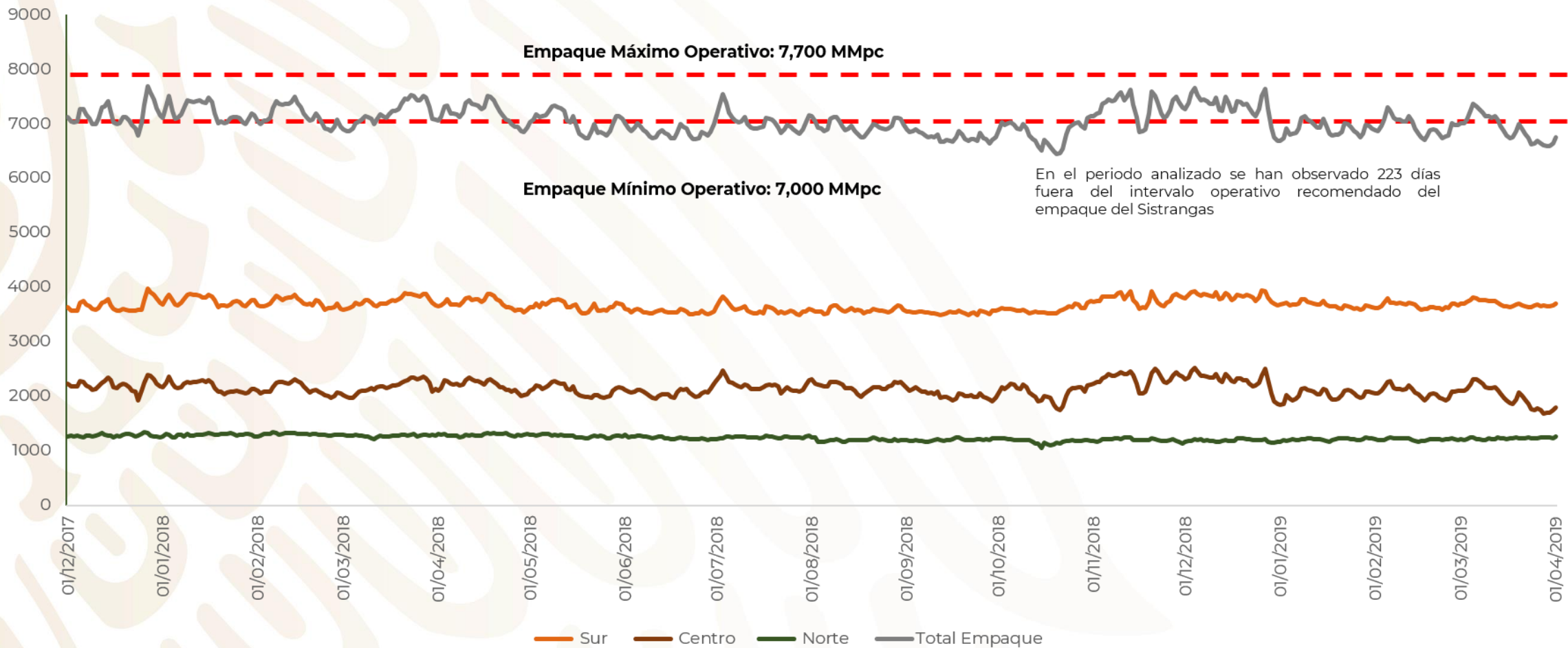
Nivel del empaque (MMpcd)
