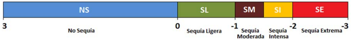
Escala del Índice de Sequía por Ecurrimiento
