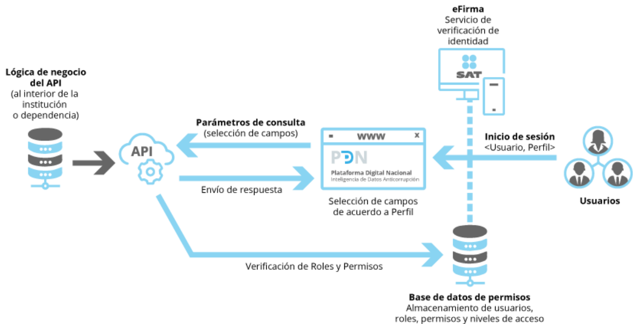
Figura 1. Esquema conceptual del flujo de comunicación entre Instituciones y la Plataforma Digital Nacional. De derecha a izquierda se observan usuarios con diferentes perfiles accediendo a la PDN y solicitando información de acuerdo a sus atribuciones.
