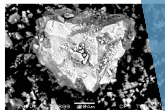
Micrografías del clinker del cemento Portland CPC 30R RS
