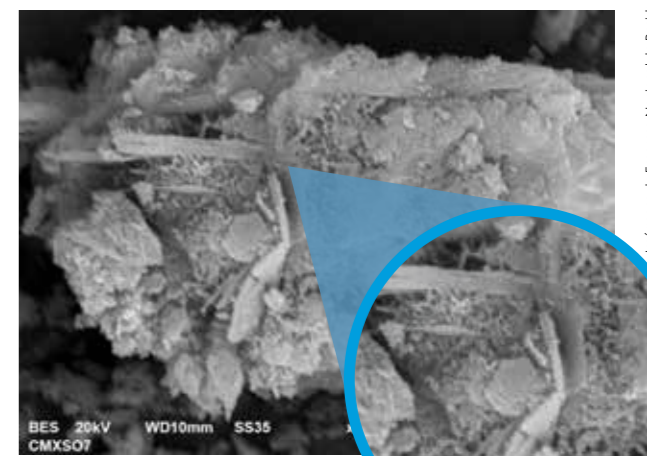
Micrografías de la pasta de cemento Portland hidratado
