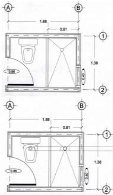
CROQUIS BAÑO
