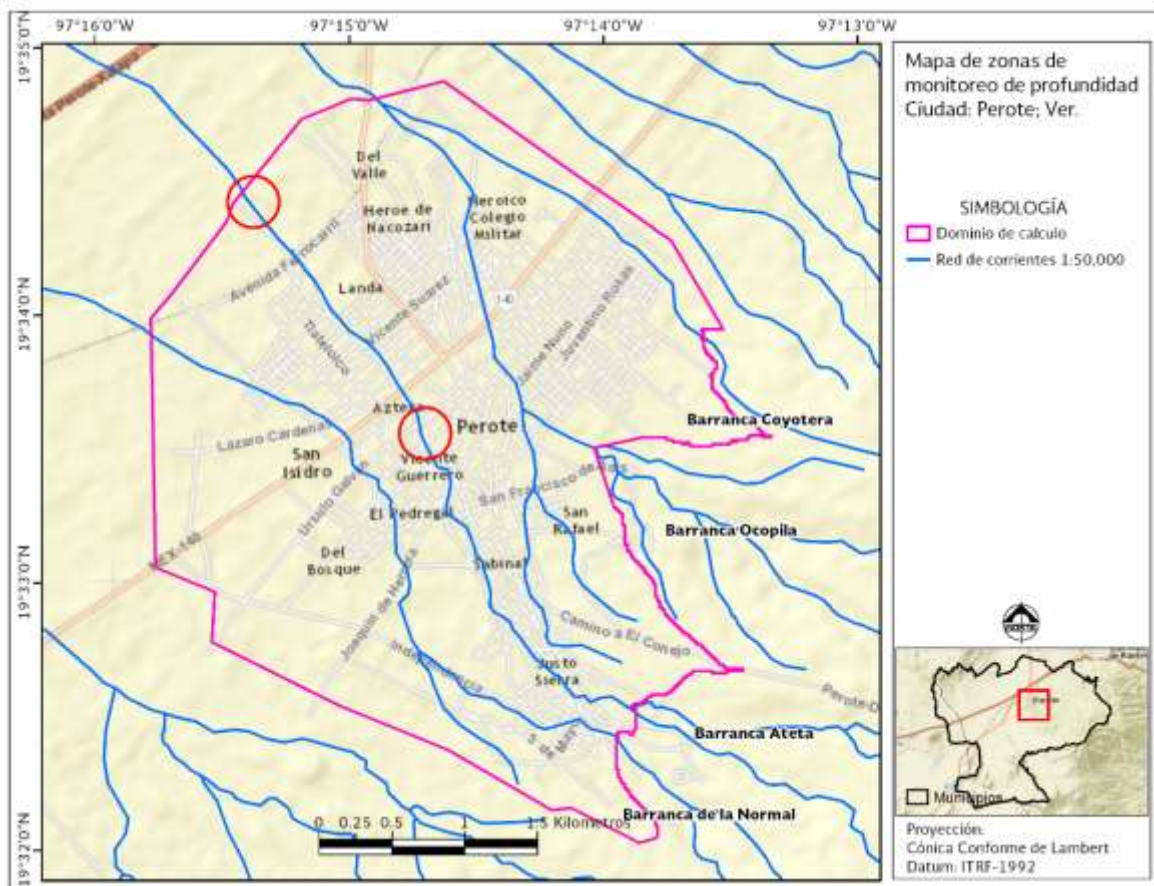
Figura 5.30 Zonas de tirantes máximos alcanzados (Tr= 100 años)
