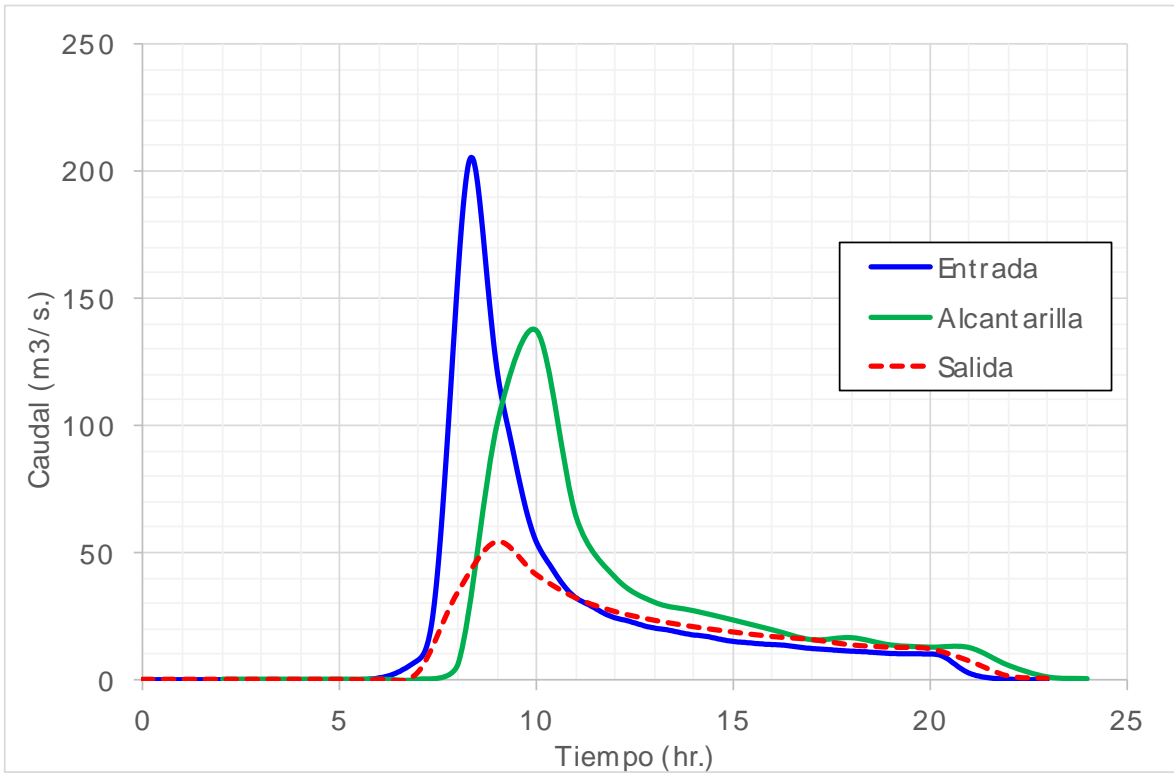
Figura 5.29 Hidrograma de entrada y salida de la subcuena 3 de Perote (Tr=100 años)
