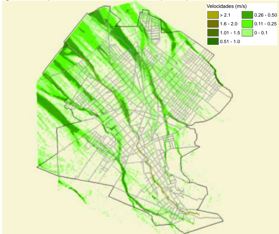
Figura 5.19 Mapa de velocidades máximas alcanzadas para un periodo de retorno de 10 años
