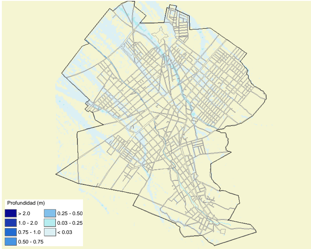
Figura 5.14 Mapa de tirantes máximos alcanzados para un periodo de retorno de 2 años
