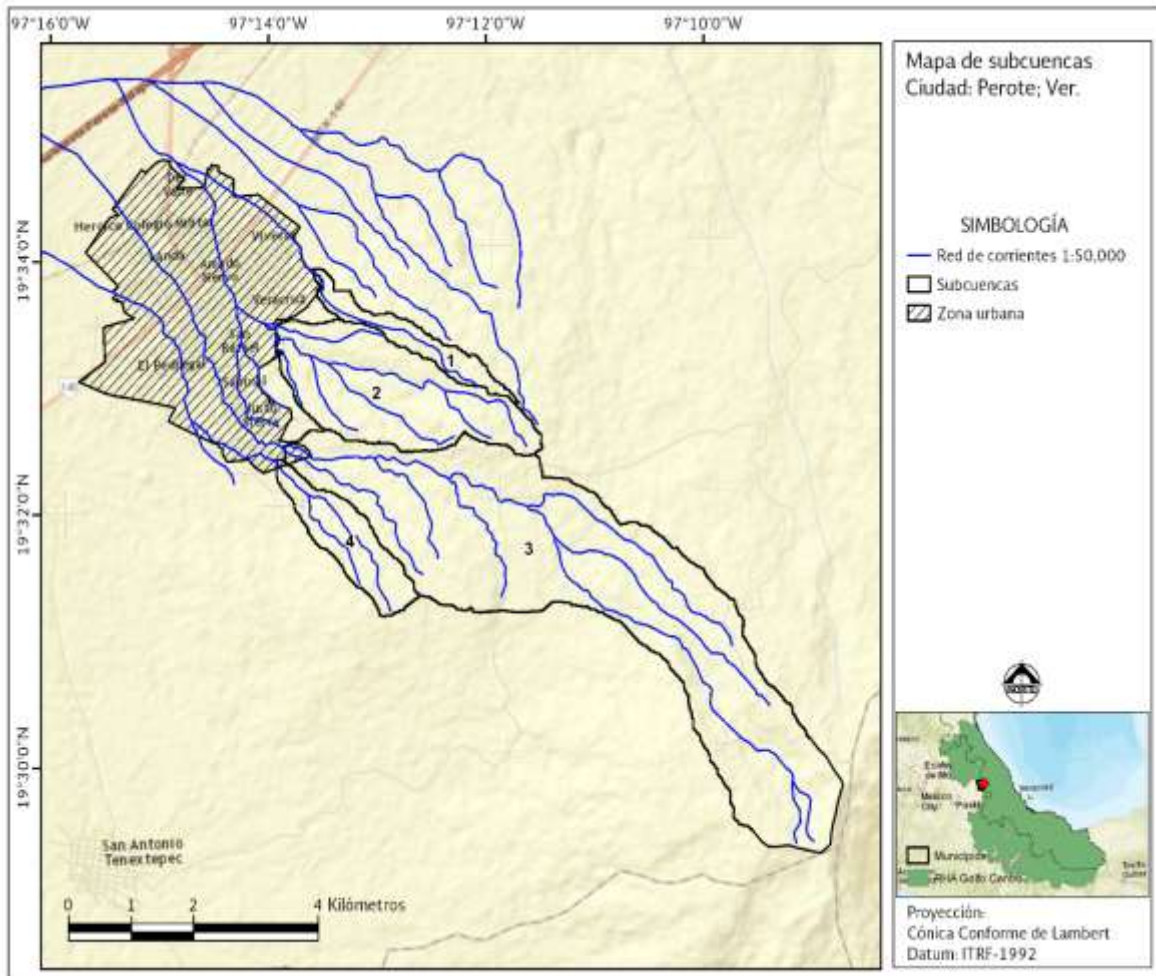
Figura 3.4 Subcuencas de aportación
