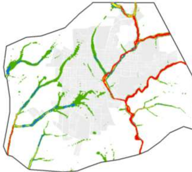
Figura 5.35 Mapa de severidad para un periodo de retorno de 100 años en Arandas, Jalisco
