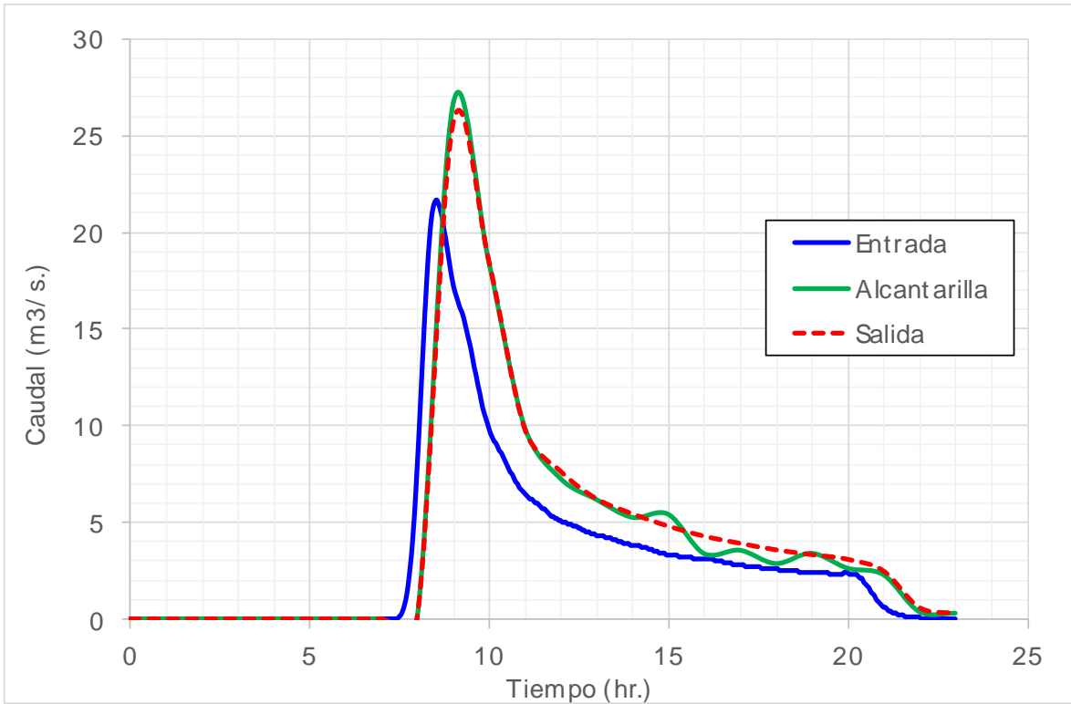
Figura 5.26 Hidrograma de entrada y salida de la subcuena 3 de Perote (Tr=5 años)
