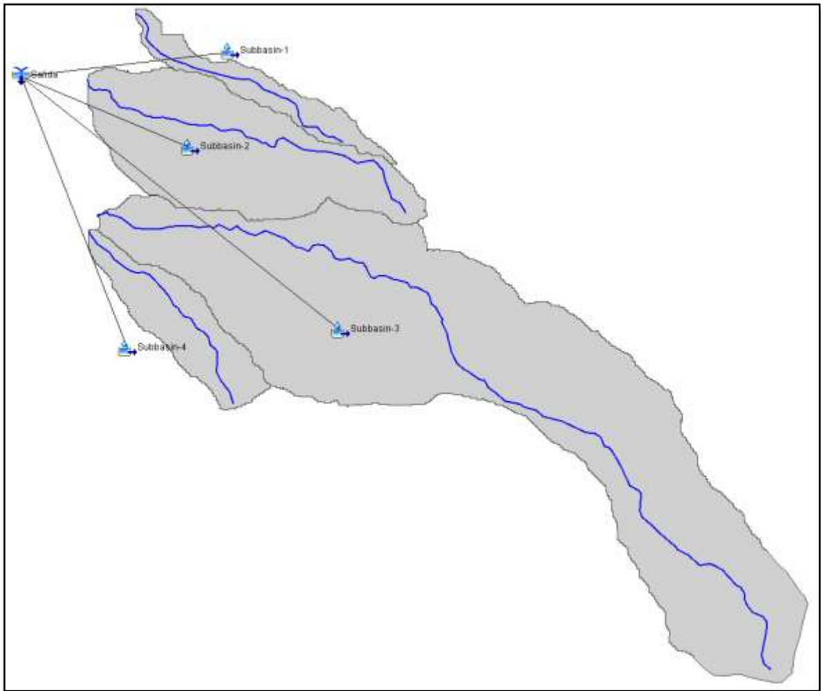
Figura 5.3 Esquema del modelo hidrológico
