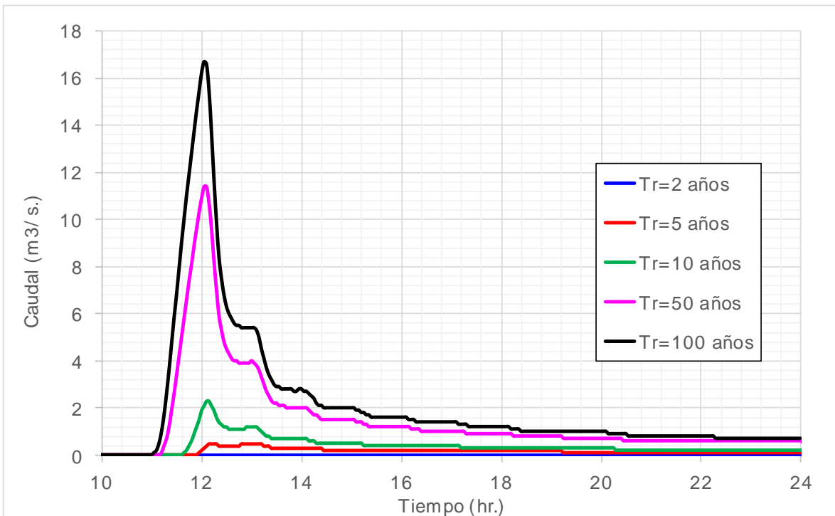
Figura 5.7 Hidrogramas a la salida de la subcuenca 4 (Barranca de la Normal)
