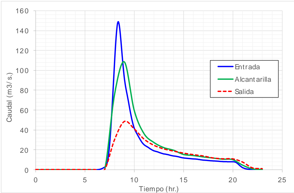
Figura 5.28 Hidrograma de entrada y salida de la subcuena 3 de Perote (Tr=50 años)
