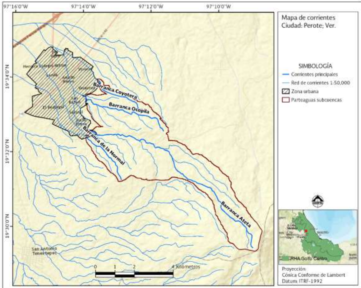
Figura 3.10 Principales ríos y corrientes
