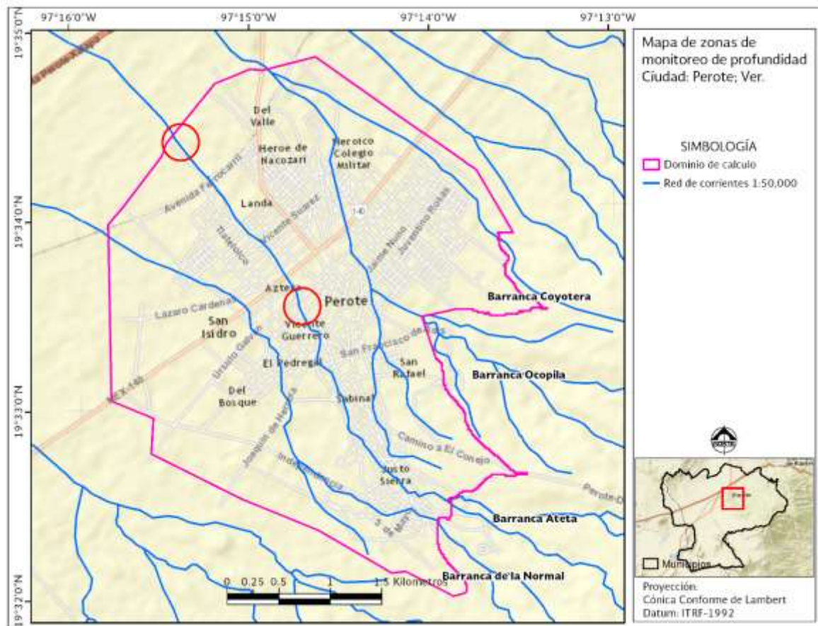
Figura 5.24 Sitios de monitoreo de la evolución de los escurrimientos
