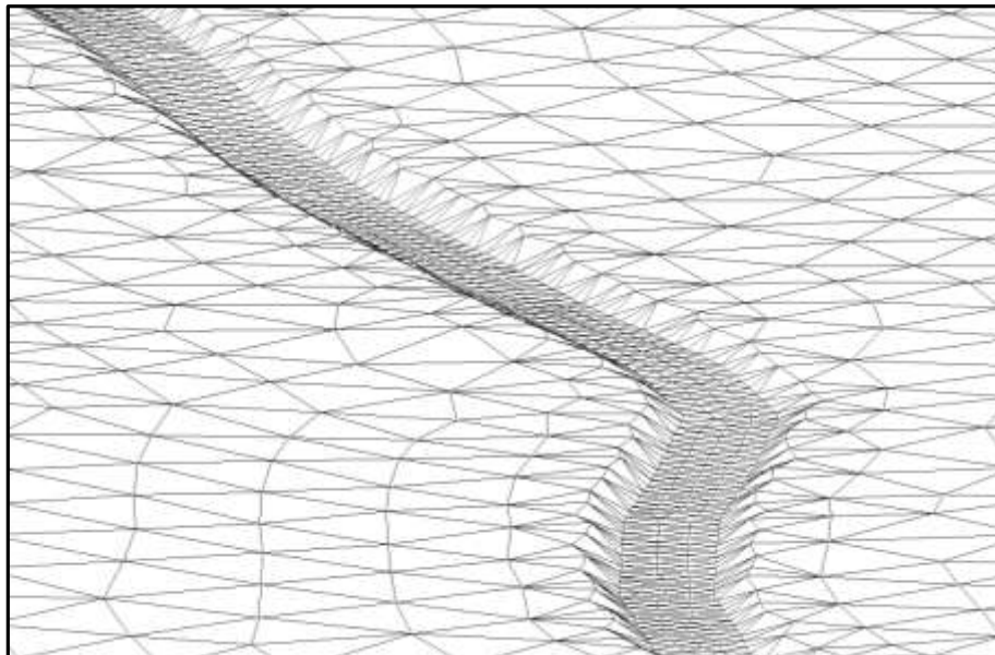
Figura 5.9 Mallado obtenido con el modelo IBER, en la zona de un arroyo de Perote
