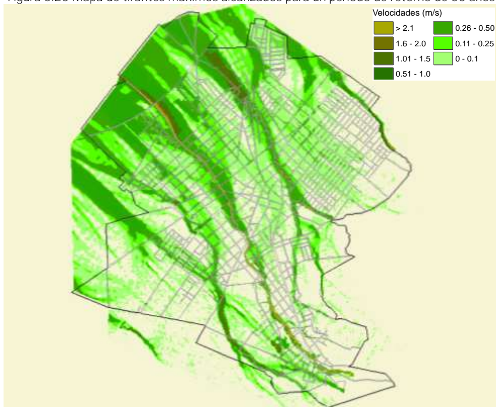
Figura 5.21 Mapa de velocidades máximas alcanzadas para un periodo de retorno de 50 años
