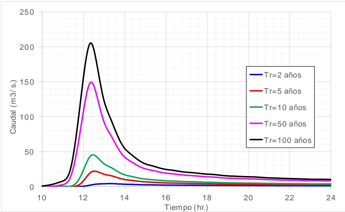
Figura 5.6 Hidrogramas a la salida de la subcuenca 3 (Barranca Ateta)
