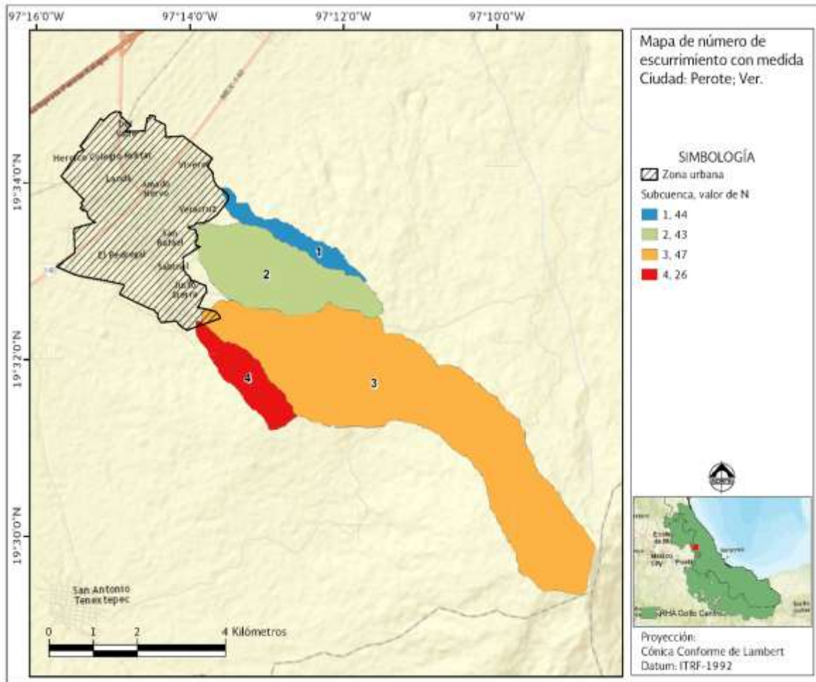
Figura 3.11 Variación del número de escurrimiento por subcuenca
