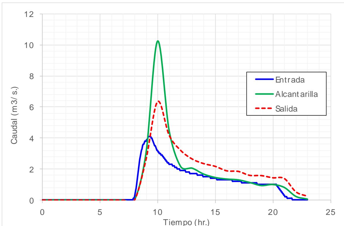
Figura 5.25 Hidrograma de entrada y salida de la subcuenca 3 de Perote ( Tr=2 años)
