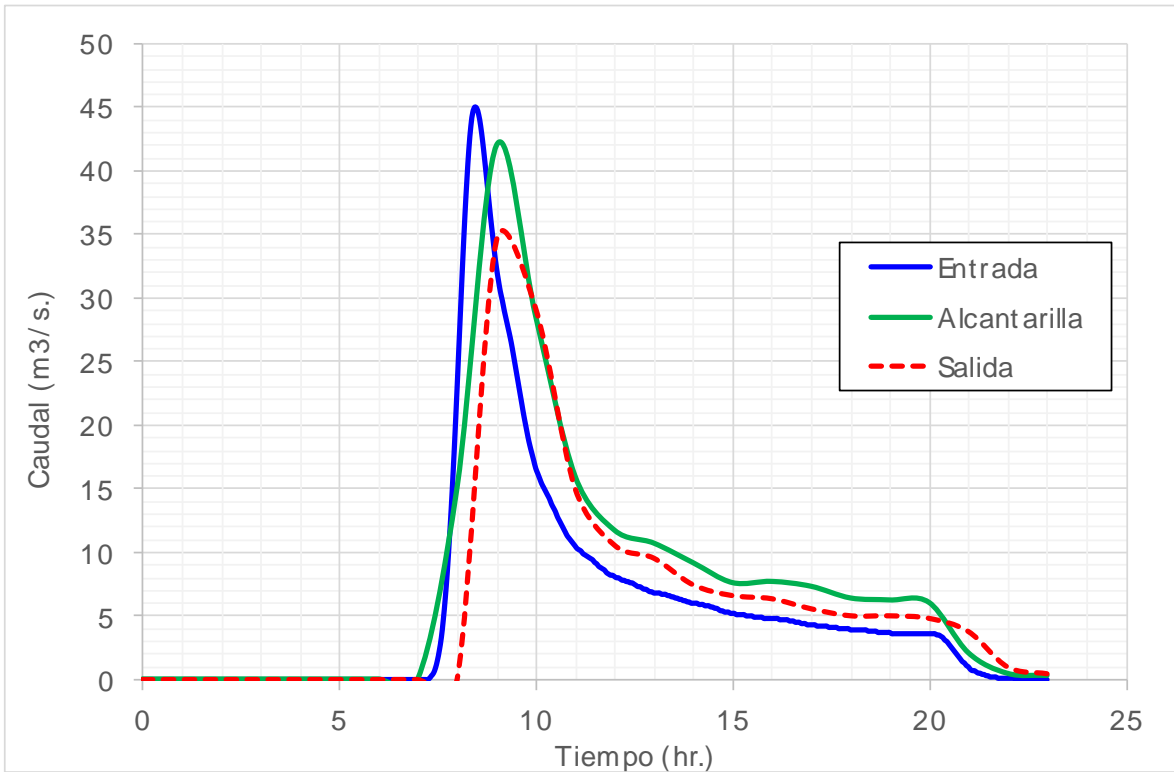
Figura 5.27 Hidrograma de entrada y salida de la subcuena 3 de Perote (Tr=10 años)
