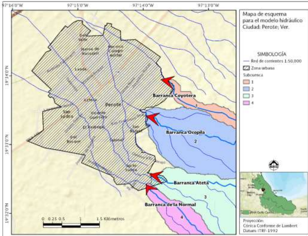
Figura 5.13 Esquema del modelo hidráulico para la ciudad de Perote; Ver
