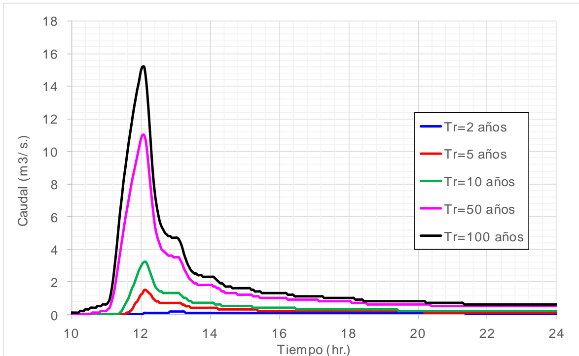
Figura 5.4 Hidrogramas a la salida de la subcuenca 1 (Barranca Coyotera)
