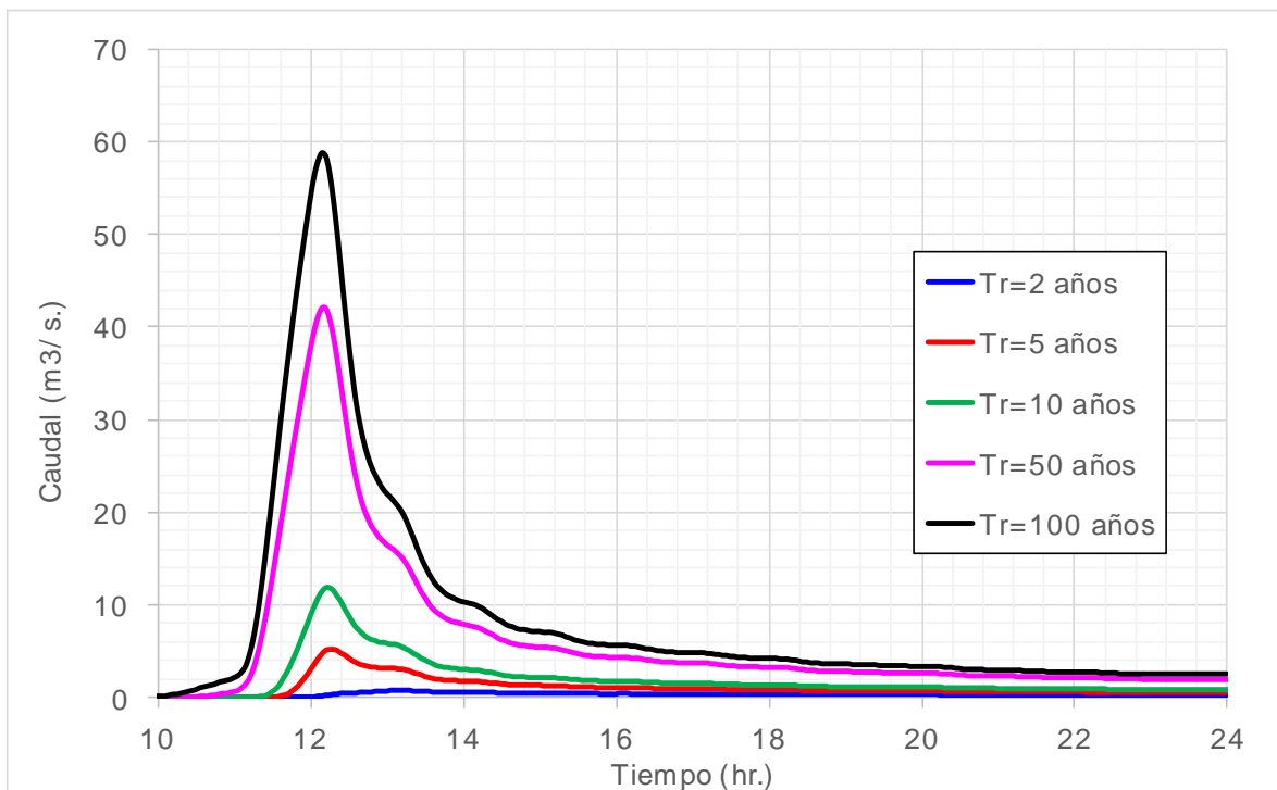
Figura 5.5 Hidrogramas a la salida de la subcuenca 2 (Barranca Ocopila)
