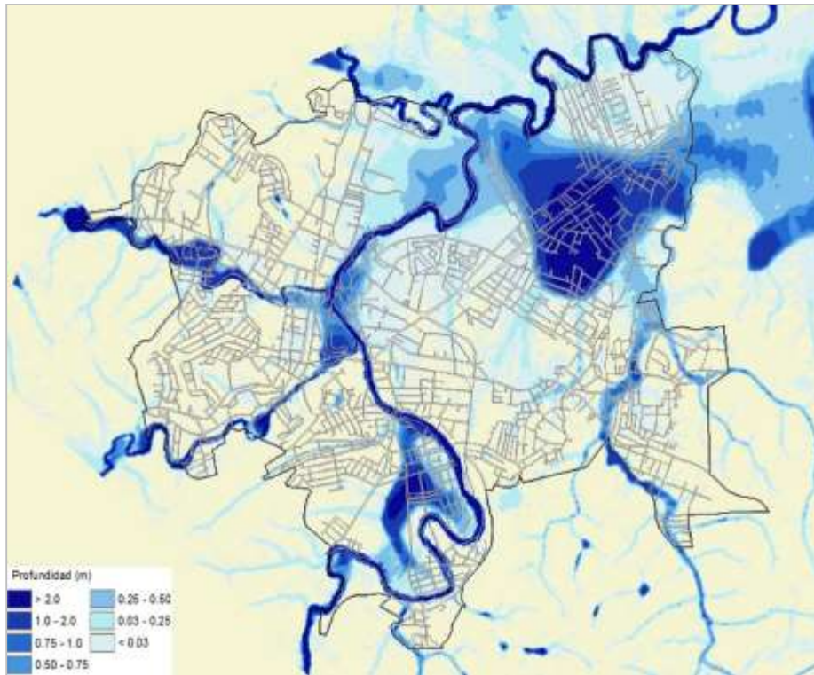
Figura 5.17. Mapa de tirantes máximos para un Tr de 10 años.
