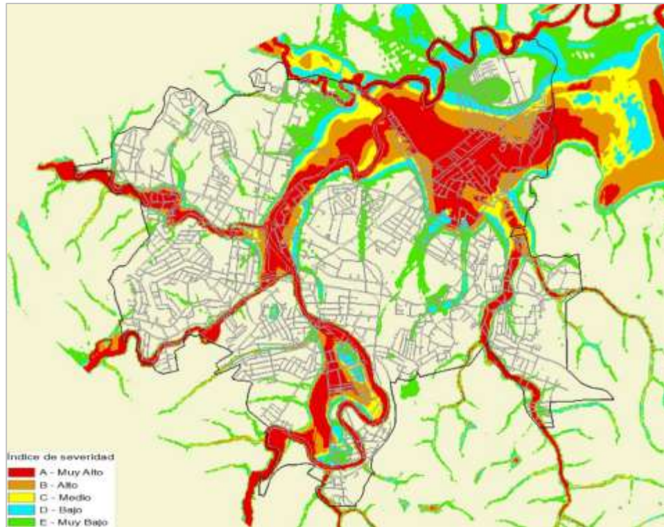
Figura 5.29. Mapa de severidad para un periodo de retorno de 100 años.
