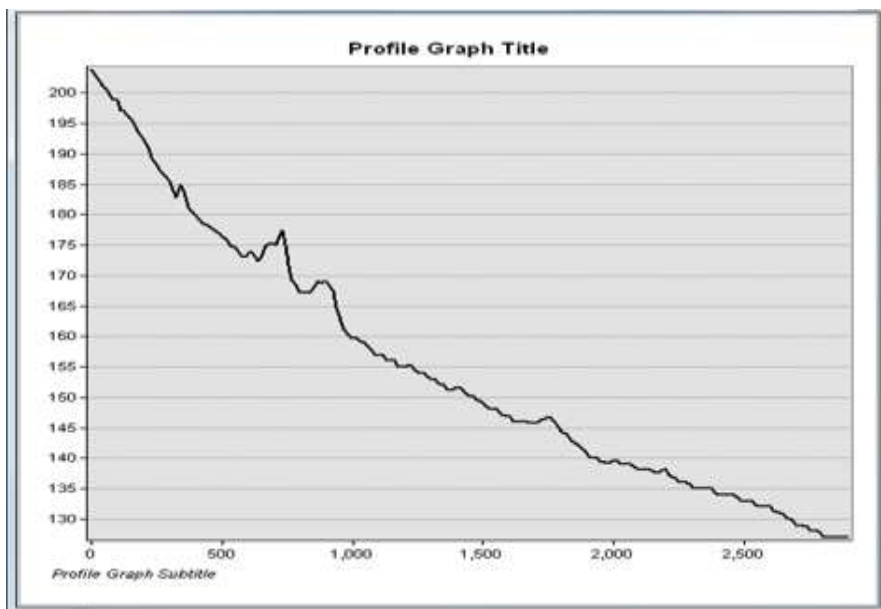
Figura 5.8. Perfil longitudinal con errores considerables
