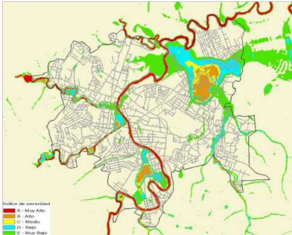
Figura 5.25. Mapa de severidad para un periodo de retorno de 2 años.
