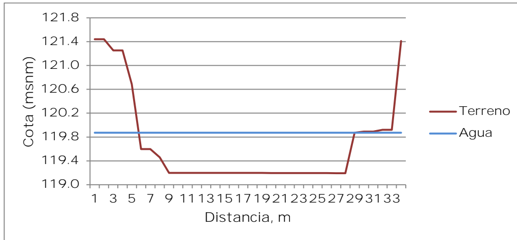
Figura 5.34 Cota de agua en la sección 2 para un periodo de retorno de 100 años
