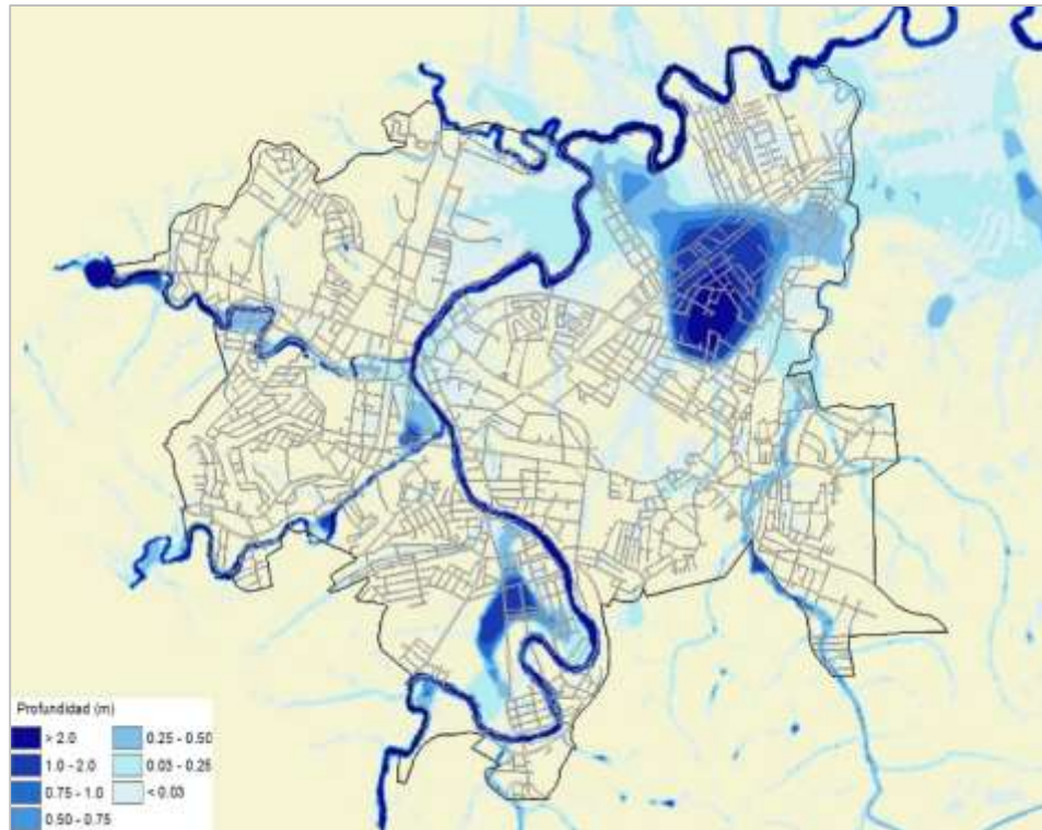
Figura 5.13. Mapa de tirantes máximos para un Tr de 2 años.
