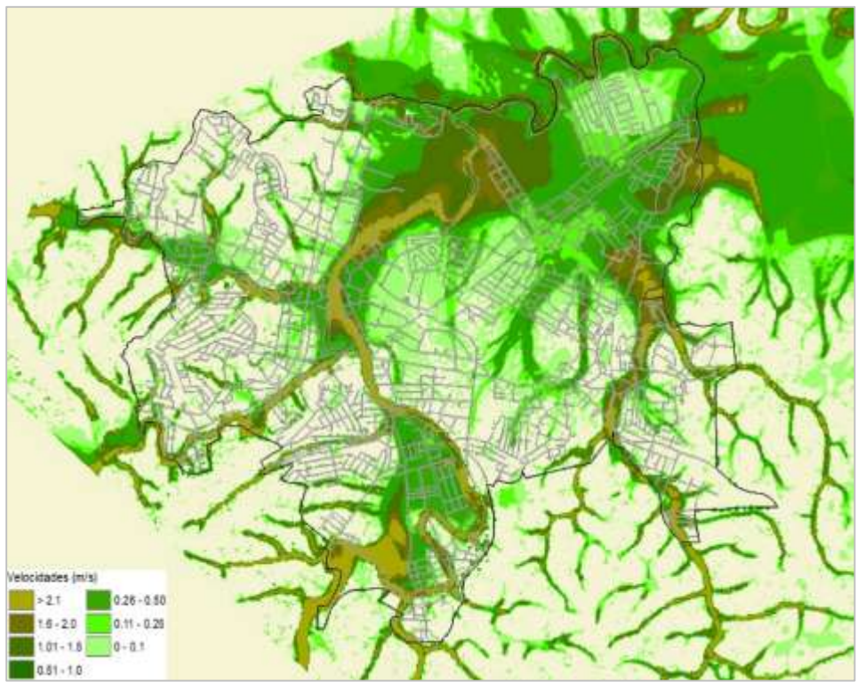
Figura 5.22. Mapa de velocidades máximas para un Tr de 100 años.
