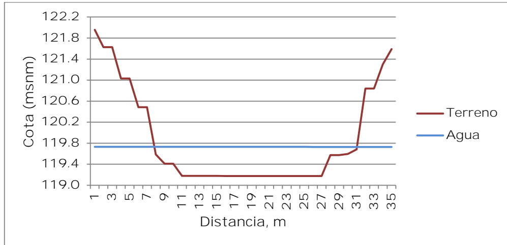
Figura 5.32 Cota de agua en la sección 2 para un periodo de retorno de 5 años.
