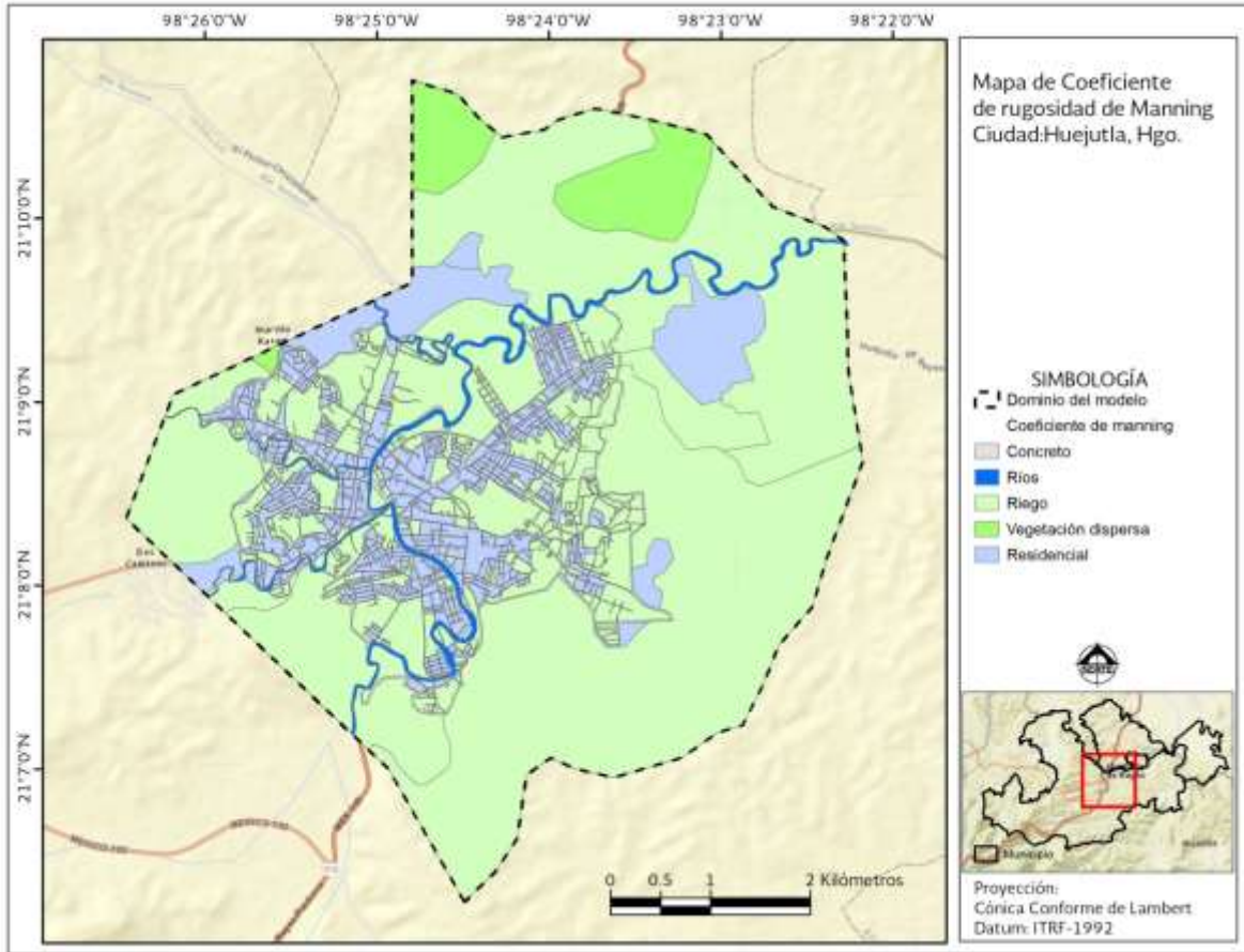
Figura 5.11 Variación del coeficiente de rugosidad en la zona de Huejutla, Hgo.
