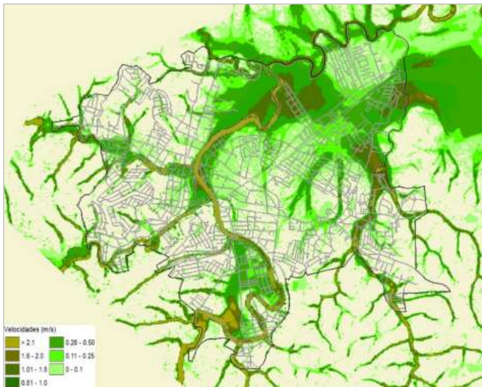
Figura 5.18. Mapa de velocidades máximas para un Tr de 10 años.
