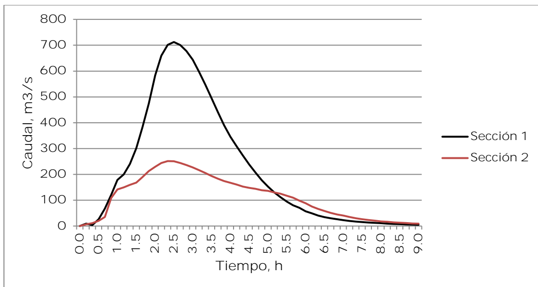
Figura 5.33. Hidrogramas en las secciones 1 y 2 para un periodo de retorno de 100 años.
