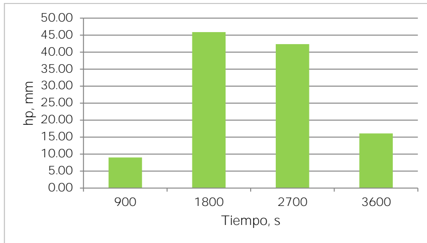
Figura 5.2 Distribución de la lluvia (100 años) a partir de una tormenta histórica en la Zona Urbana.
