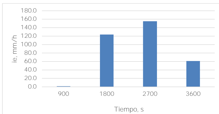
Figura 5.3. Hietograma de lluvia efectiva de 100 años para el área de modelación incluida la Zona Urbana.
