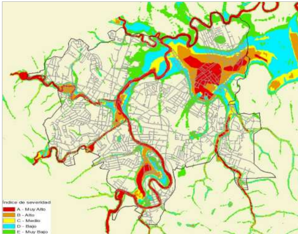
Figura 5.27. Mapa de severidad para un periodo de retorno de 10 años.
