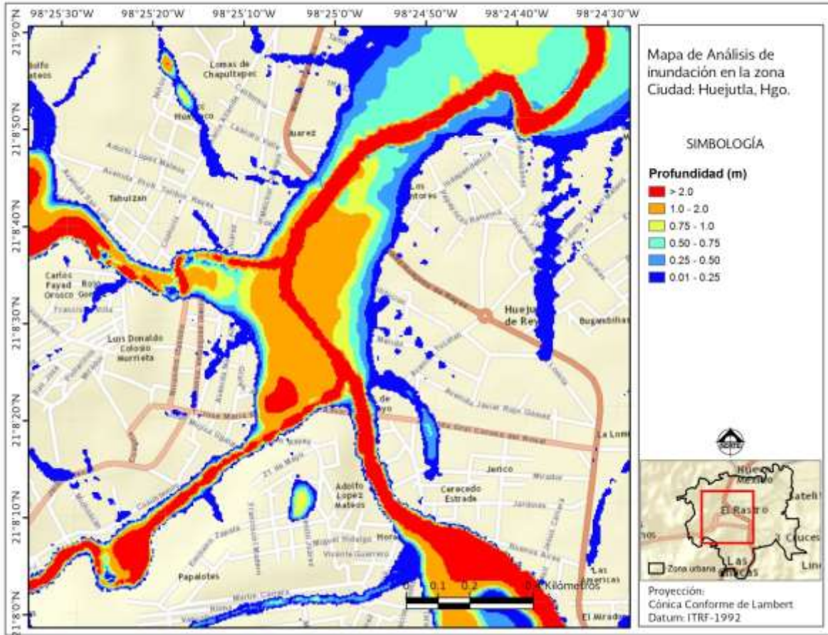
Figura 5.35 Mapa de tirantes máximos para un período de retorno de 100 años.
