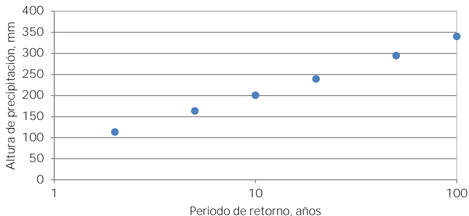
Figura 5.1. Lluvias de diseño (24 horas) en la cuenca de la zona urbana Huejutla, Hidalgo.
