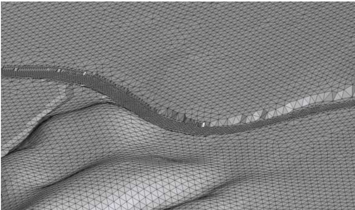
Figura 5.10. Incorporación de la “batimetría” del cauce en la malla del IBER.
