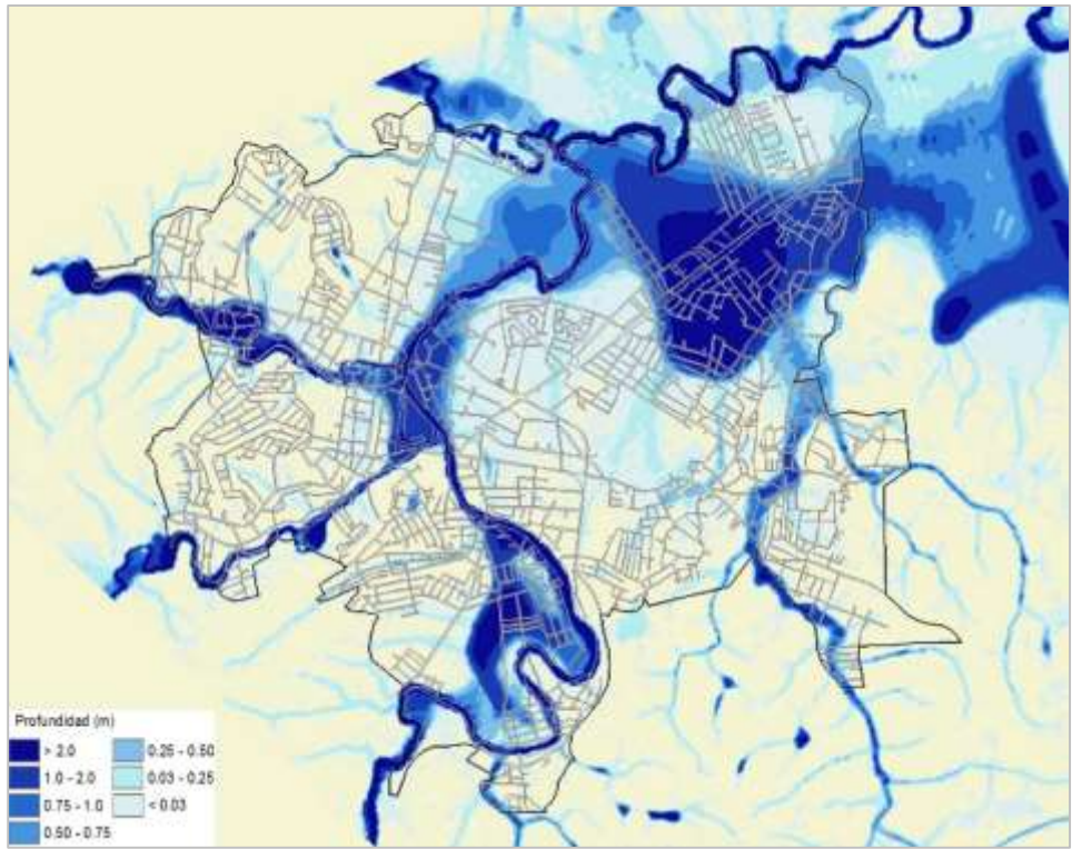
Figura 5.21. Mapa de tirantes máximos para un Tr de 100 años.
