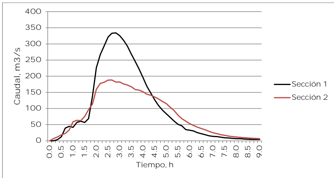
Figura 5.31 Hidrogramas en las secciones 1 y 2 para un periodo de retorno de 5 años.
