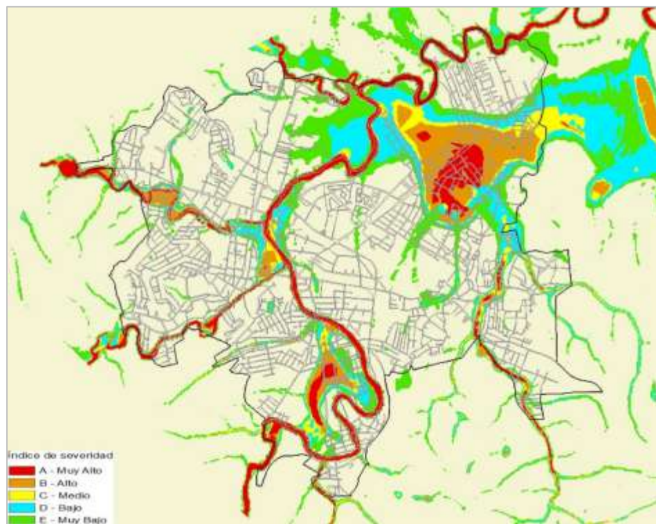
Figura 5.26. Mapa de severidad para un periodo de retorno de 5 años.
