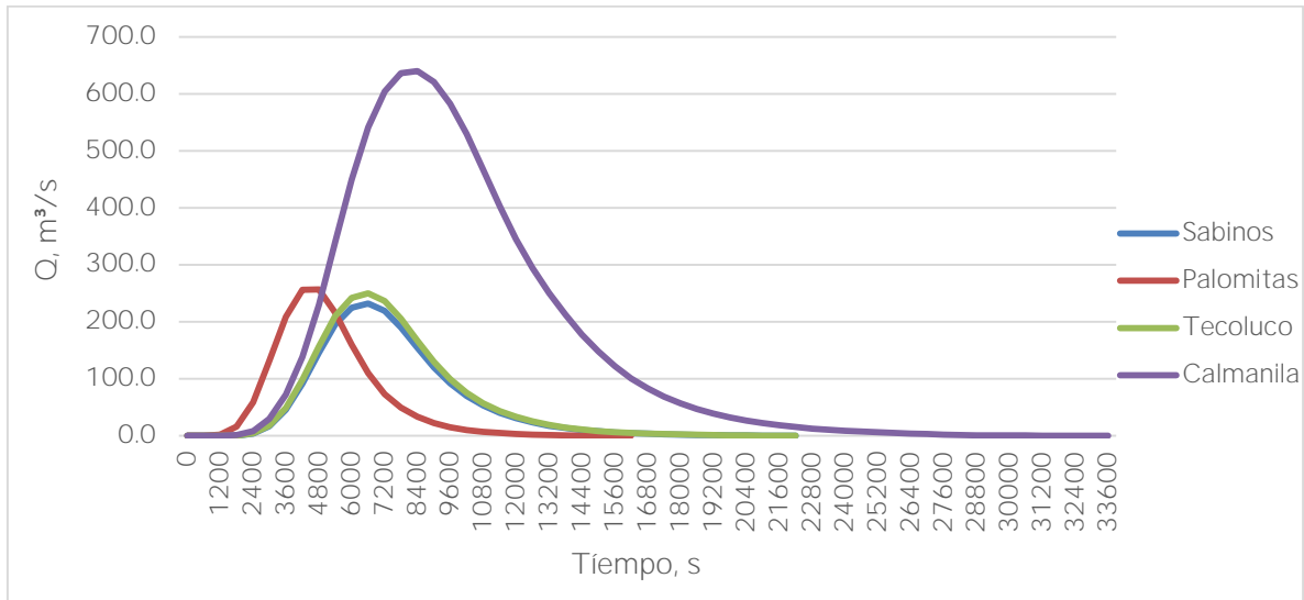
Figura 5.5. Hidrogramas para 100 años de periodo de retorno de cuatro subcuencas.
