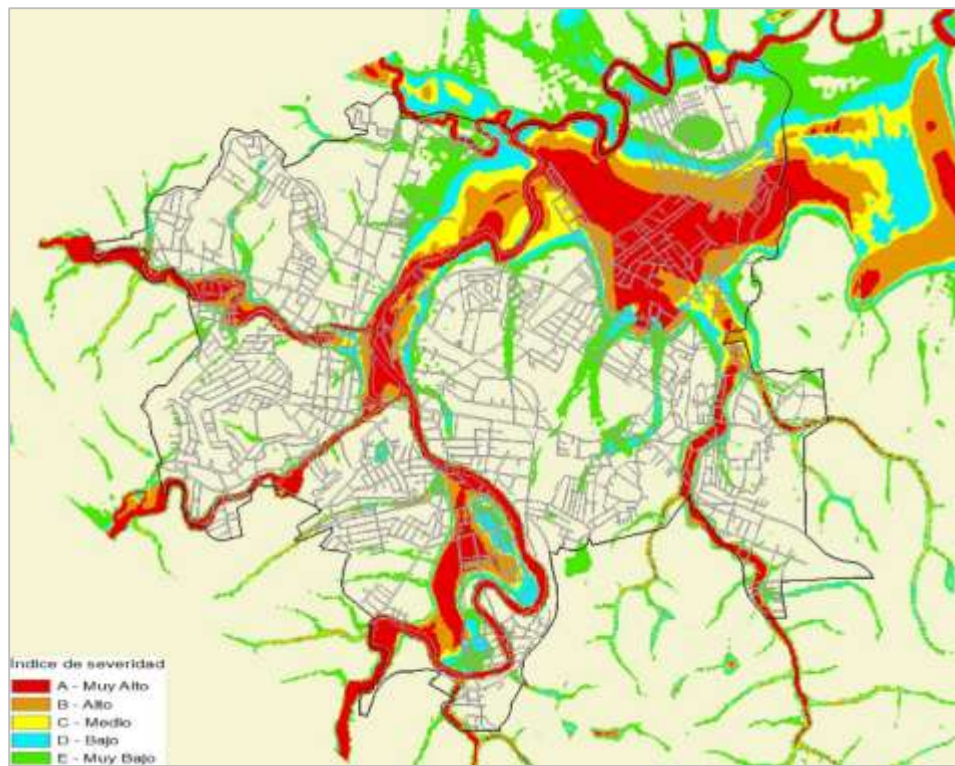
Figura 5.28. Mapa de severidad para un periodo de retorno de 50 años.
