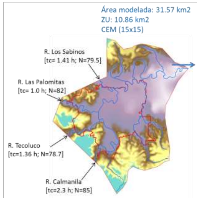
Figura 5.6. Entradas consideradas a la zona de modelación de la zona urbana de Huejutla, Hgo.
