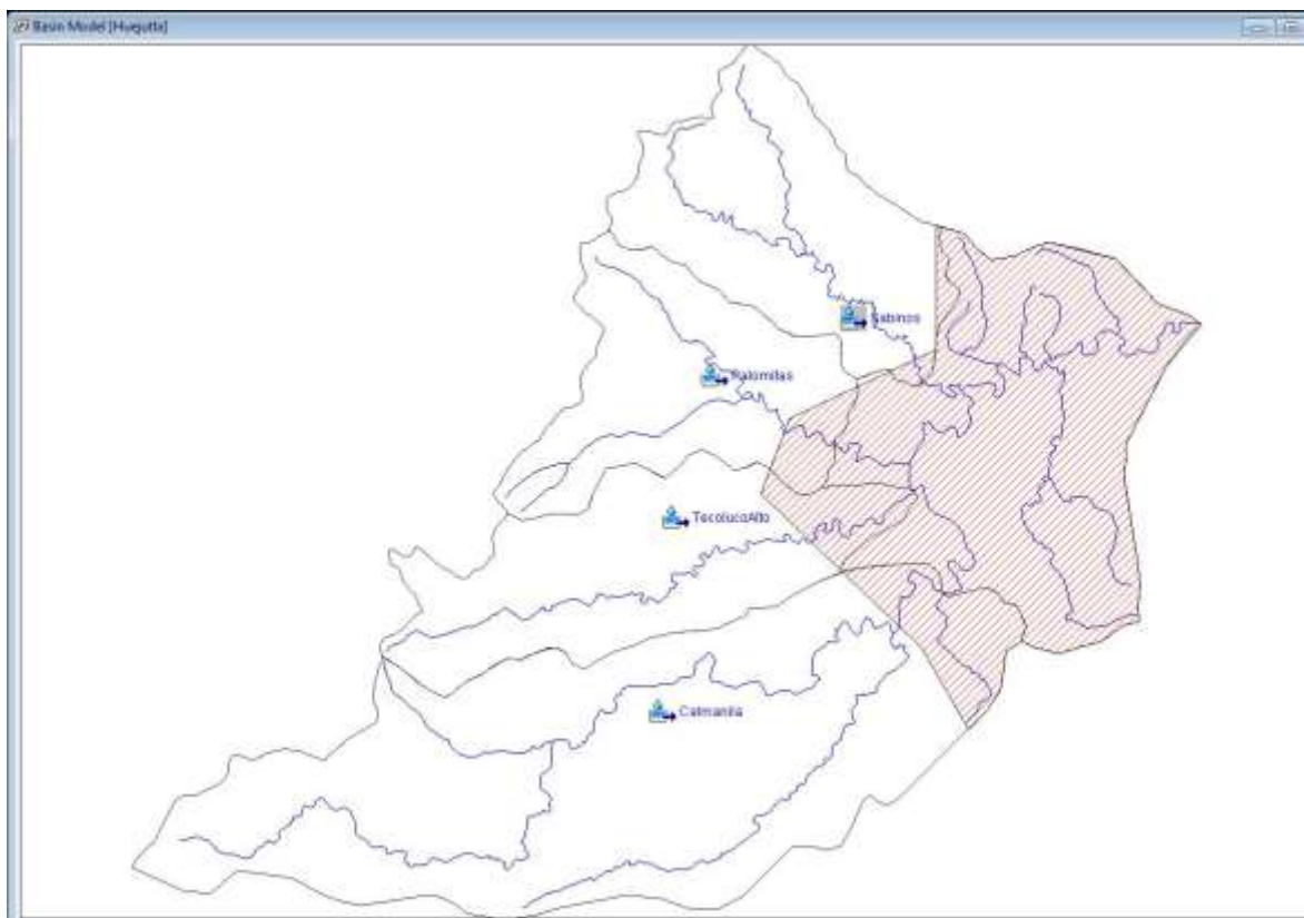
Figura 5.4. Esquema del modelo hidrológico en la plataforma HEC-HMS.
