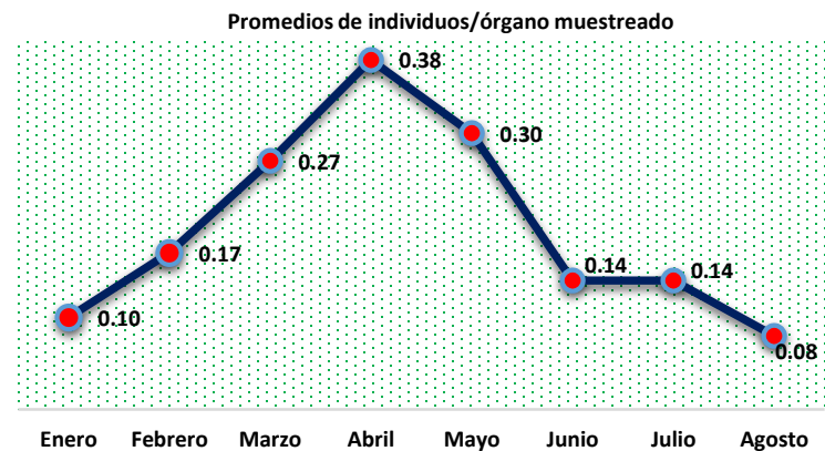
Gráfica 6. Densidades poblacionales nacionales al mes de agosto, 2017
