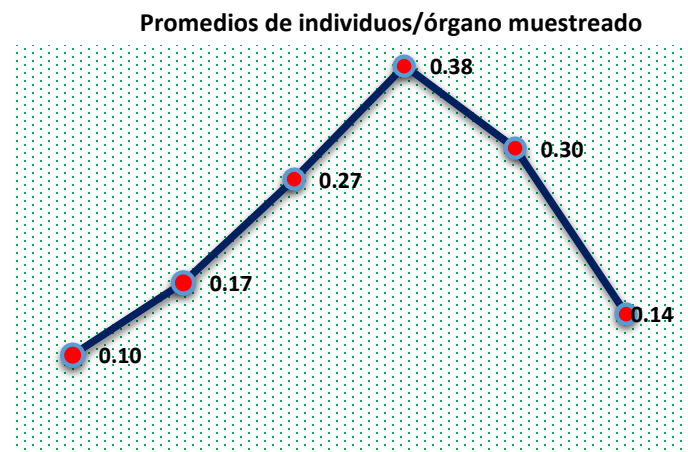
Gráfica 6. Densidades poblacionales nacionales al mes de junio, 2017
