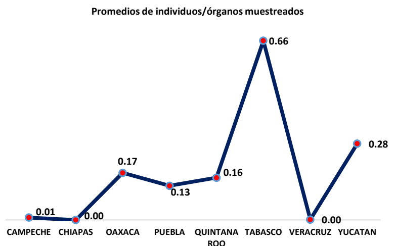
Gráfica 2. Densidades poblaciones al mes de junio
