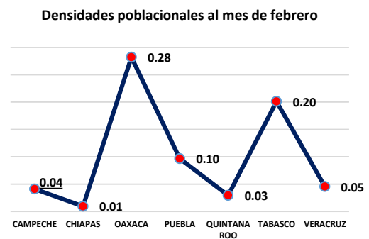
Gráfica 2.- Densidades poblacionales al mes de febrero, 2016.
