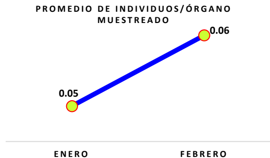
Grafica 3.- Promedios mensuales al mes de febrero, 2016.
