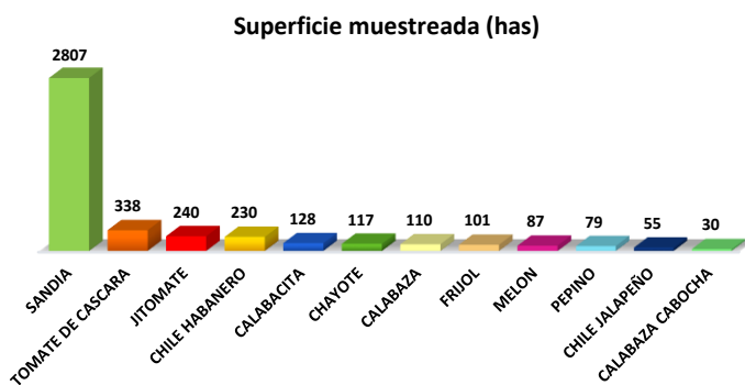
Gráfica 1.-Superficie muestreada por cultivo en el mes de febrero, 2016.
