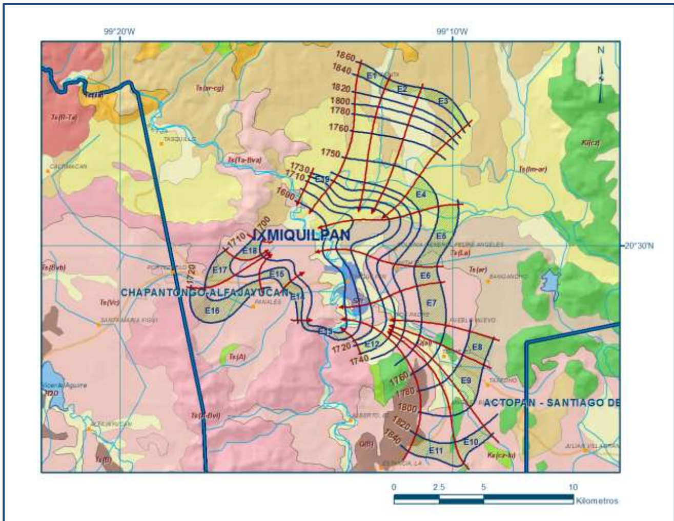
Figura 5. Elevación del nivel estático en msnm (2012)
