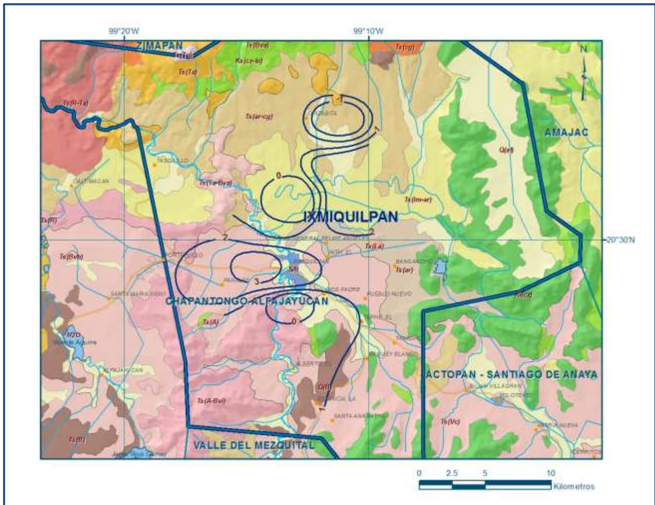
Figura 6. Evolución del nivel estático en m (2007-2012)
