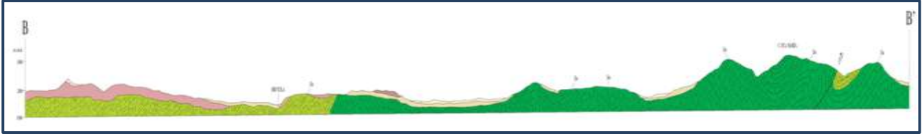
Figura 3. Sección geológica
