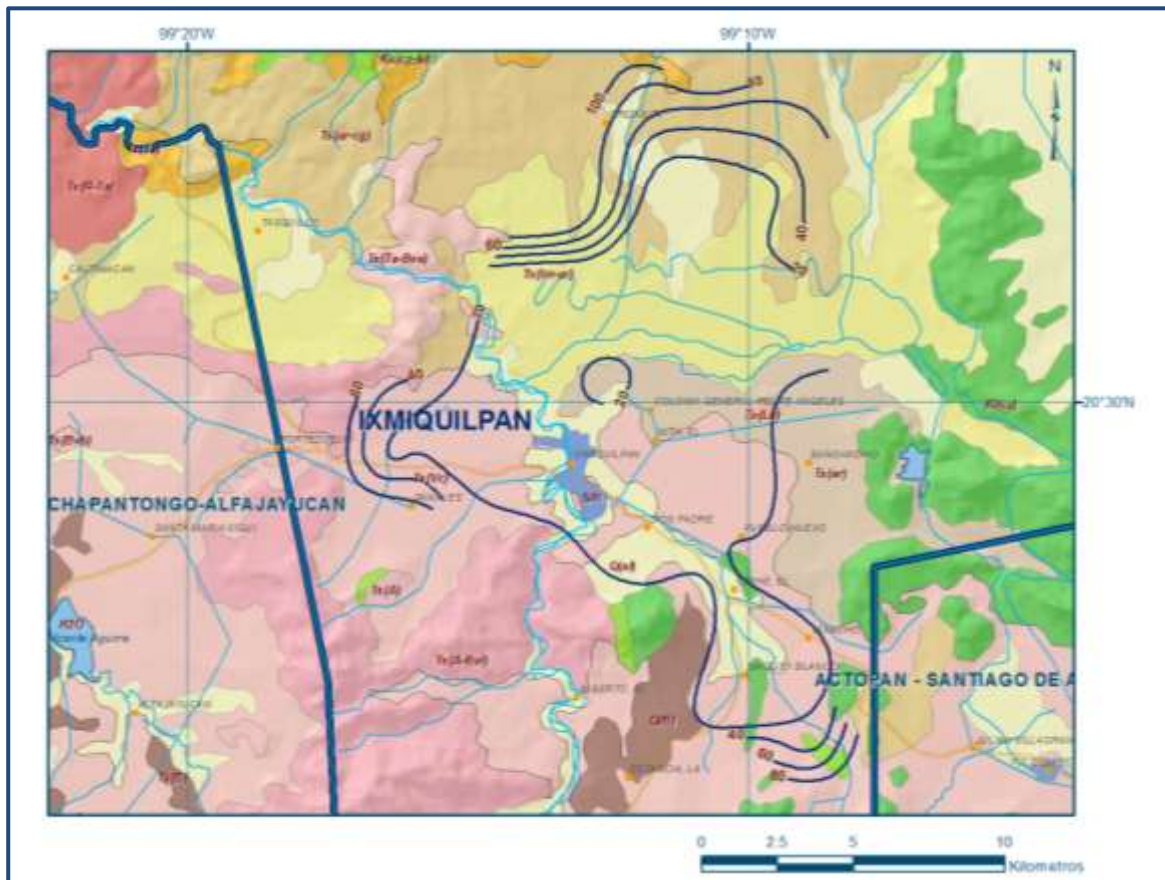
Figura 4. Profundidad al nivel estático en m (2012)
