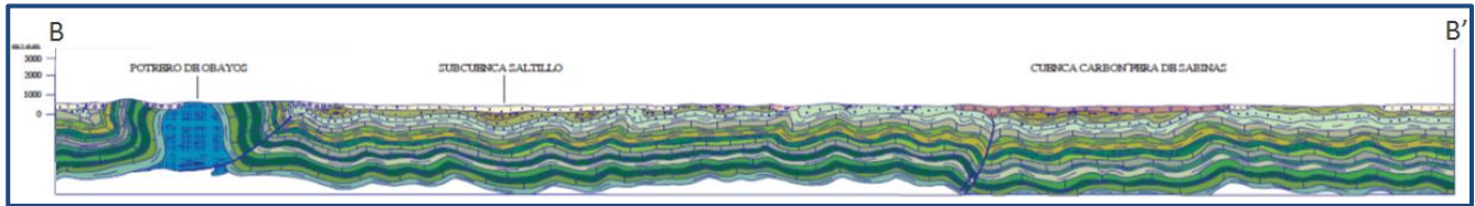
Fuente: Carta Geológica-Minera G14-1 "Nueva Rosita", Coahuila y Nuevo León. Esc. 1:250,000 (SGM, 2008) Figura 3. Sección geológica esquemática
