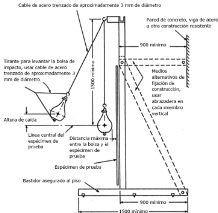
Figura 1.- Saco o pera para impacto no concentrado de alta y baja energía Acotaciones en mm
