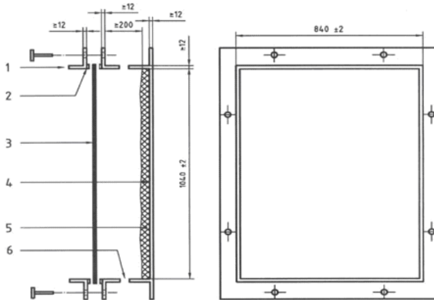
VISTA VERTICAL DEL BASTIDOR
