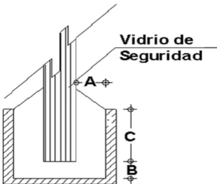
Figura 7.- Vidrio de Seguridad C.4A VIDRIO MONOLÍTICO
