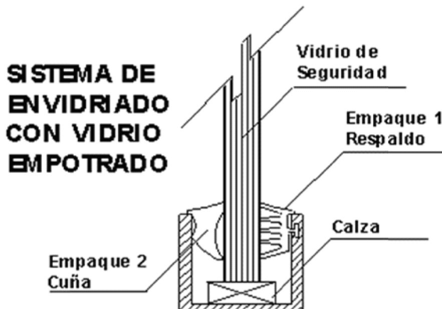
Figura 6.- Sistema de envidriado
