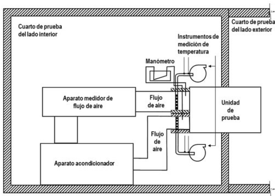
Figura A.2-Método de enlace de aire-entalpía
