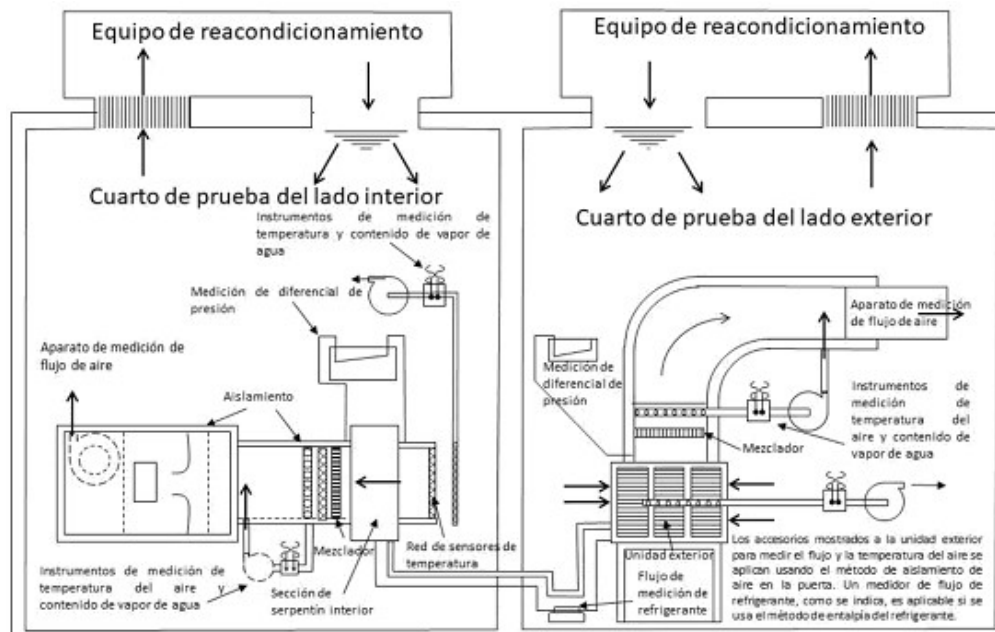
Figura A.1-Método de túnel aire-entalpía
