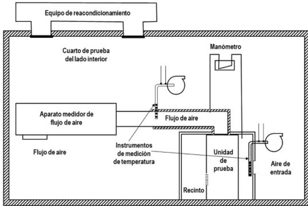
Figura A.3-Calorímetro aire-entalpía
