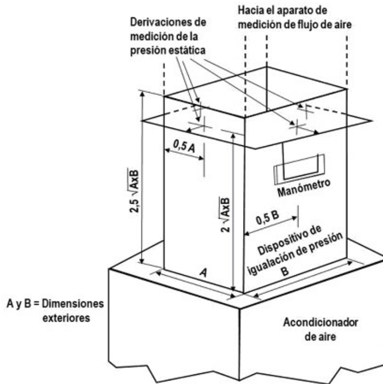
Figura A.7-Medición de la presión estática externa
