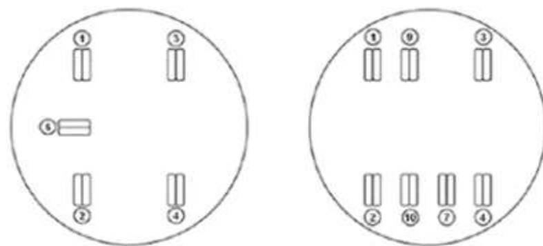
Figura 5- Identificación de la posición de las mordazas de sujeción del waththorímetro una base enchufe
