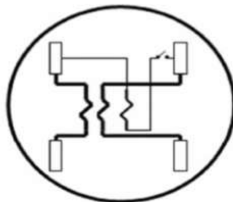
3 Hilos Auto contenido Forma 2S
