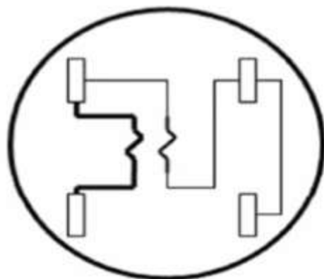
2 Hilos Auto contenido Forma 1S
