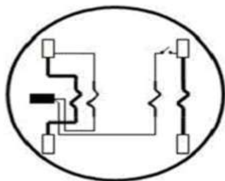
2 Estatores 3 Hilos Forma 12 S
