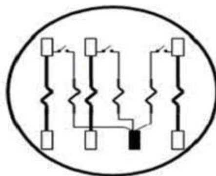
3 Estatores 4 Hilos y Estrella Forma 16 S
