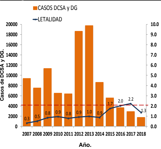
Gráfica 1. Casos de Dengue con Signos de Alarma y Dengue Grave, letalidad anual. México, 2007 – 2018.
