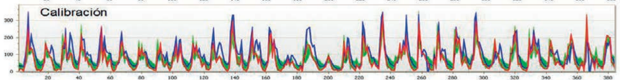
Figura 2.9. Período de calibración de caudales observados y medidos.
