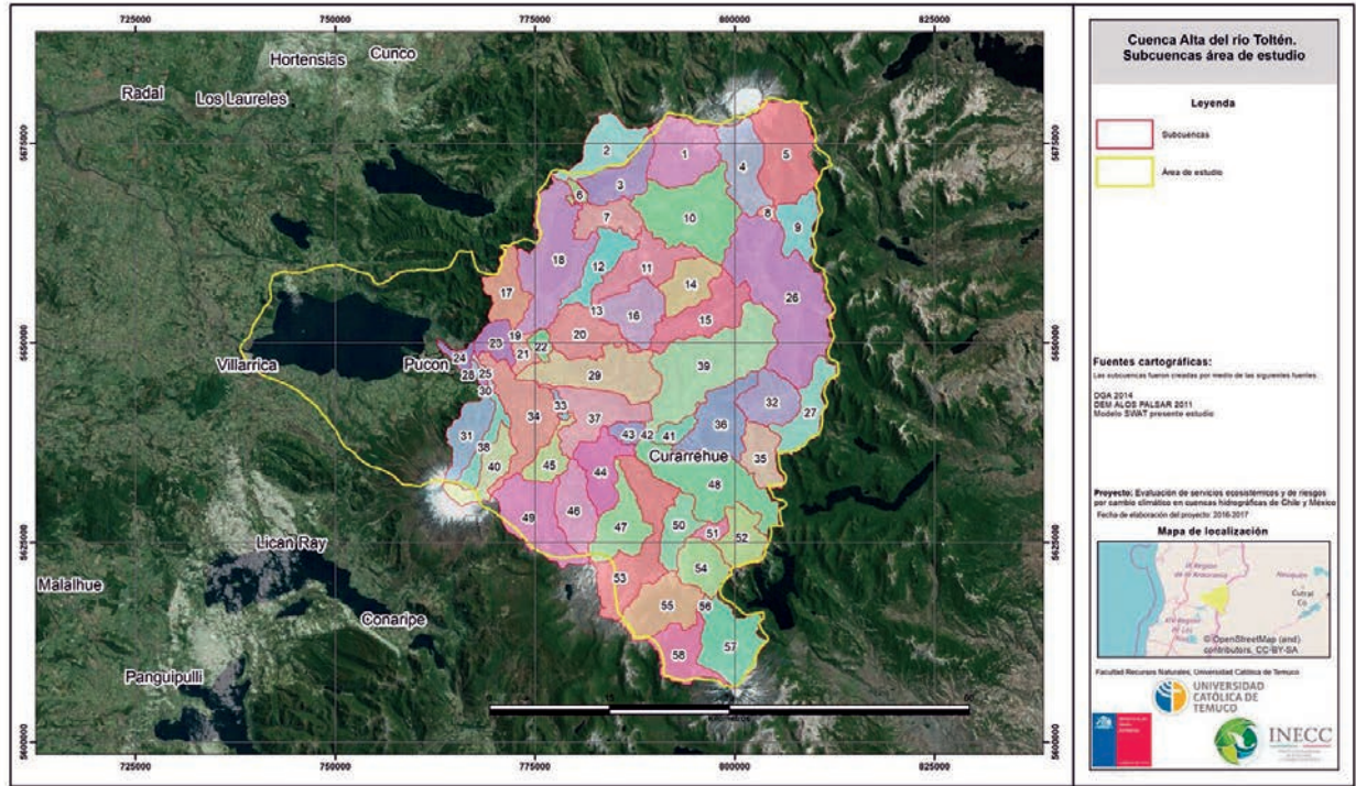
Figura 2.8. Identificación de unidades de respuesta hidrológica (HRU) y subcuencas.
