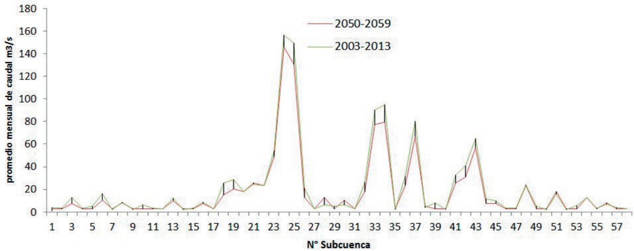
Figura 2.10. Comparación promedios mensuales períodos: 2003-2059 versus 2050-2059.
