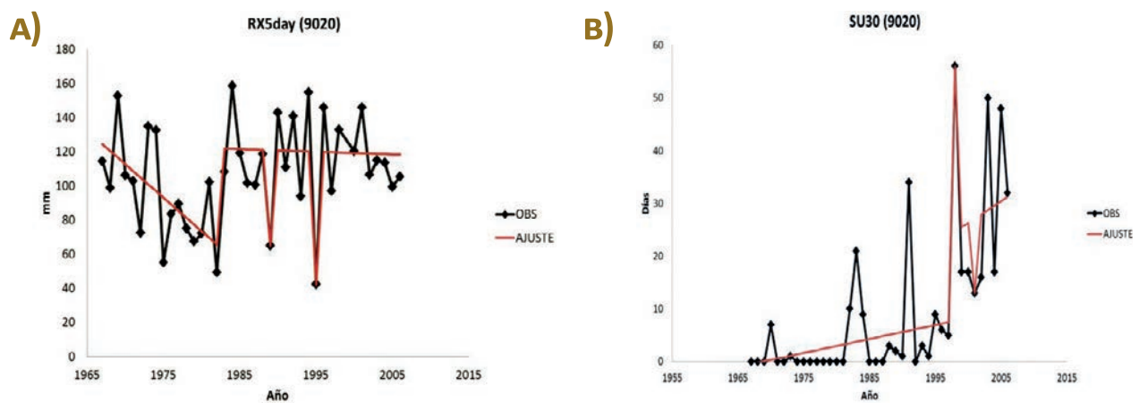
Figura 3.8. Gráficas de ajuste de tendencia en la estación 9020 (CDMX) para los índices de a) cantidad máxima de precipitación en 5 días consecutivos (RX5day), b) Días de verano – T_{max} > 30^{\circ}\text{C} (SU30). La línea roja representa el ajuste con el modelo de regresión lineal, en ambos casos se detectaron cambios de decremento e incremento, respectivamente.
