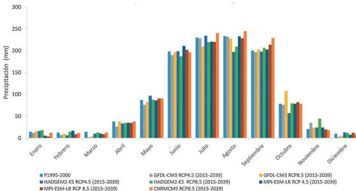
Figura 3.5. Precipitación en la Cuenca del Río Magdalena, histórica y proyectada.
