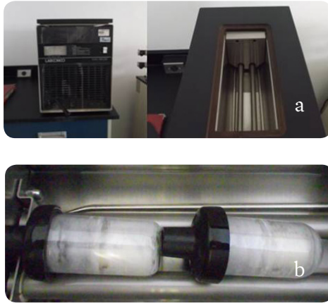
Figura 5.2 Ultracongelador de rodillos vista frontal y superior (a), Las botellas serológicas conteniendo el material biológico son colocadas en la cámara del ultracongelador, que contiene etanol y alcanza una temperatura de -50^{\circ}\text{C} (b).
