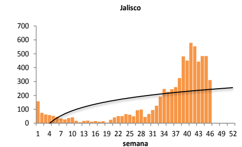
Gráfica 5. Curva epidémica en entidades con tendencia ascendente de casos estimados. México, 2016.
