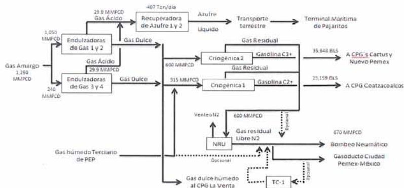
Diagrama General de Flujo de Procesos
