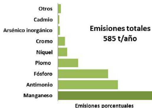
Figura 41. Emisiones de metales tóxico ZMVM, 2012
