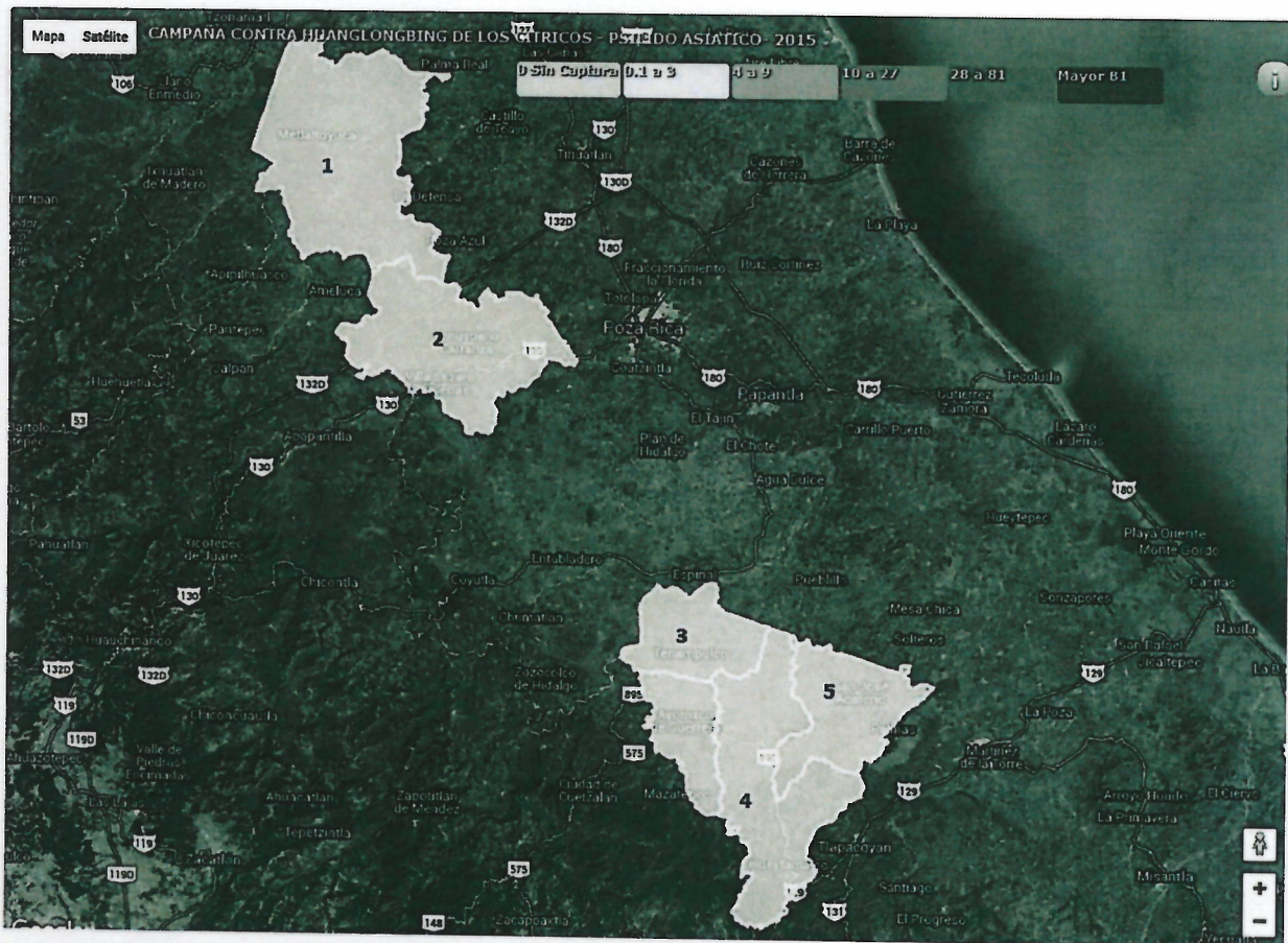
Figura 1. Mapa de la situación fitosanitaria que guarda la plaga en la Entidad (1.- Francisco Z. Mena, 2.- Venustiano Carranza, 3.- Tenampulco, 4.- Hueytamalco y 5.- San José Acateno. (fuente: http://www.sicafi.gob.mx:81/SICAFI/Admin/Reportes/bdc/Criterios/MapalInfestacion.aspx ).
