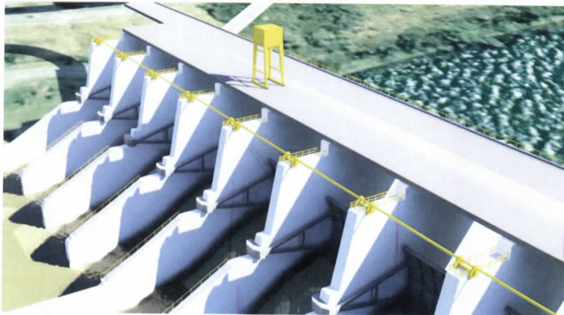
Figura 7.405.- Modelado y mapeado de presa
