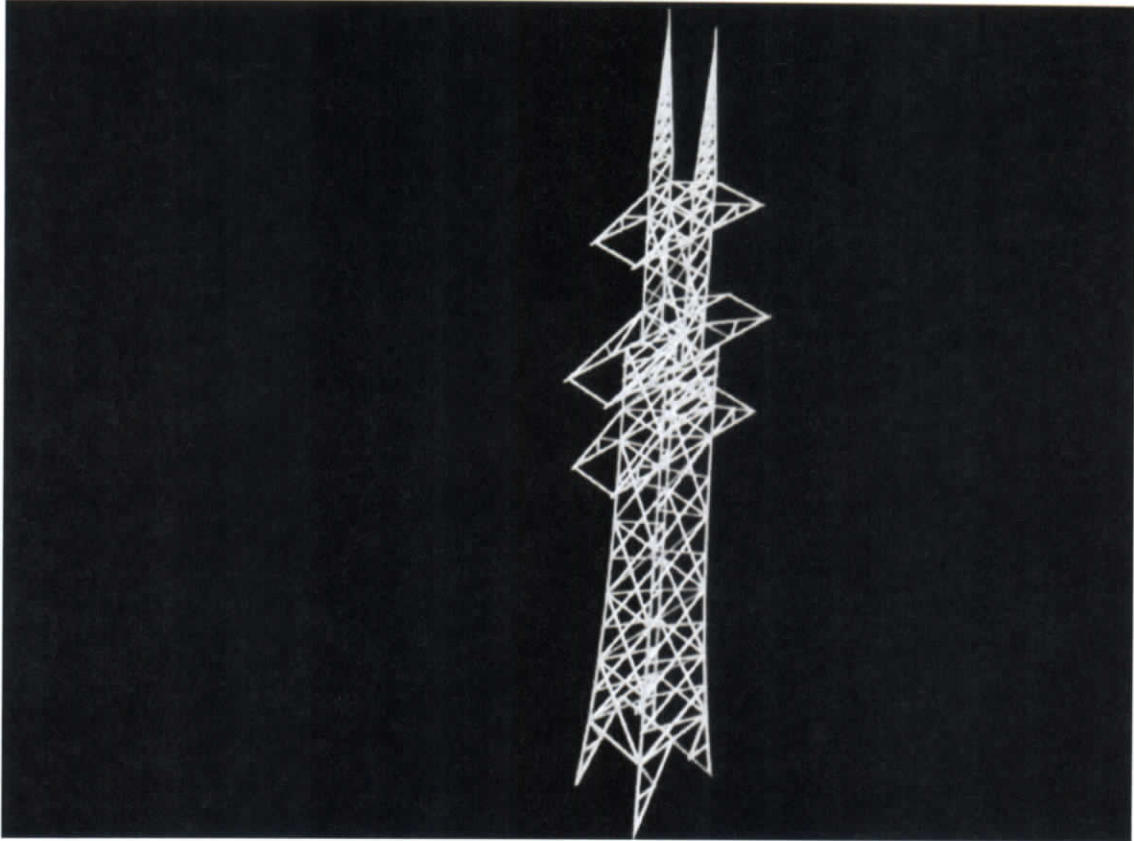
Figura 7.457.- Modelado de torres eléctricas
