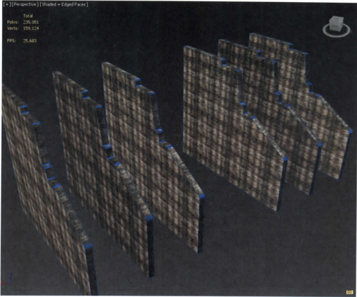
Figura 7.390.- Modelado y mapeado de presa
