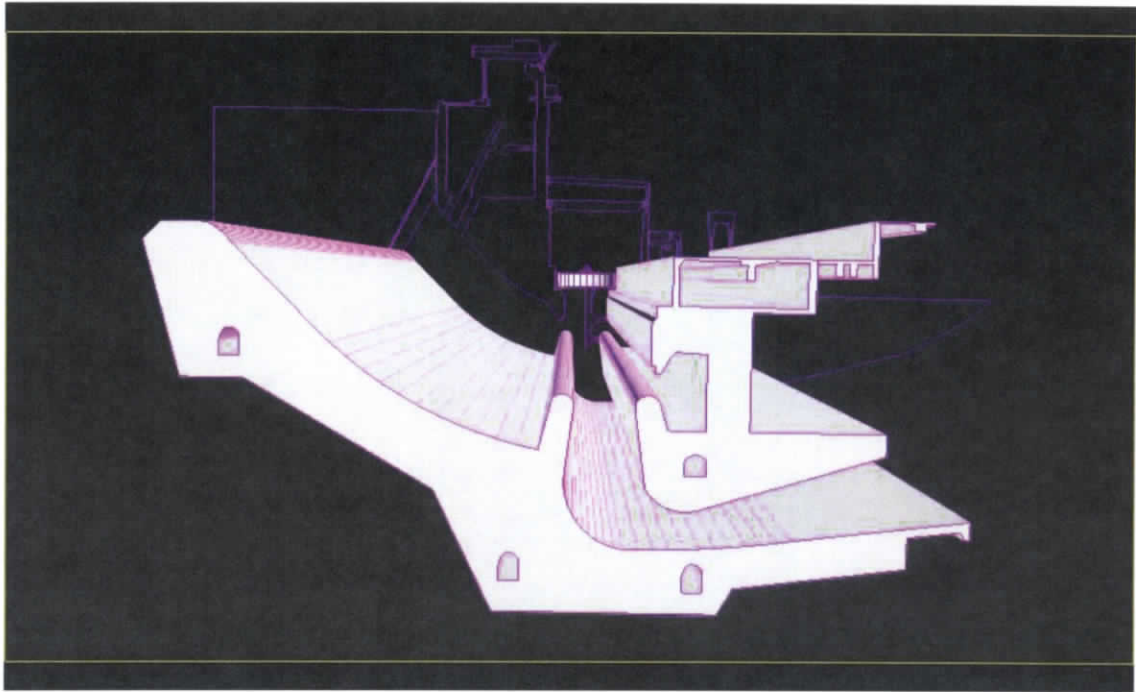
Figura 7.433.- Modelado de presa
