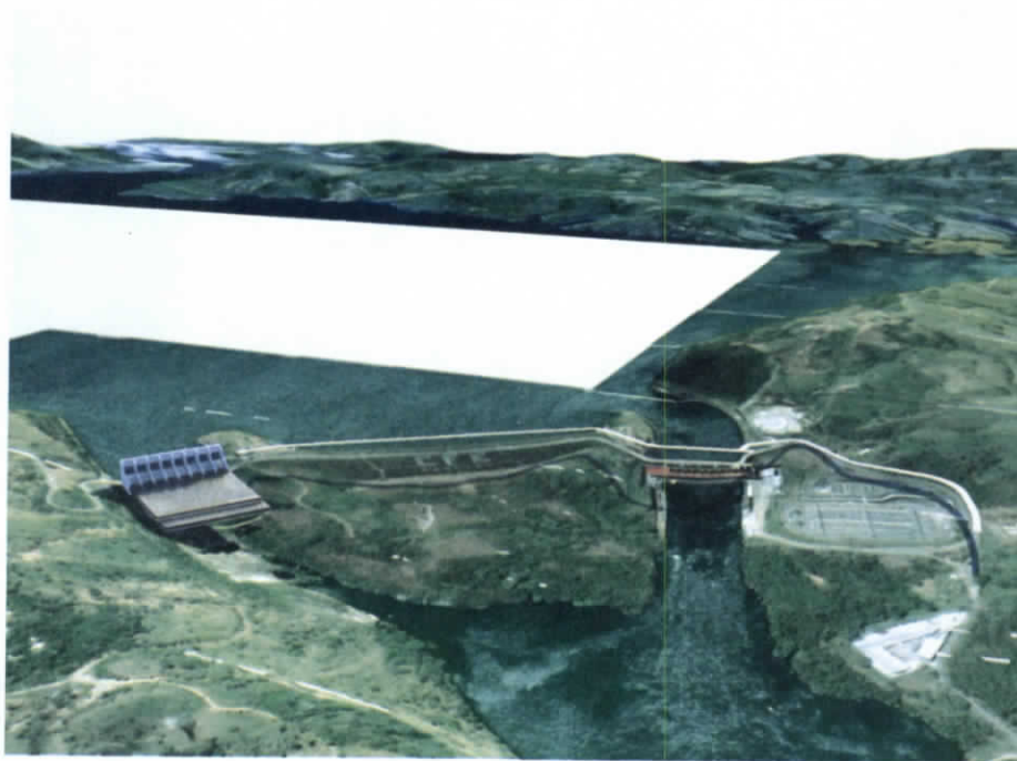
Figura 7.408.- Modelado y mapeado de presa y contexto
