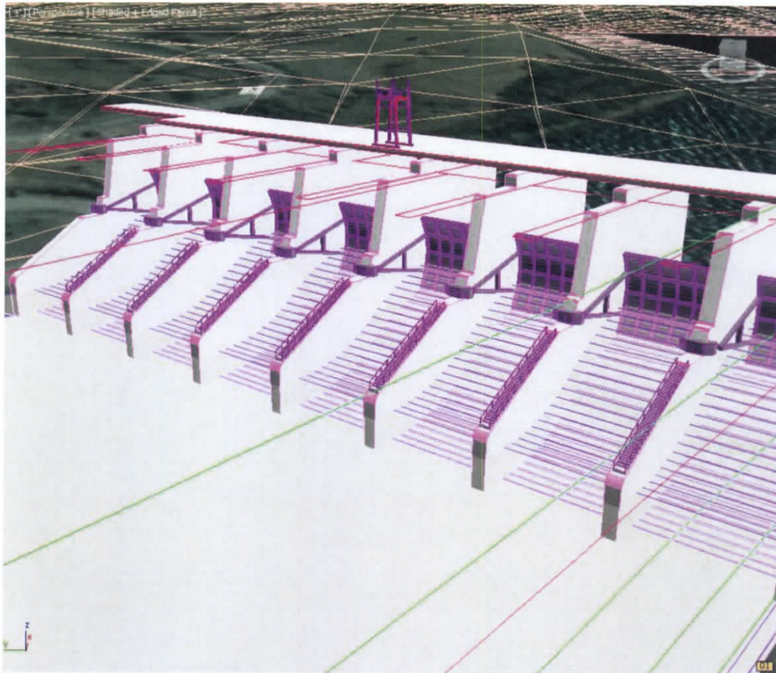
Figura 7.413.- Modelado y mapeado de presa y contexto
