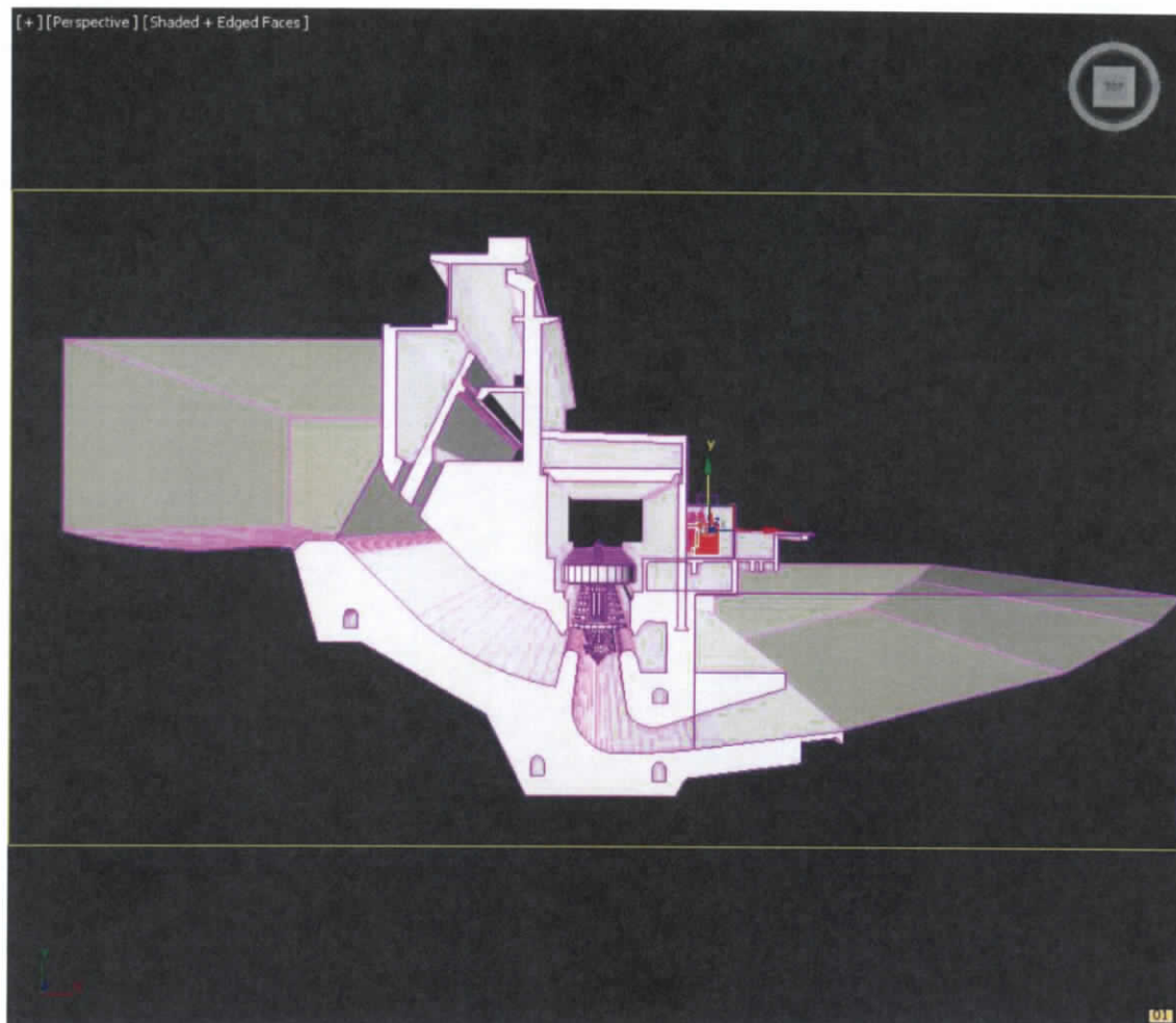
Figura 7.436.- Modelado de presa
