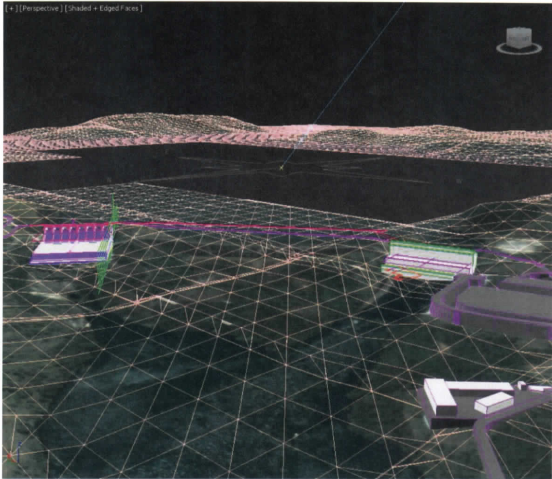
Figura 7.423.- Modelado y mapeado de presa y contexto
