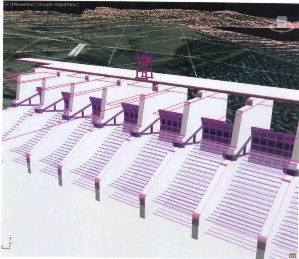
Figura 7.410.- Modelado de presa
