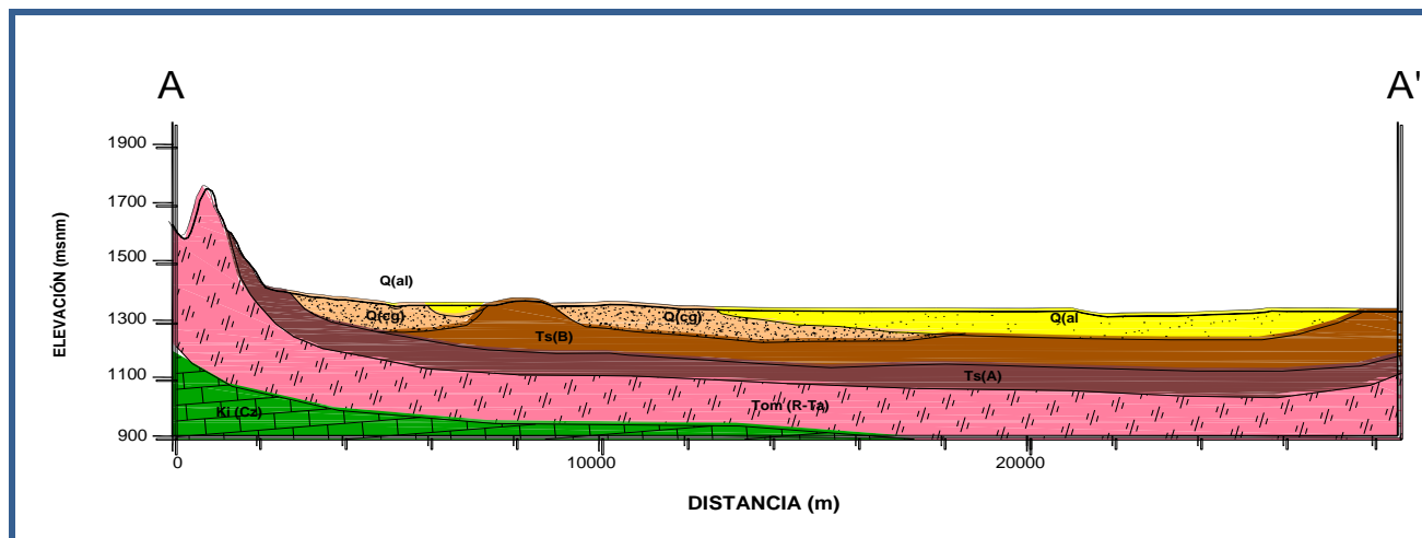
Figura 3. Sección geológica
