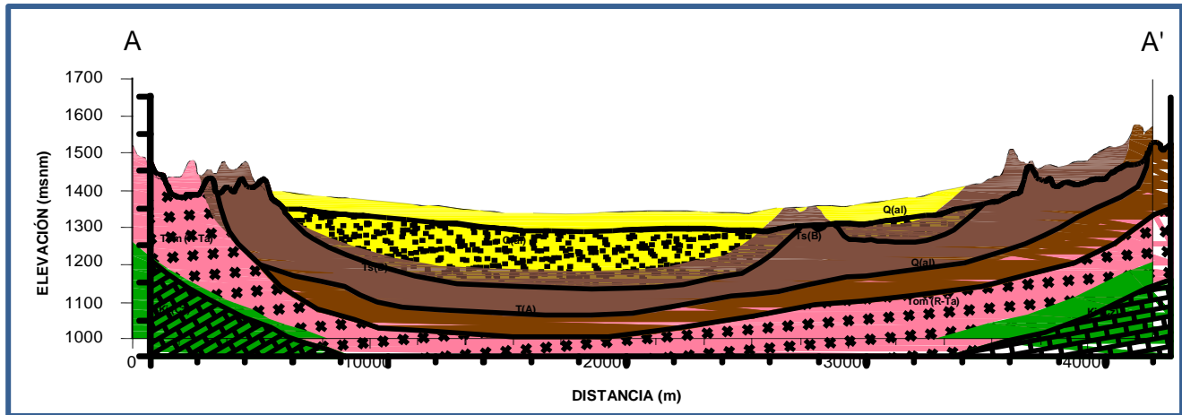
Figura 4. Sección Geológica
