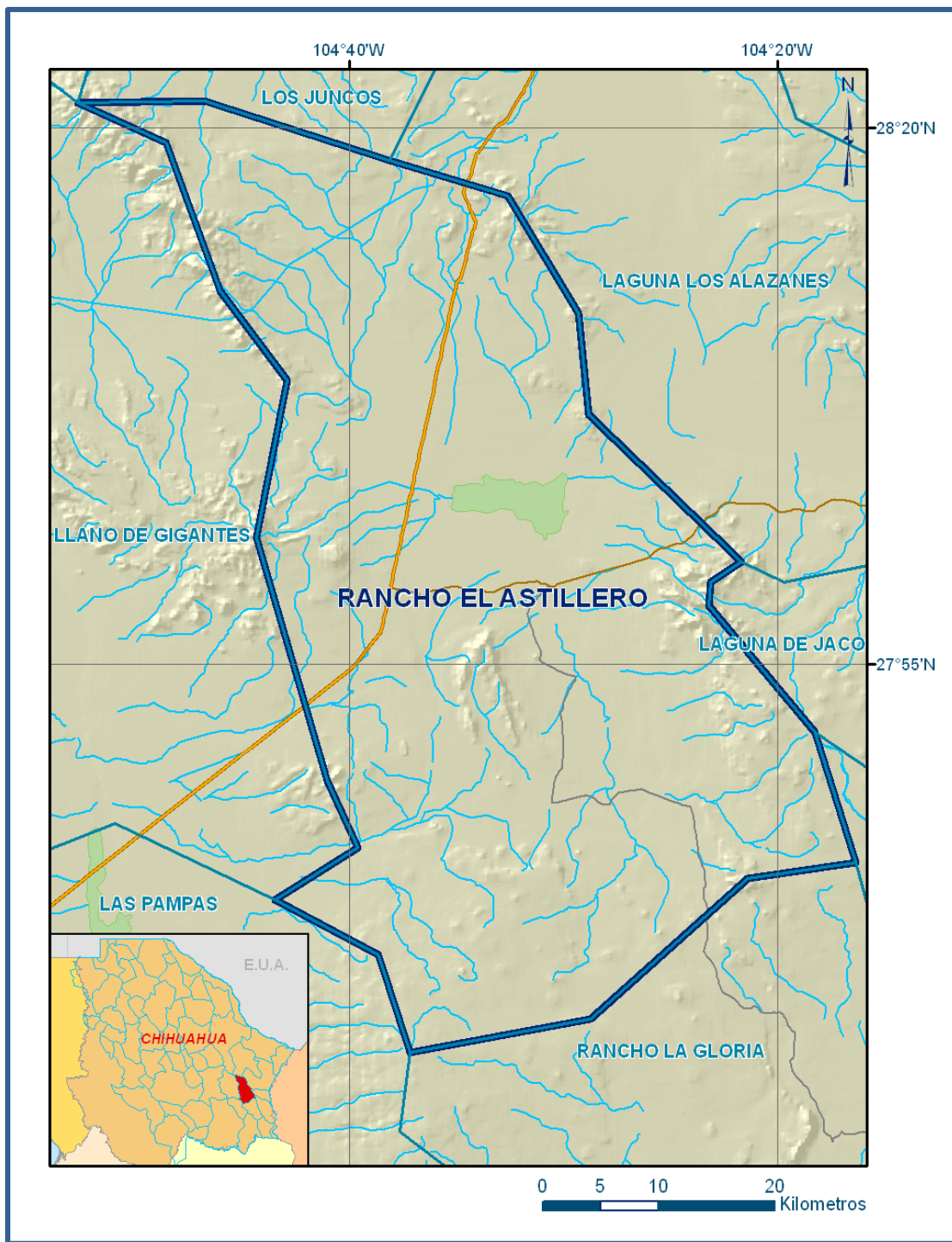
Figura 1. Localización del acuífero Rancho El Astillero.
