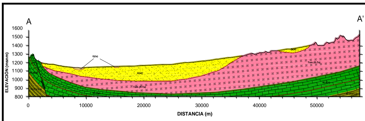
Figura 3. Sección geológica esquemática
