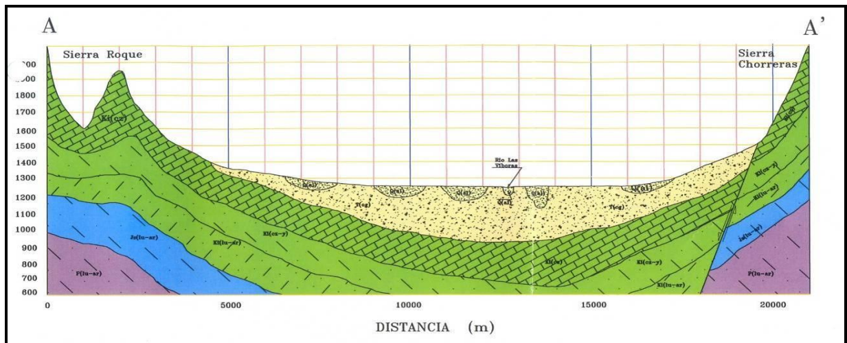
Figura 3. Sección Geológica A-A'
