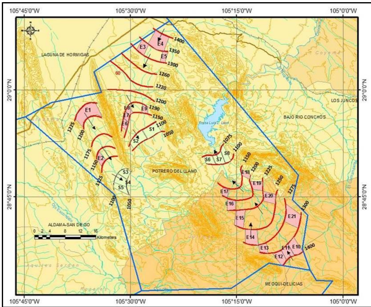
Figura 6. Elevación de nivel estático en msnm (2006)
