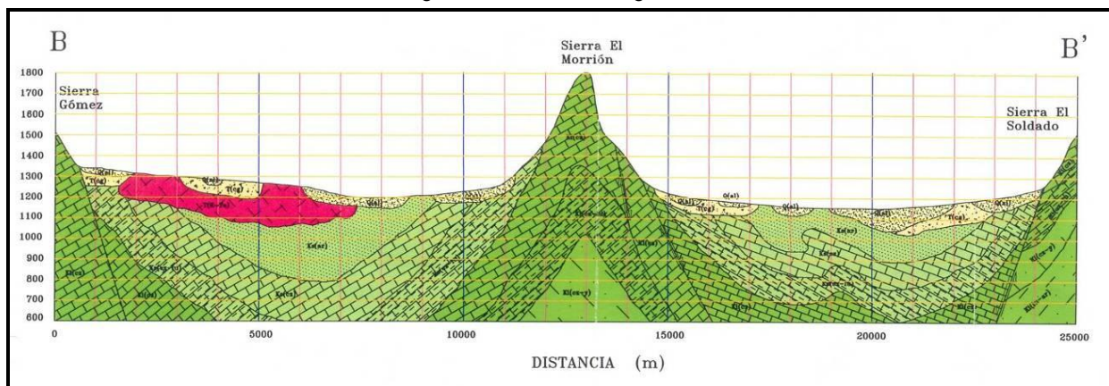
Figura 4. Sección Geológica B-B'
