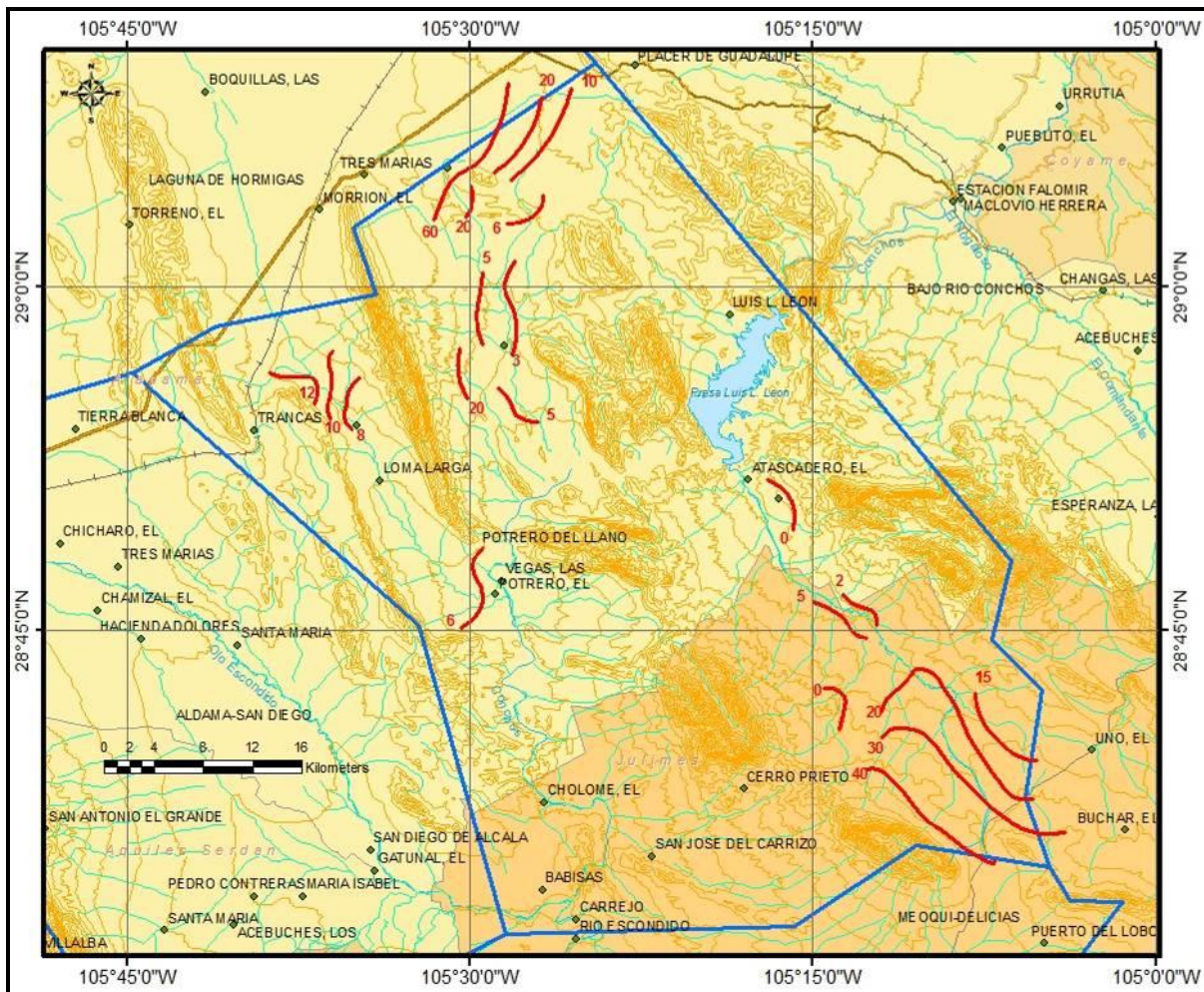
Figura 5. Profundidad al nivel estático en m (2006)
