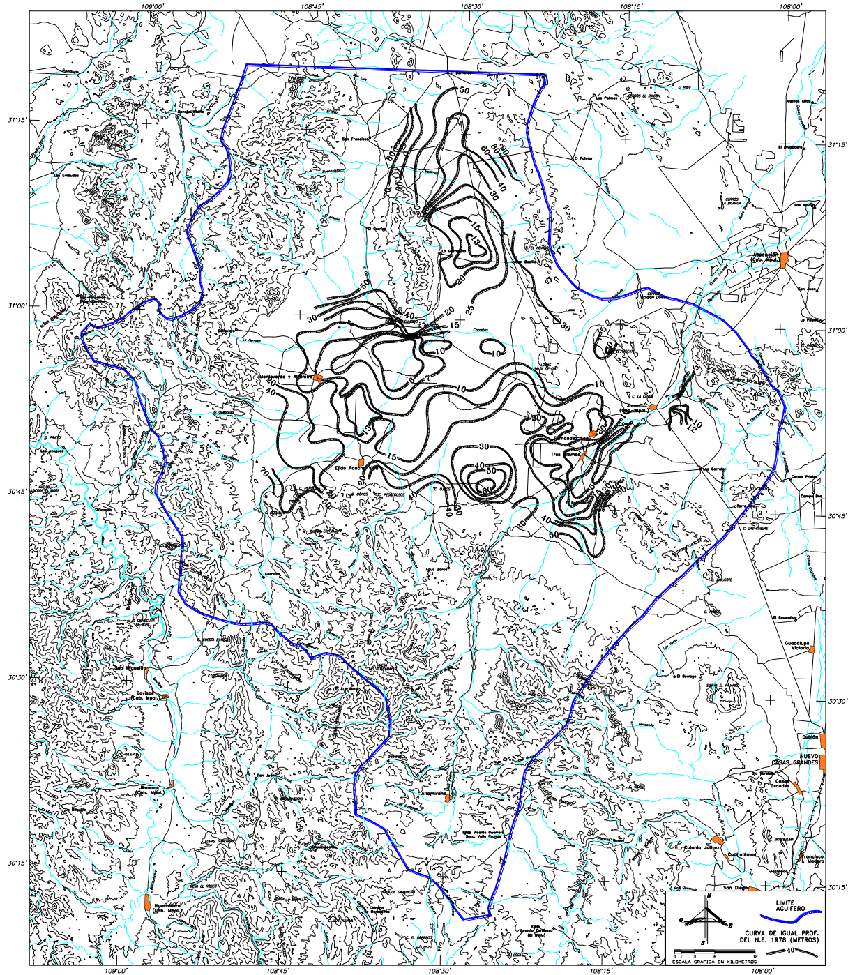
Figura 2 Profundidad del nivel estático. 1978
