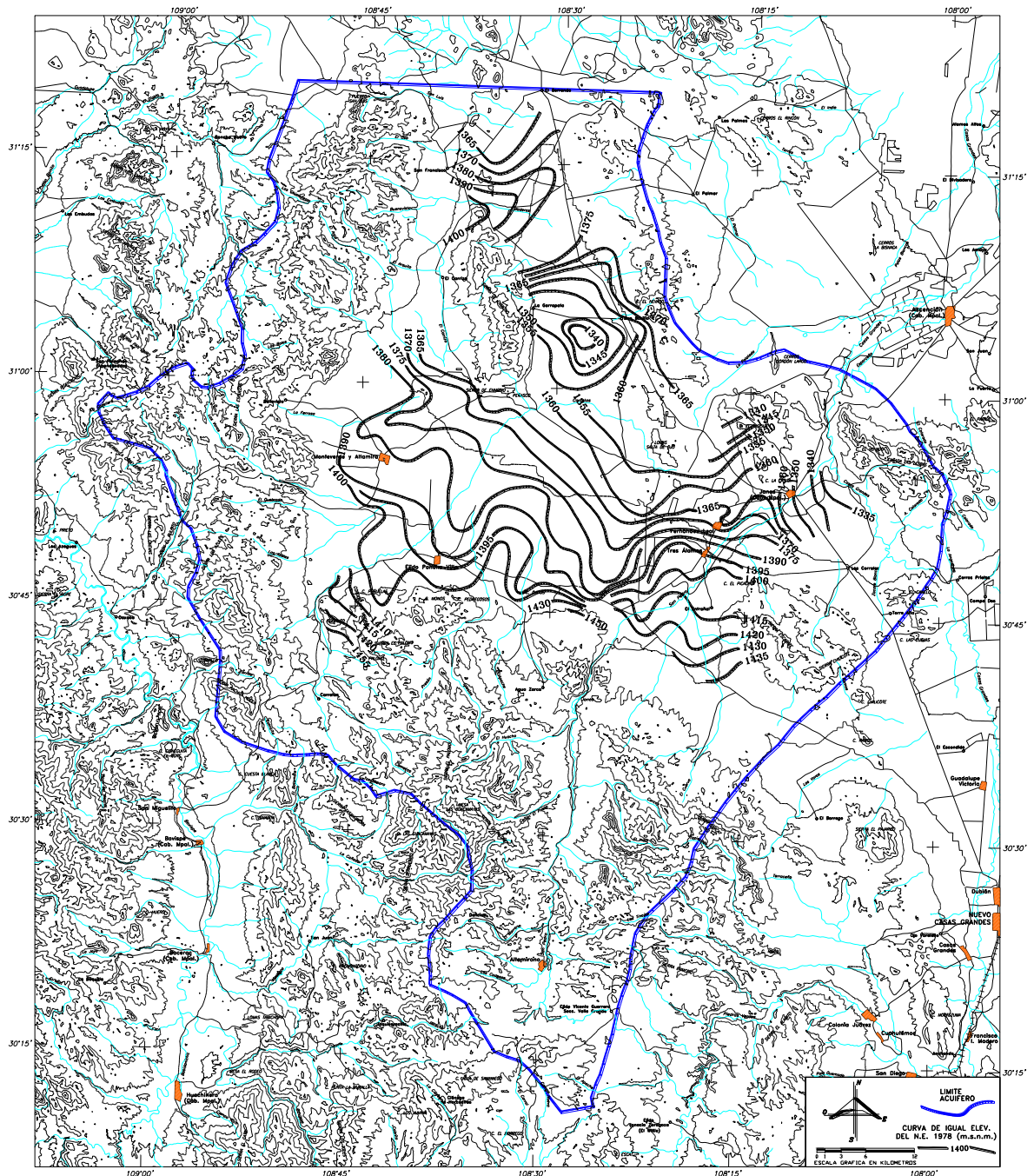
Figura 3 Elevación de los niveles estáticos. 1978
