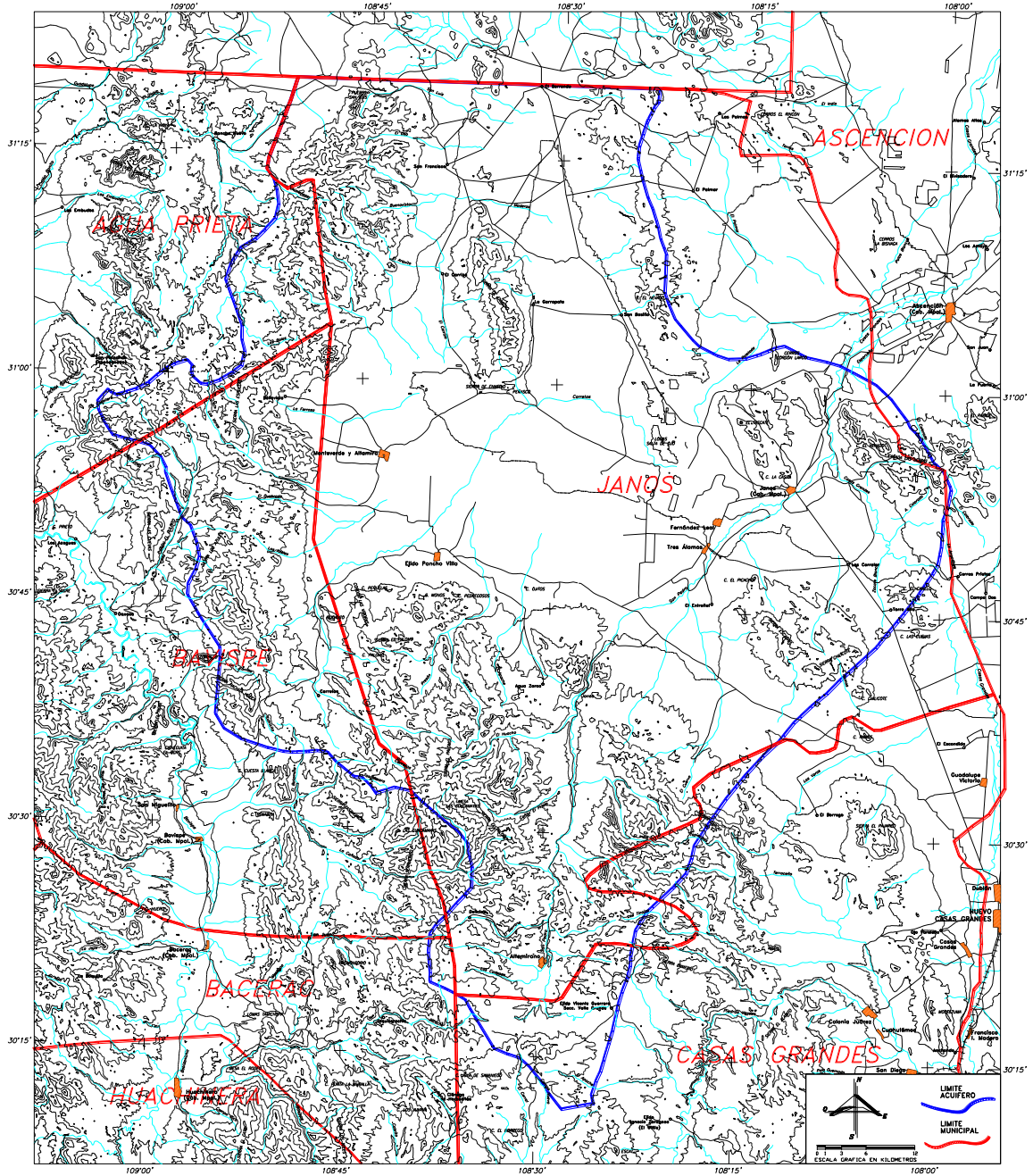
Figura 1 Zona del acuífero Janos, Chih.
