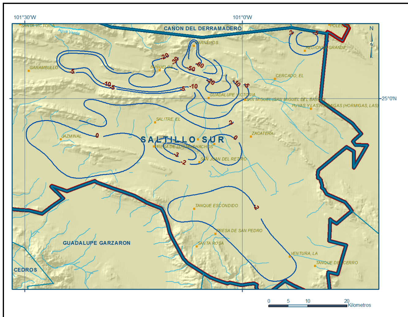
Figura 7. Evolución del nivel estático en m (1997 - 2010)
