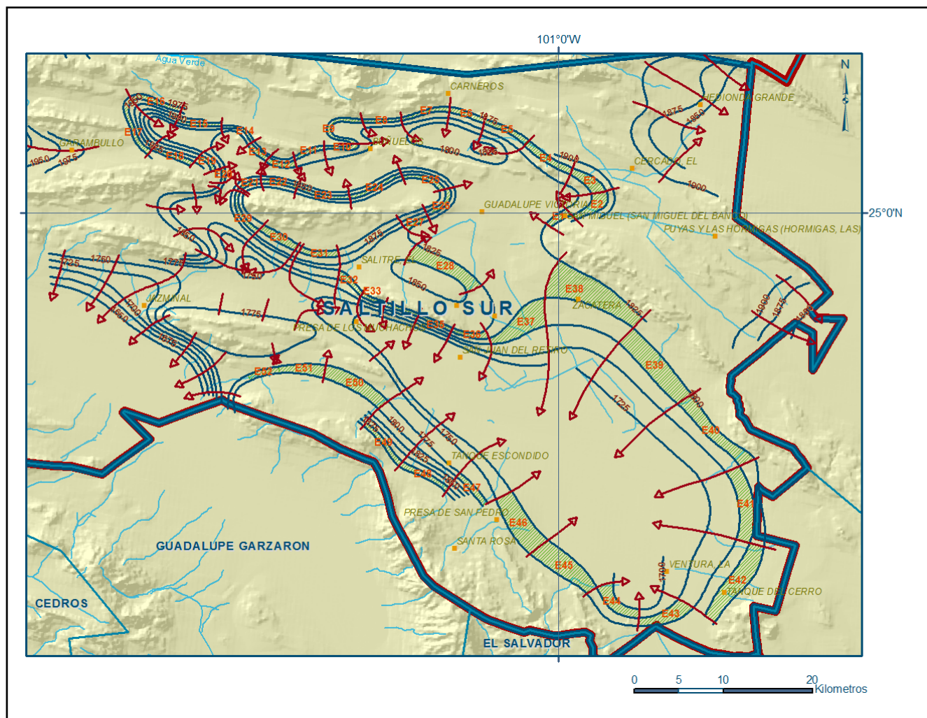
Figura 6. Elevación del nivel estático en msnm (2010)
