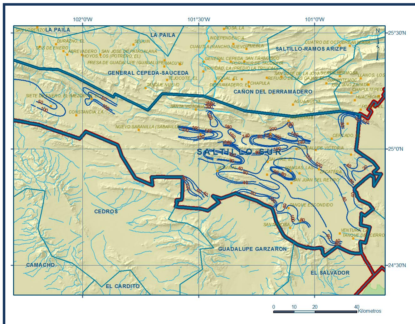
Figura 5. Profundidad al nivel estático en m (2010)
