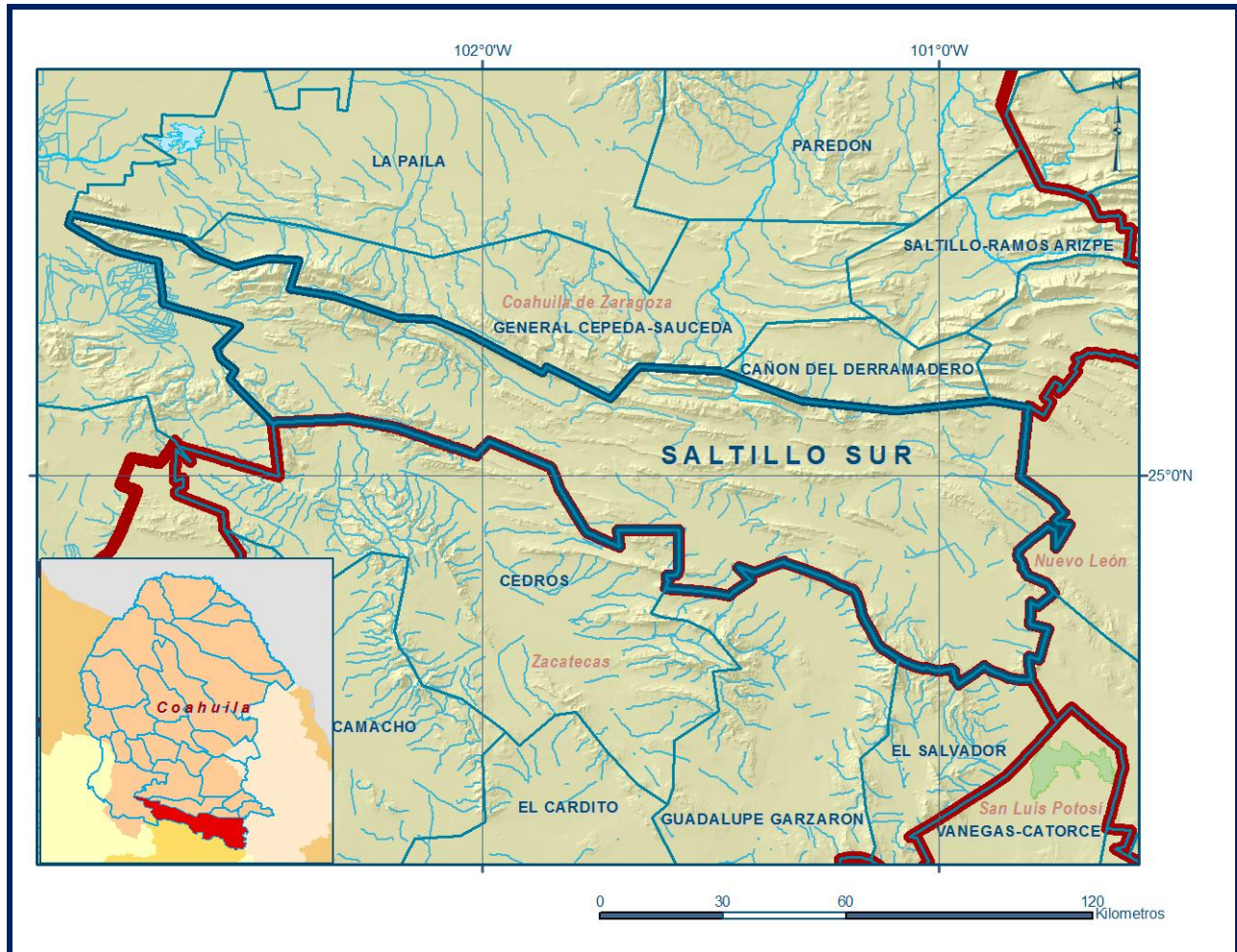
Figura 1. Localización del acuífero Saltillo Sur
