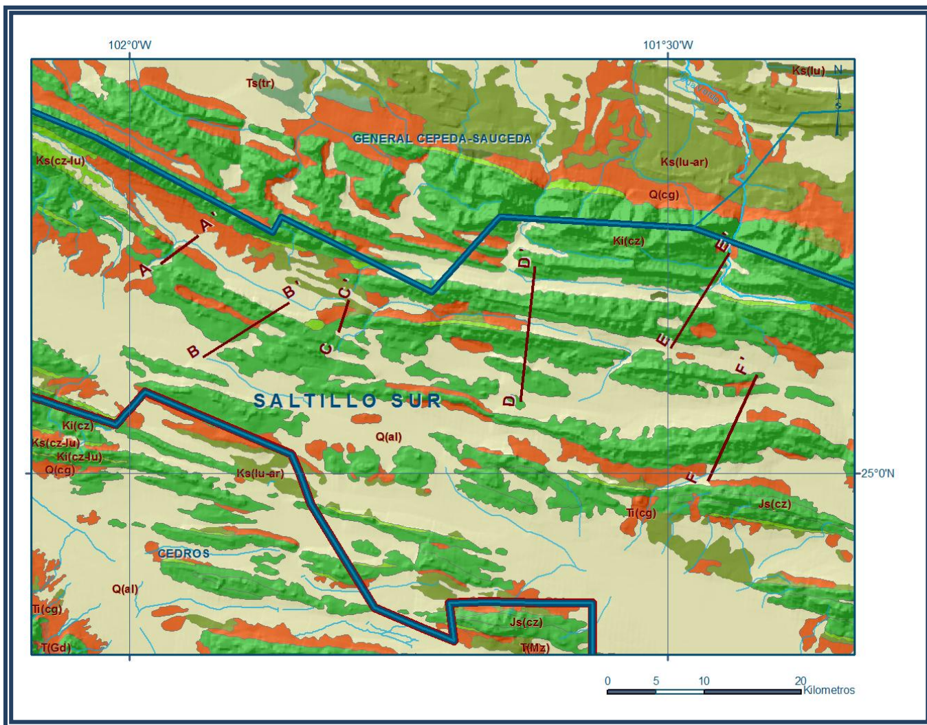
Figura 3. Localización de Secciones Geológicas
