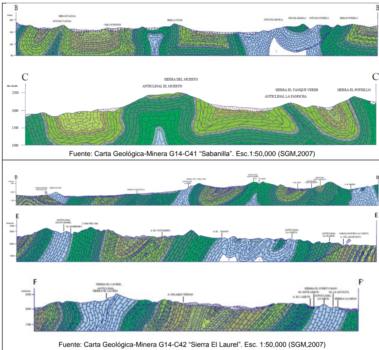
Figura 4. Secciones Geológicas Esquemáticas
